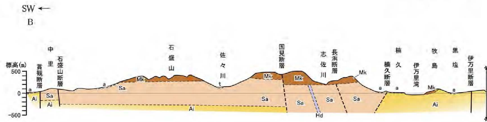
【B-B'断面図】
