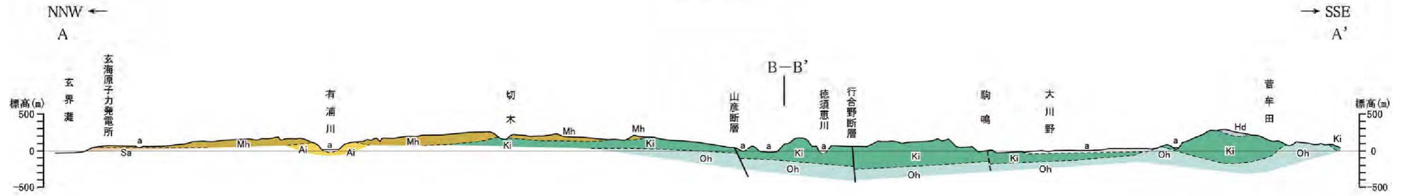
【A-A'断面図】
