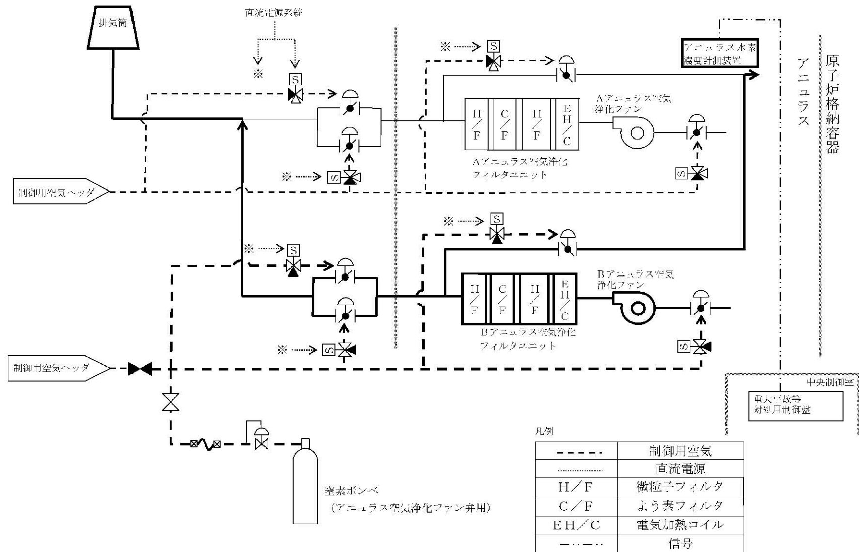
第1.6-71図 アネウラス空気浄化設備(重大事故等時) 概略系統図(2) (全交流動力電源又は直流電源が喪失した場合)
