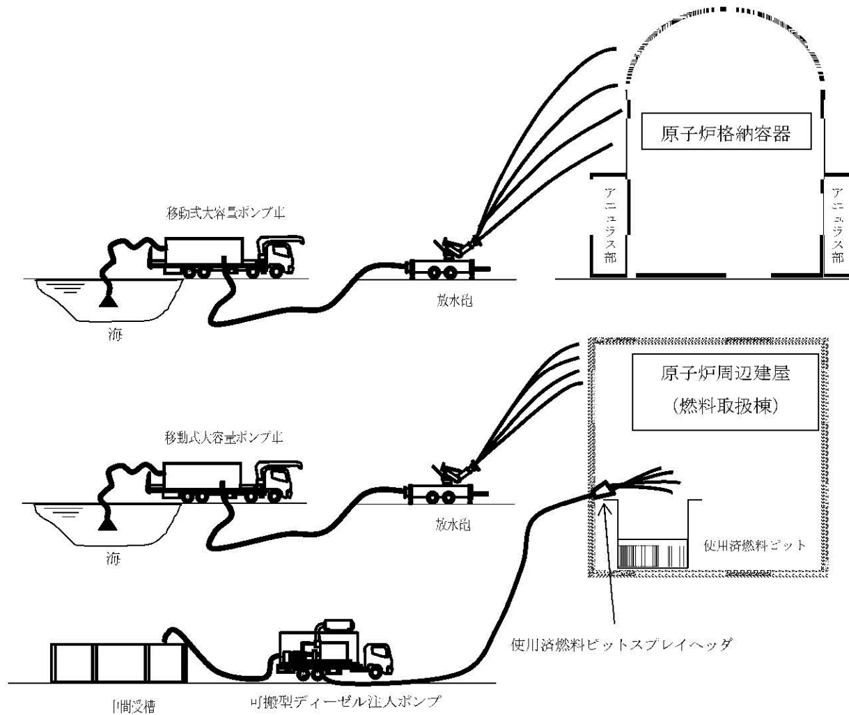
第1.6-81図 発電所外への放射性物質の拡散を抑制するための設備 概略系統図(1) (移動式大容量ポンプ車及び放水砲による大気への拡散抑制、可搬型ディーゼル注入ポンプを用いた使用済燃料ピットスプレイヘッダによる使用済燃料ピットへのスプレイ)
