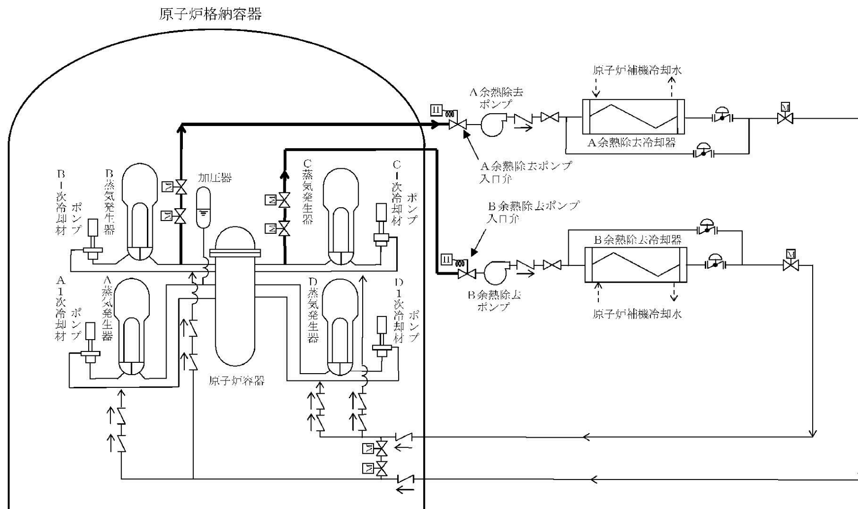
第1.6-10図 原子炉冷却材圧力バウンダリを減圧するための設備 概略系統図(5) (1次冷却材の漏えい量抑制)
