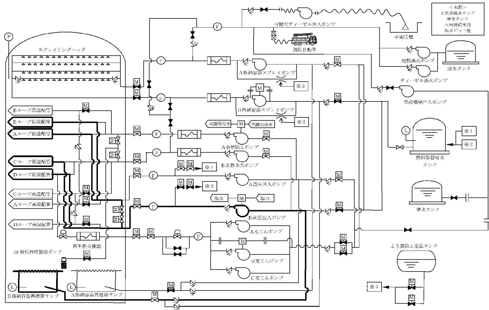
第1.6-35図 重大事故等の収束に必要となる水の供給設備 概略系統図 (5) (高圧注入ポンプによる高圧再循環)
