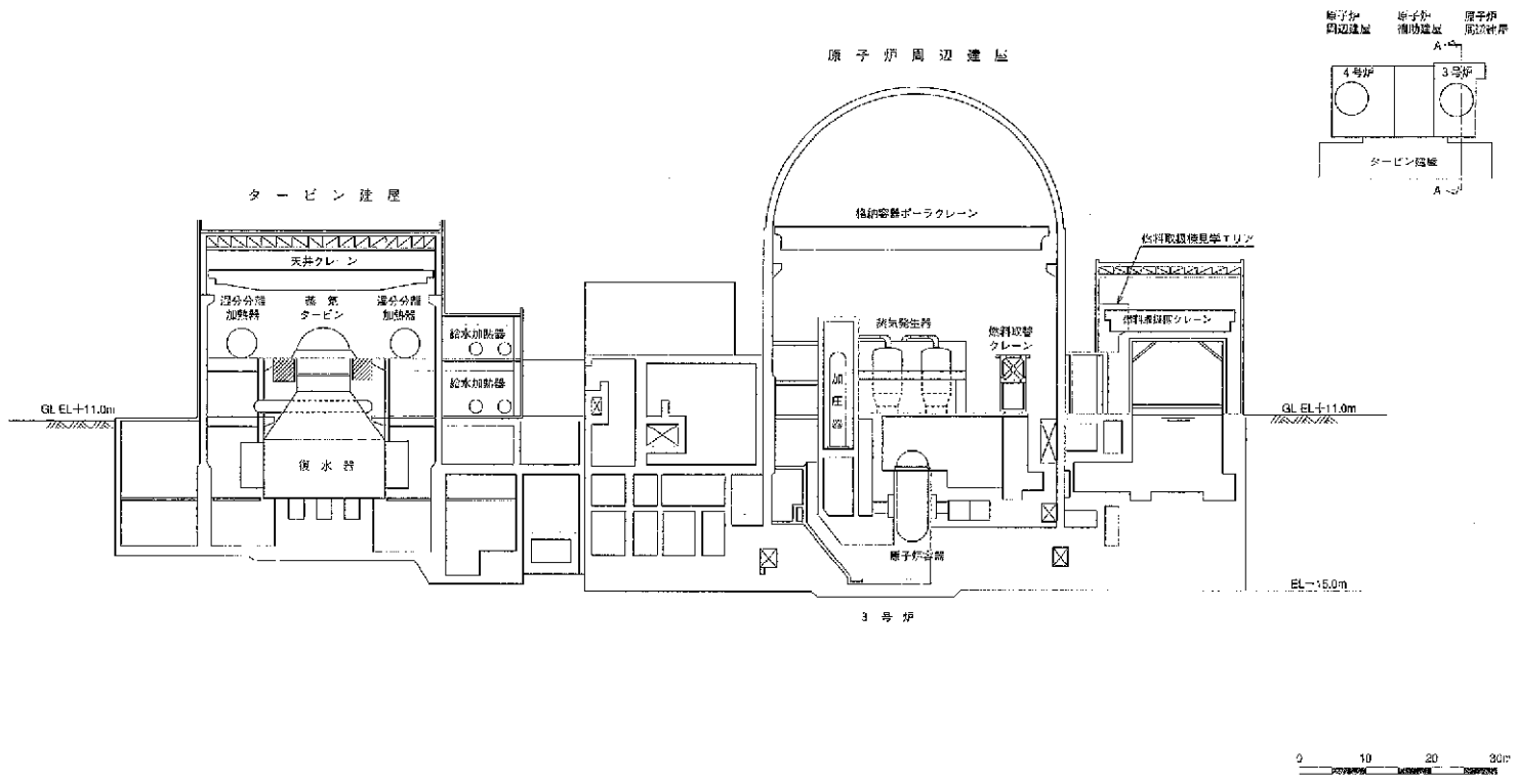
第1.9-33図 主要建屋断面図(A-A断面)
