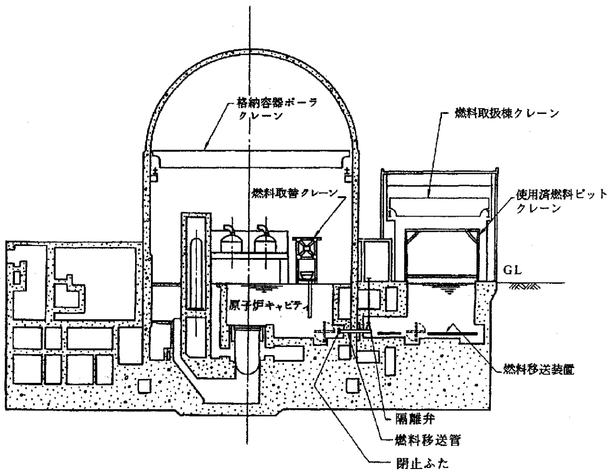
第1.9-2図 燃料取扱設備説明図(2)
