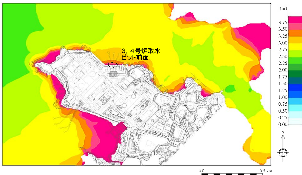
第1.2-10図(1) 基準津波の最高水位分布(朔望平均満潮位を考慮)
