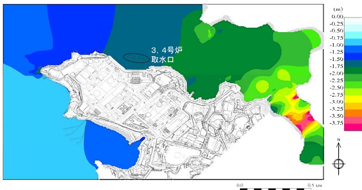
第1.2-9図(2) 基準津波の最大水位下降量分布 (初期潮位:T.P.±0.00m)
