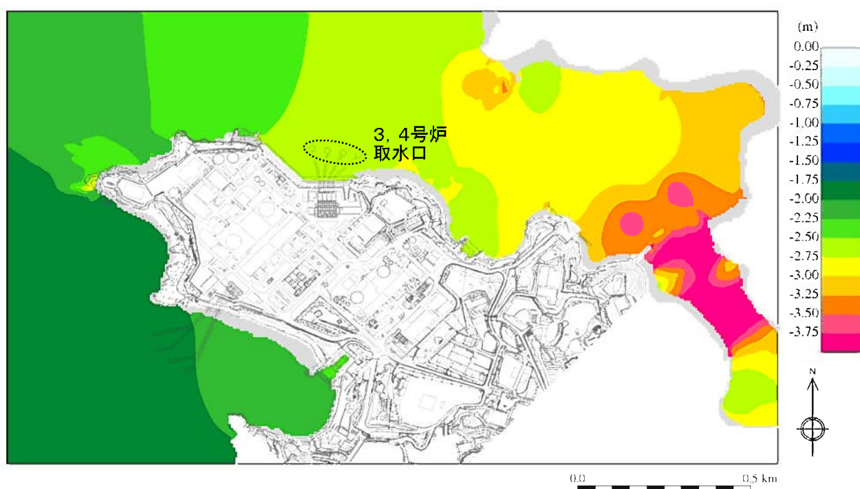
第1.2-10図(2) 基準津波の最低水位分布(朔望平均干潮位を考慮)
