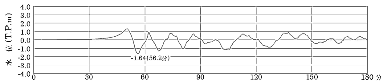
西山断層帯
