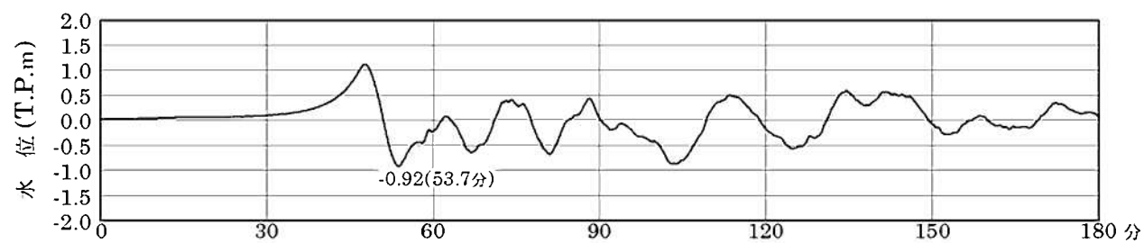
西山断層帯
