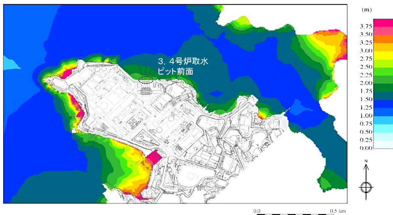
第1.2-9図(1) 基準津波の最大水位上昇量分布 (初期潮位:T.P.±0.00m)
