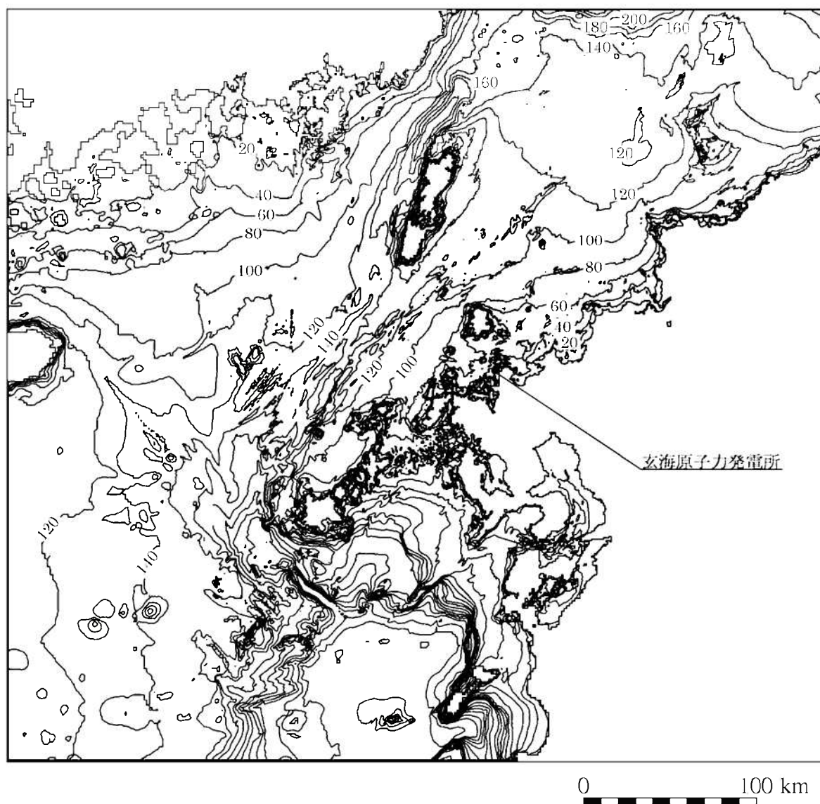
第1.2-5図(1) 海底地形(計算領域全体)
