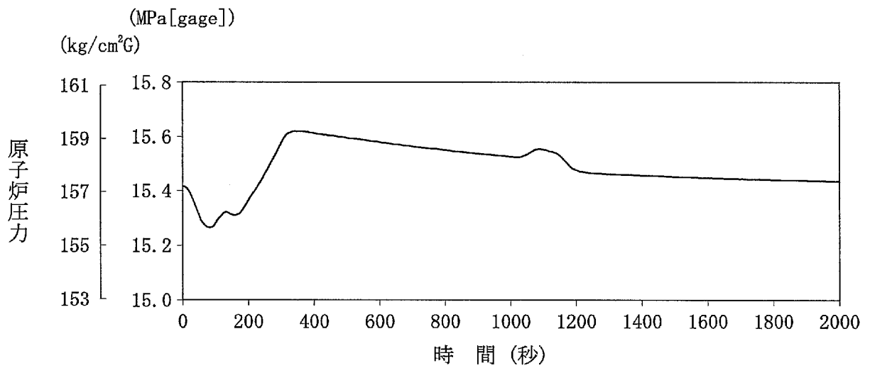
第1.4-28図 5%/minランプ状負荷増加の場合 (15%→100%) (3号機)
