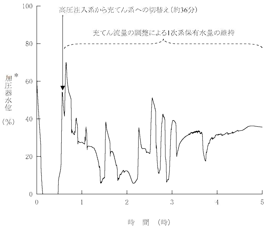
第1.15-342図 加圧器水位の推移 (蒸気発生器伝熱管破損時に破損側蒸気発生器の隔離に失敗する事故)
