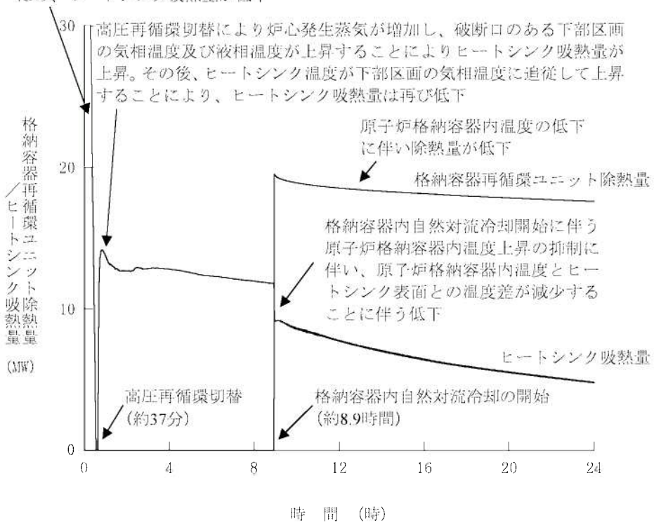
第1.15-221図 原子炉格納容器からの除熱量の推移
