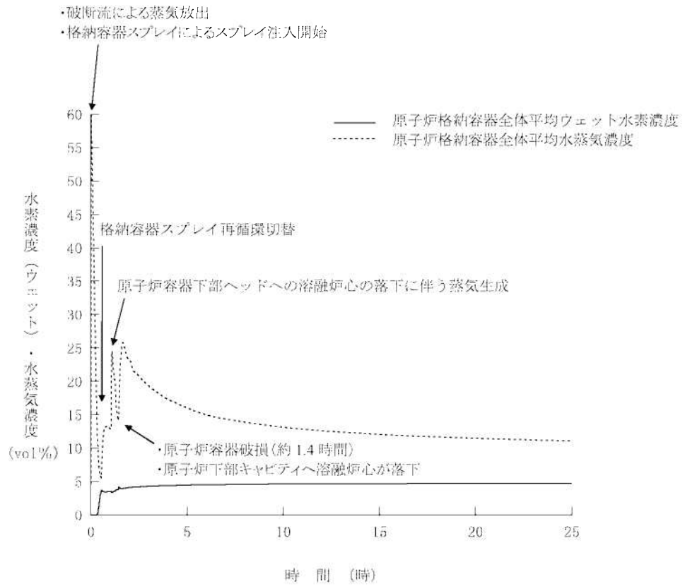
第1.15-431図 原子炉格納容器内の水素濃度(ウエット)・水蒸気濃度の推移 (MAAPコード)
