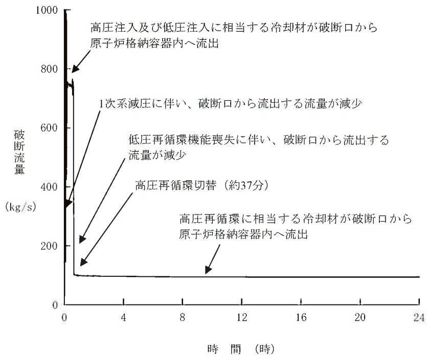
第1.15-212図 破断流量の推移
