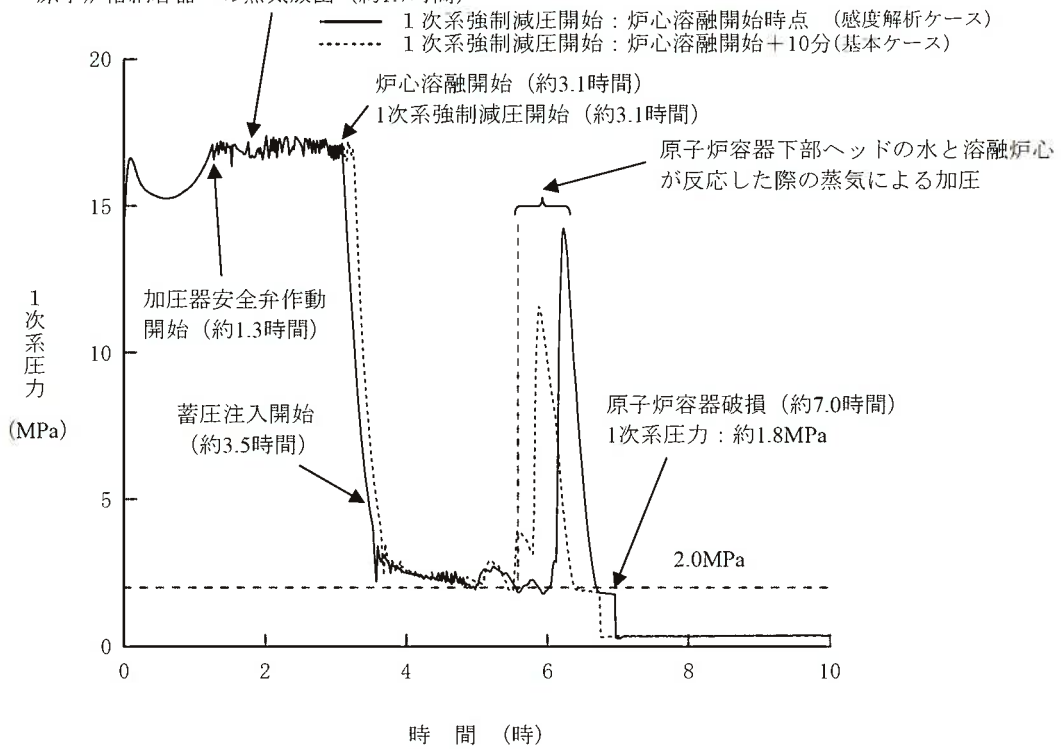
第1.15-425図 1次系圧力の推移 (加圧器逃がし弁開操作開始が早くなる場合)
