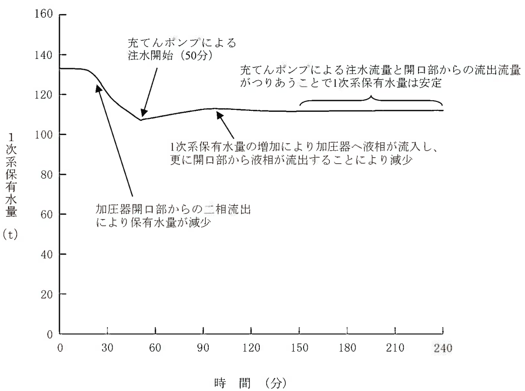
第1.15-353図 1次系保有水量の推移
