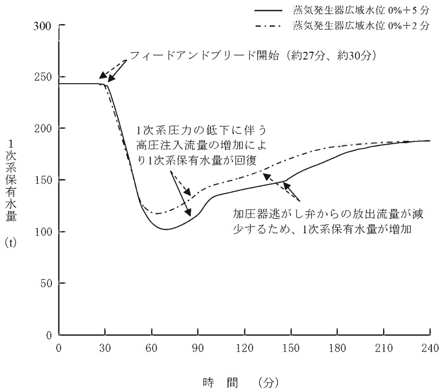
第1.15-160図 1次系保有水量の推移(開始が早くなる場合)
