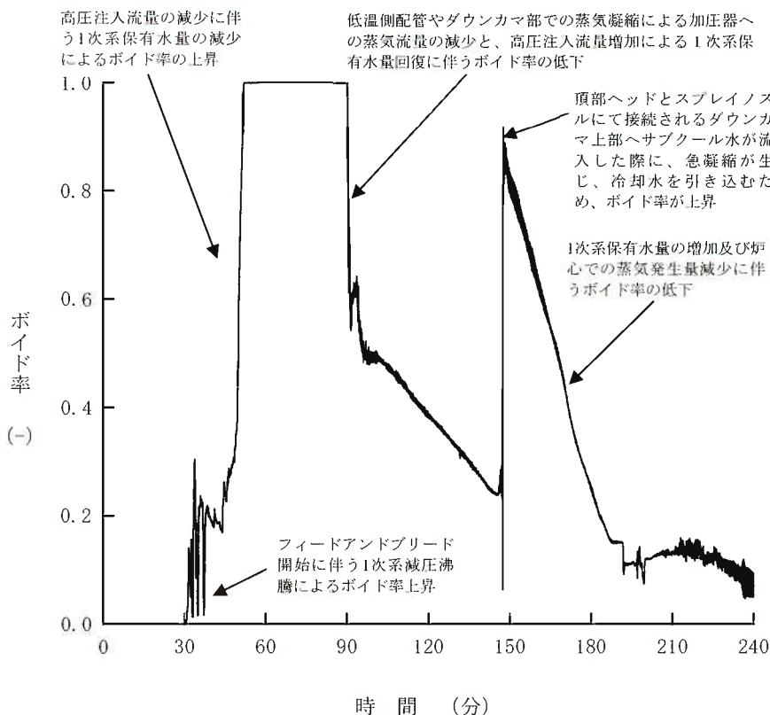
第1.15-143図 高温側配管・加圧器サージライン接続部ボイド率の推移
