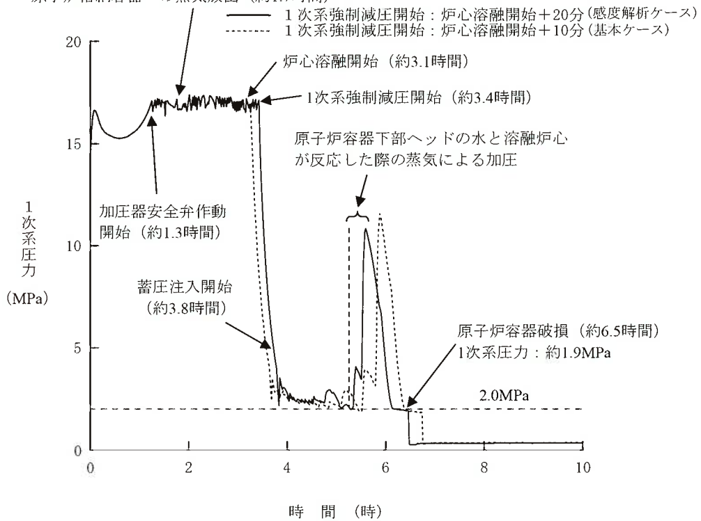
第1.15-426図 1次系圧力の推移 (加圧器逃がし弁開操作開始が遅くなる場合)
