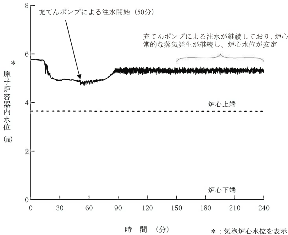
第1.15-352図 原子炉容器内水位の推移
