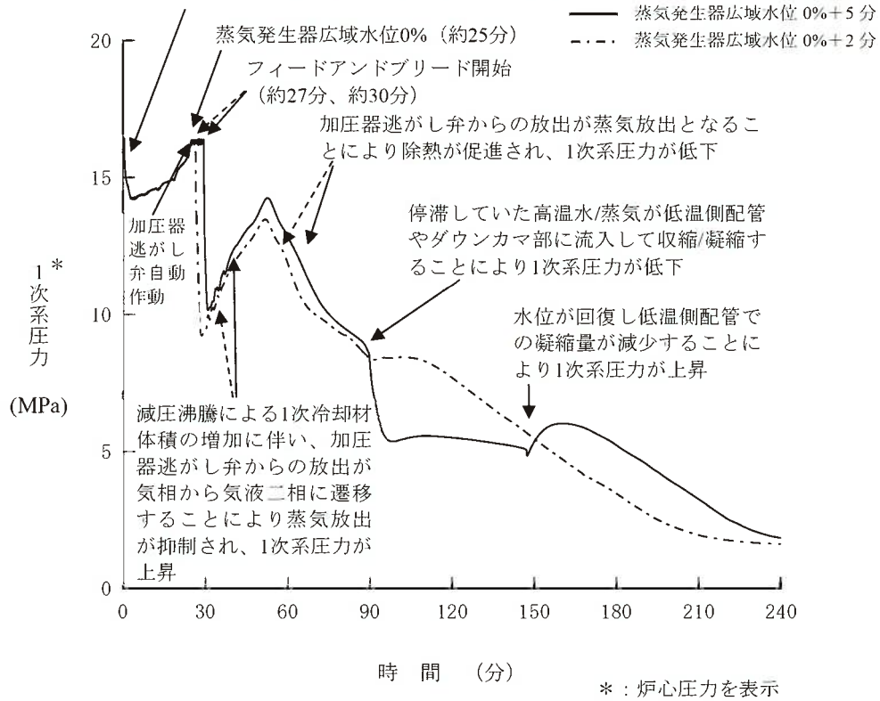
第1.15-157図 1次系圧力の推移(開始が早くなる場合)
