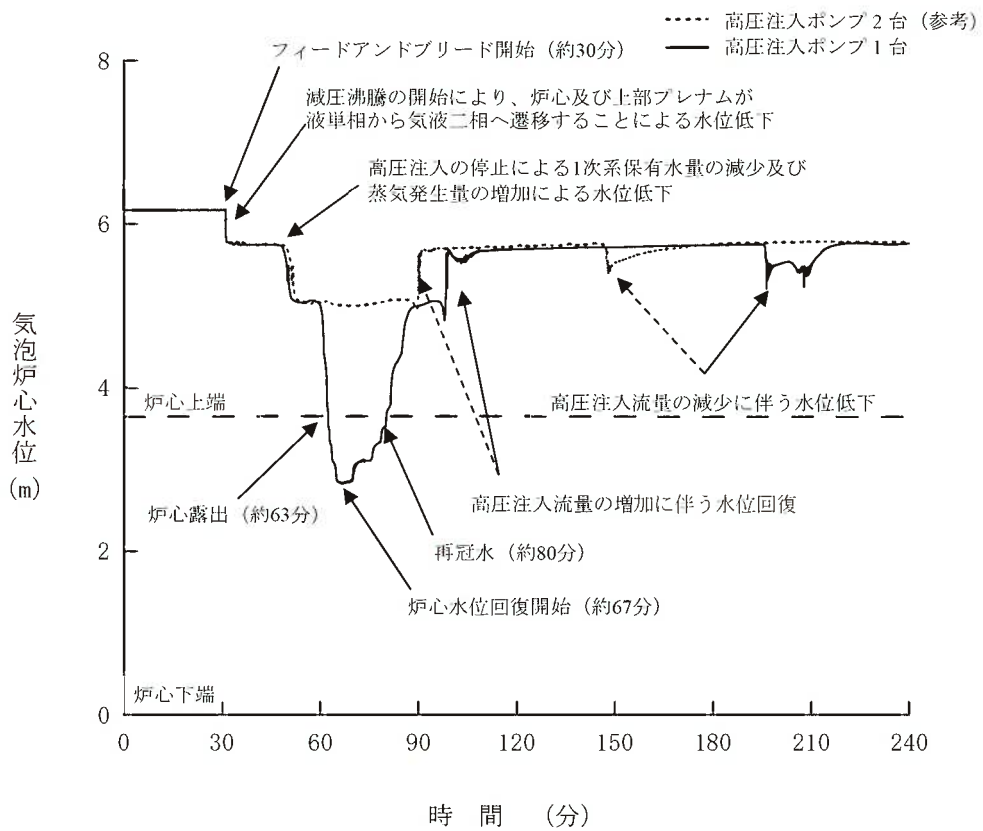
第1.15-155図 気泡炉心水位の推移(高圧注入ポンプ1台の場合)
