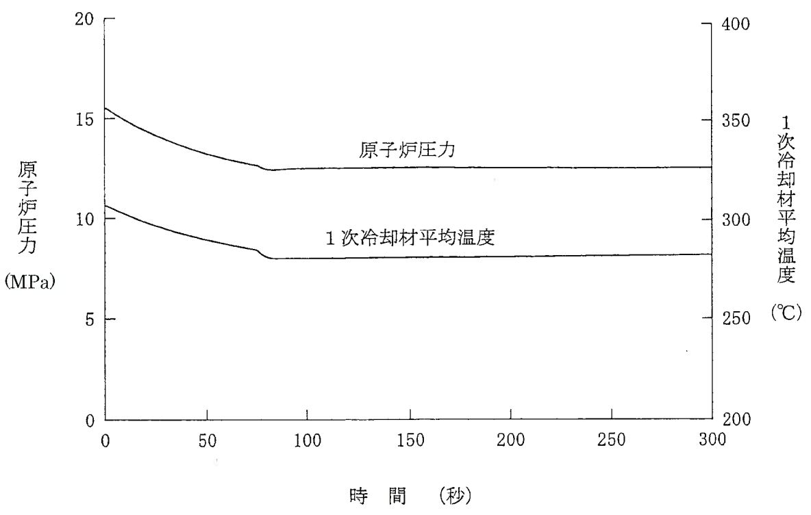
第1.15-99図 制御棒の落下—制御棒クラスタ手動制御運転
