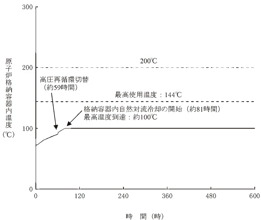
第1.15-189図 原子炉格納容器内温度の長期間の推移 (RCPシールLOCAが発生する場合)
