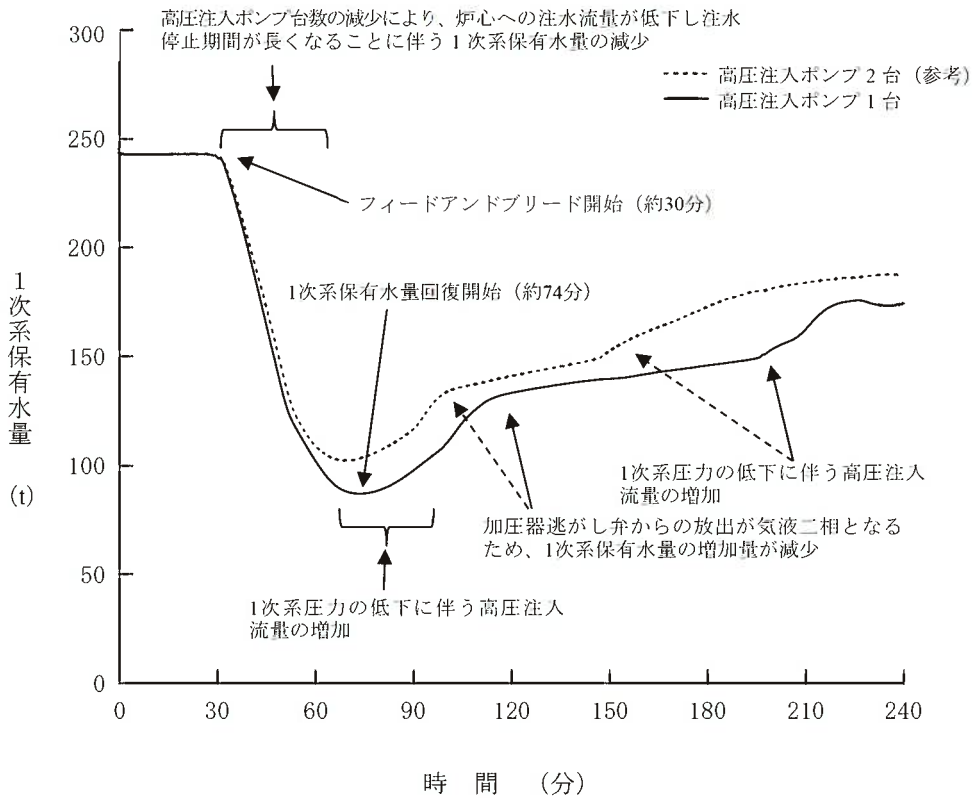
第1.15-154図 1次系保有水量の推移(高圧注入ポンプ1台の場合)
