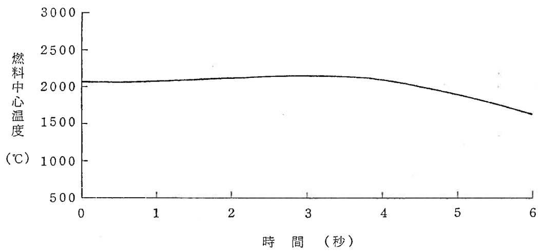
第1.15-94図 出力運転中の制御棒の異常な引抜き —速い引抜きの場合(2)
