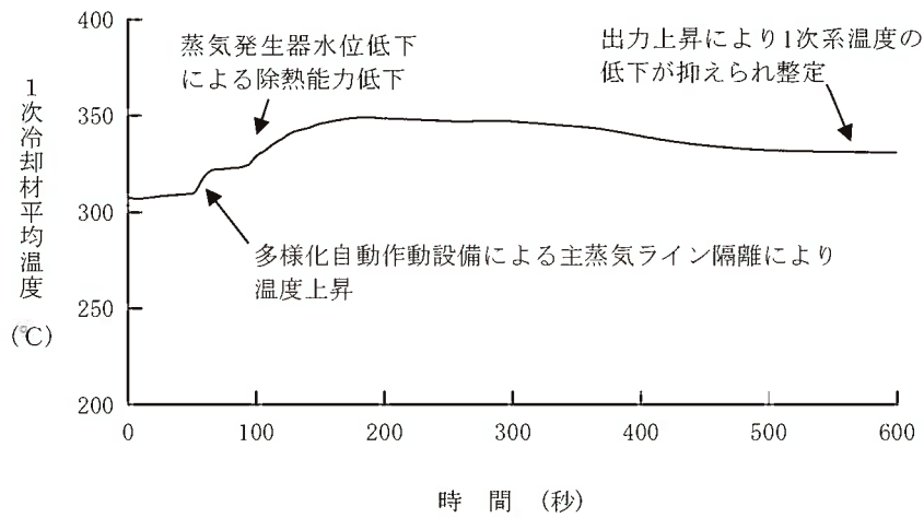
第1.15-228図 1次冷却材平均温度の推移 (主給水流量喪失時に原子炉トリップ機能が喪失する事故)
