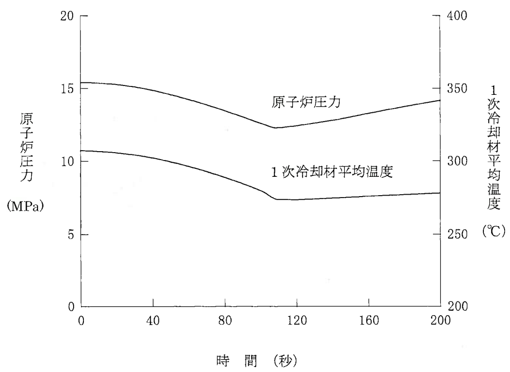
第1.15-111図 出力運転中の非常用炉心冷却系の誤起動
