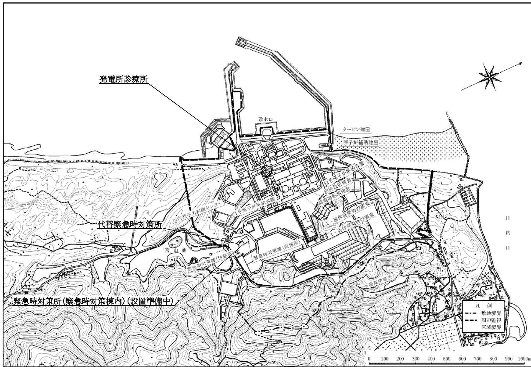
第 1.19-12 図 発電所内の緊急時対策所及び応急処置施設
