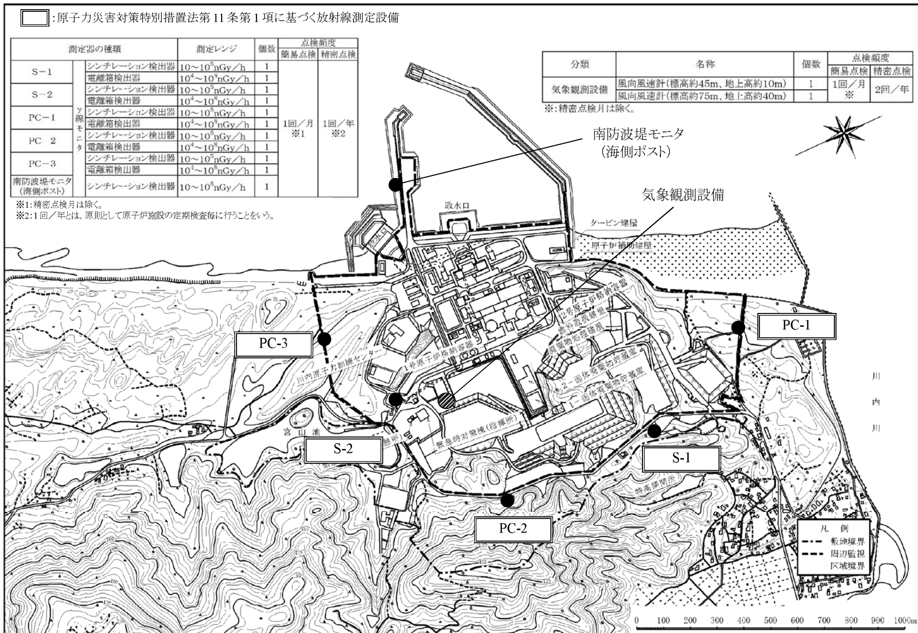
第 1.19-10 図 発電所敷地境界付近の放射線測定設備等
