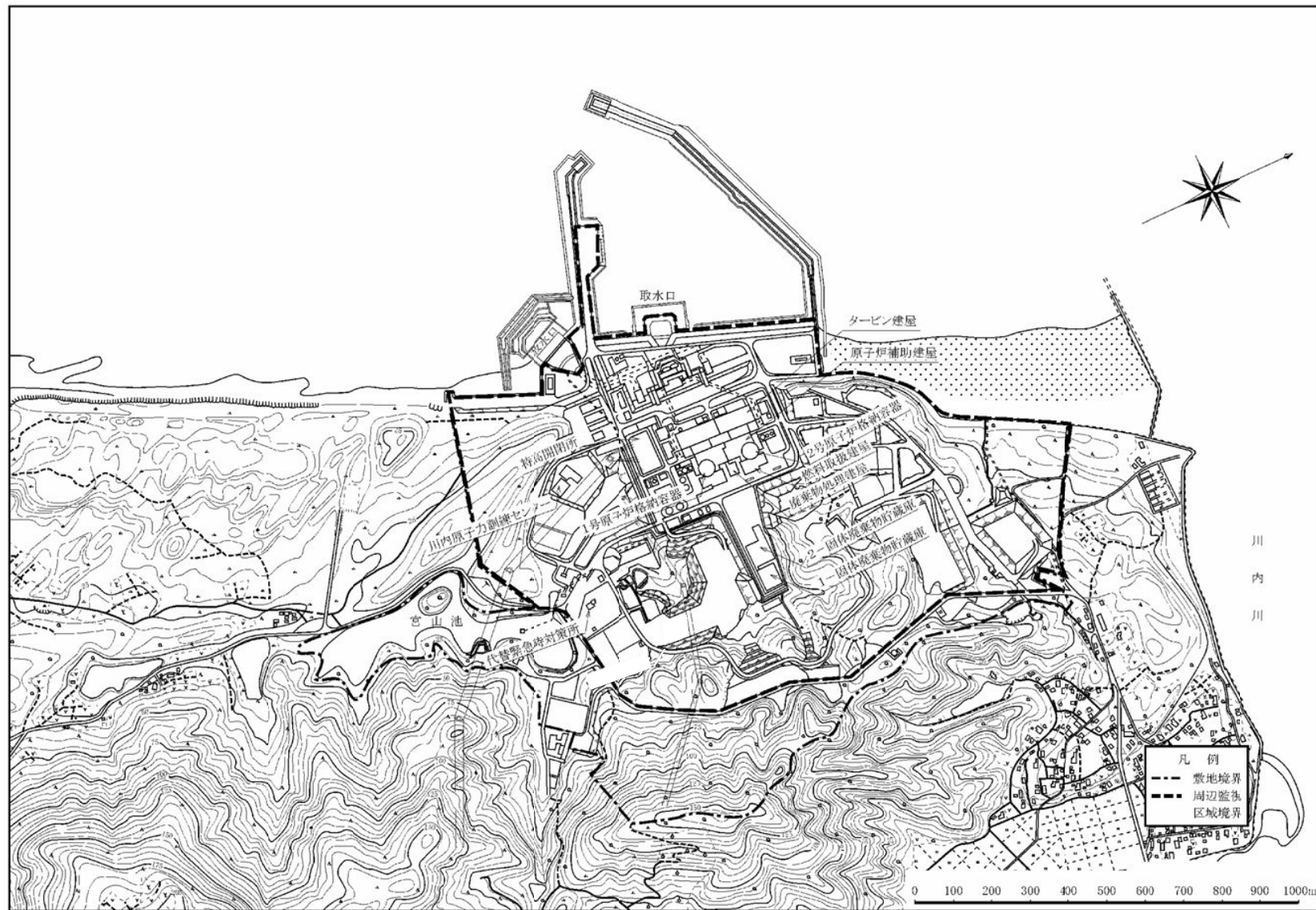
第1.1-1図 発電所敷地概況図
