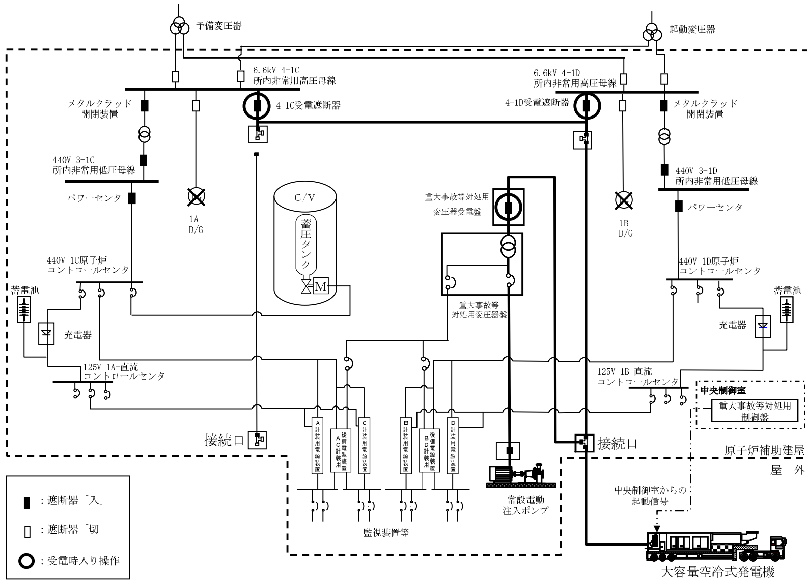
第1.8-2図 電源設備系統概要図(1)
