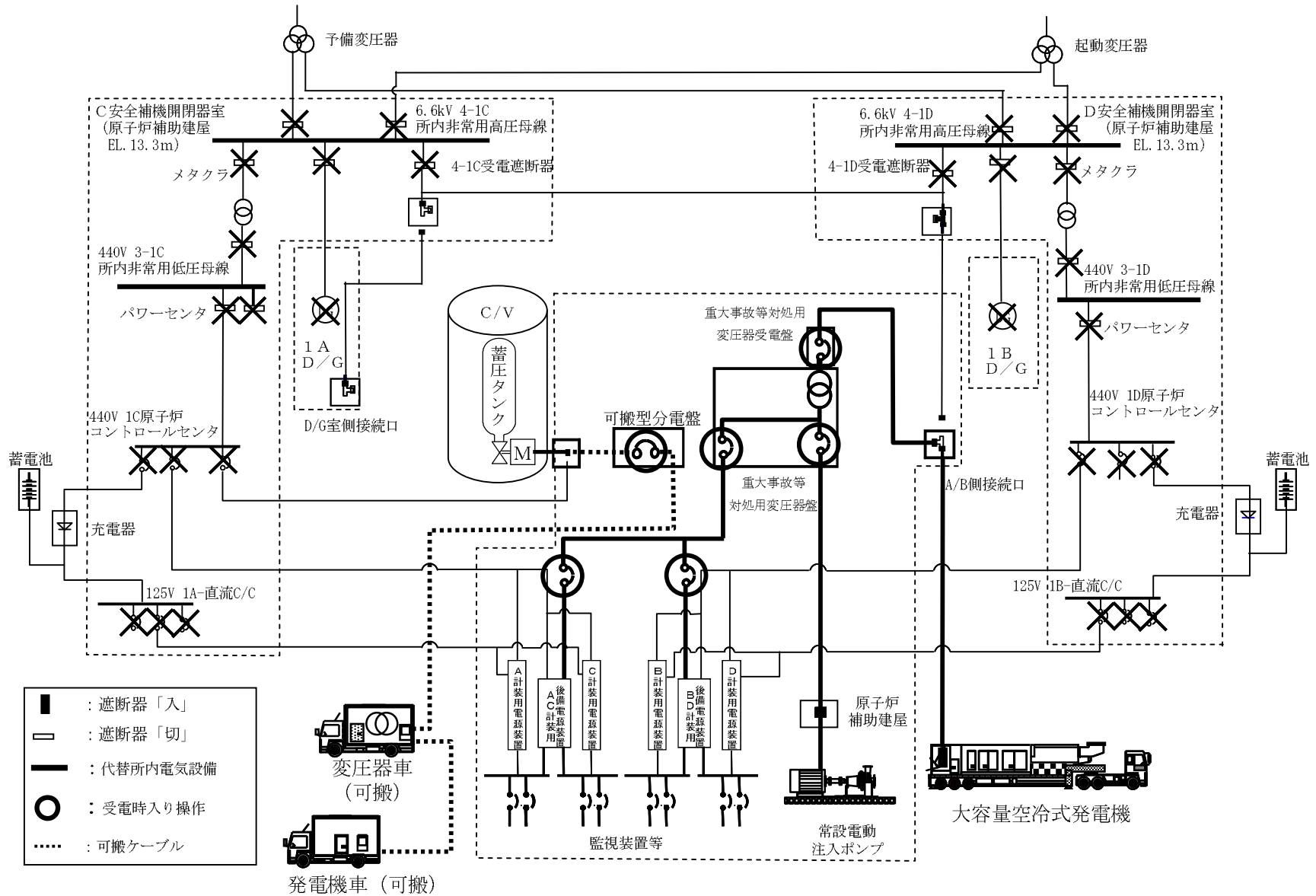
第1.8-7図 電源設備系統概要図(6)
