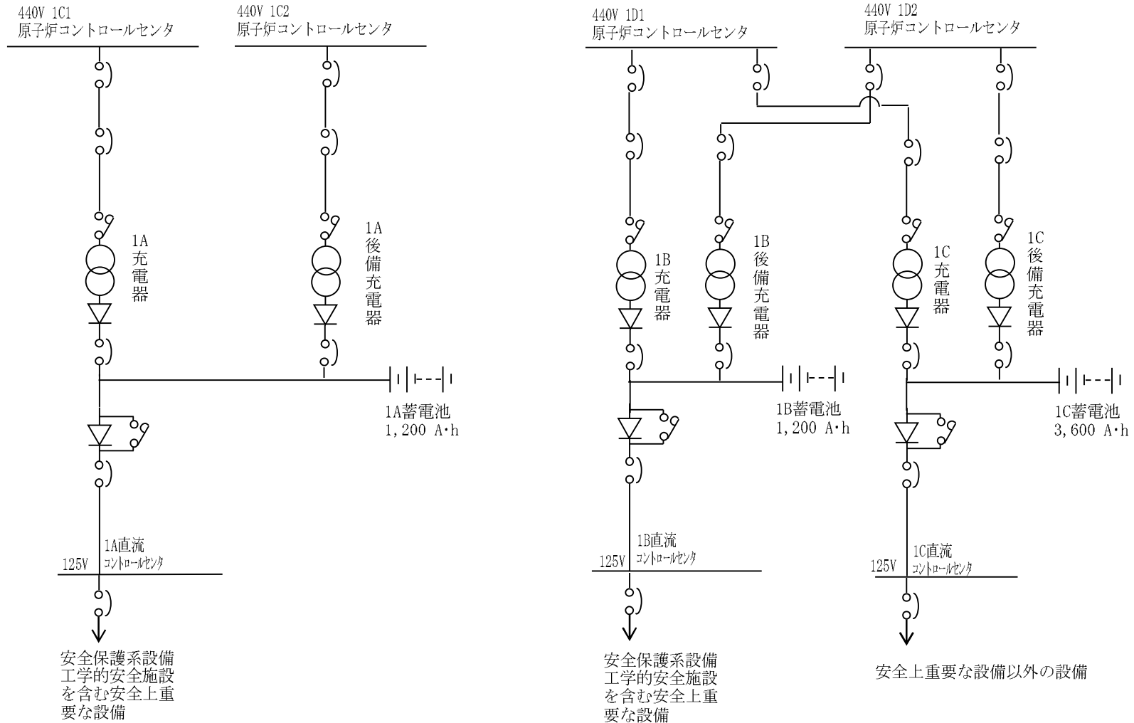
第1.8-13図 直流単線結線図
