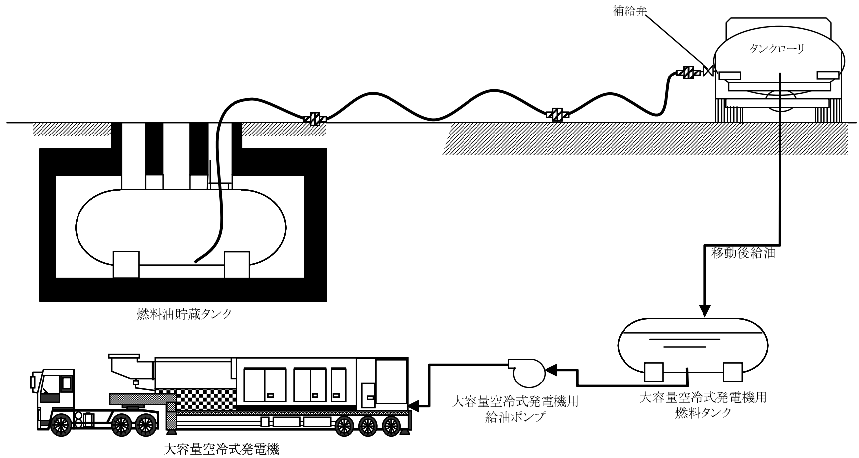
第1.8-8図 電源設備系統概要図(7)
