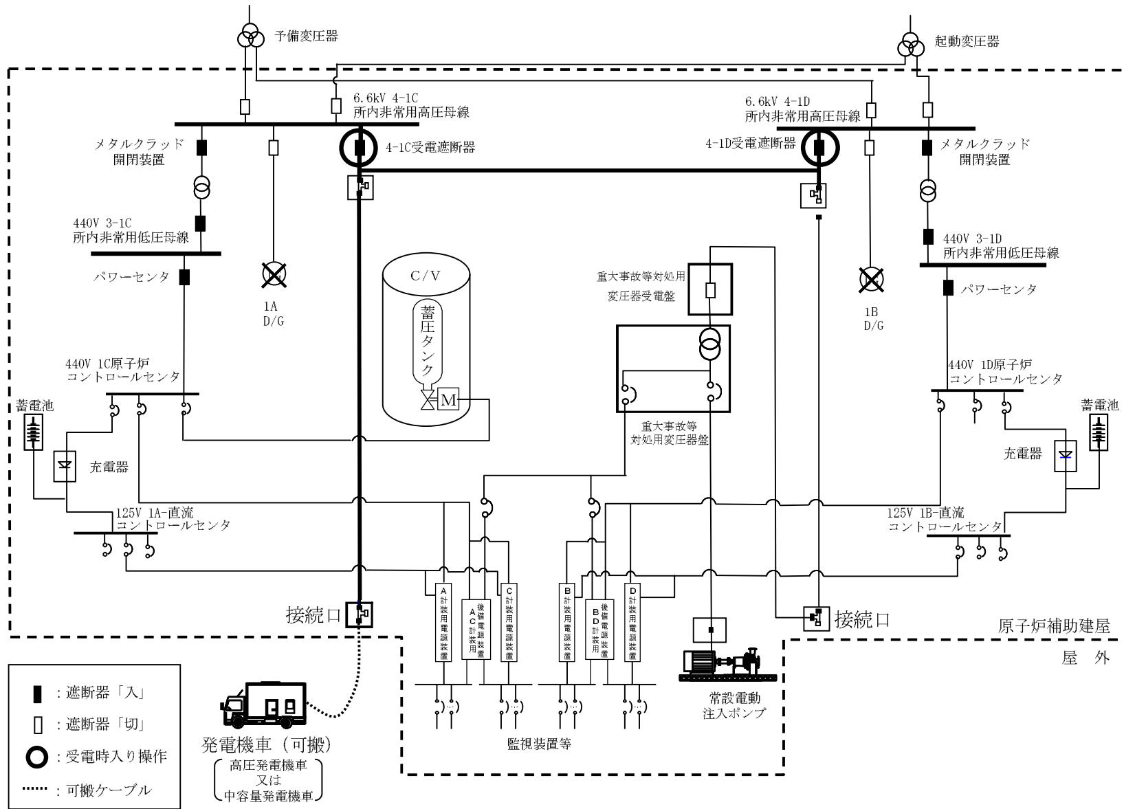
第1.8-3図 電源設備系統概要図(2)
