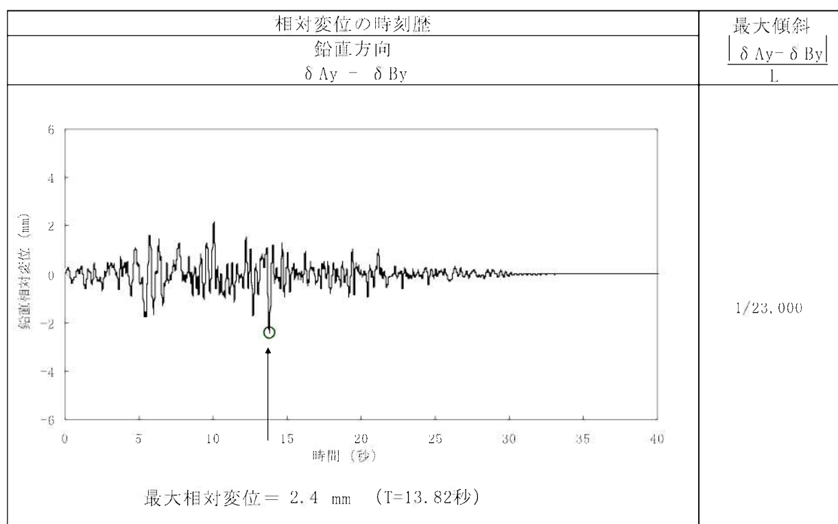
第1.2-124表(5) 原子炉建屋基礎底面両端の鉛直方向の相対変位・傾斜 (Y-Y'断面、Ss-1)(1号機)
