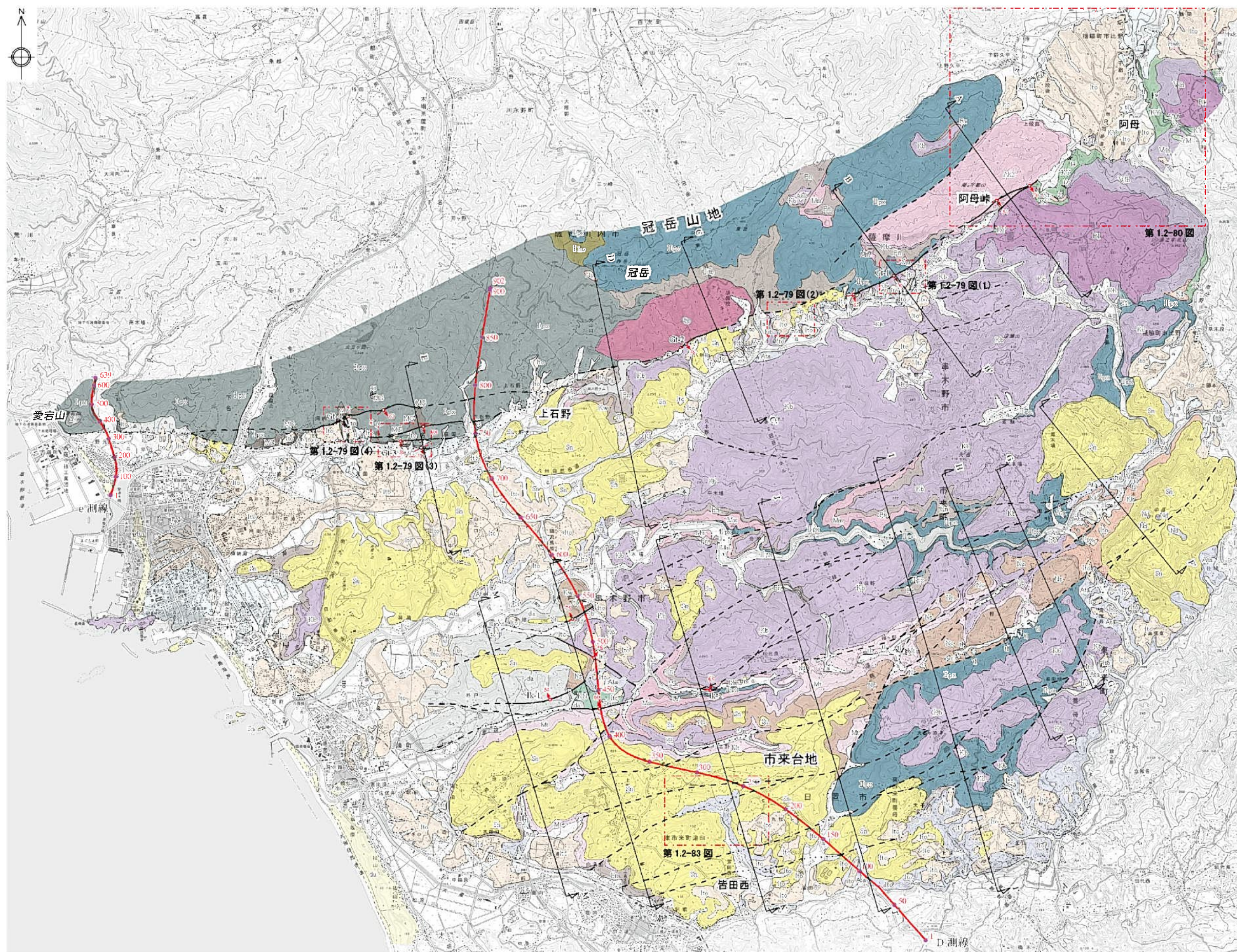
第1.2-74図 市来断層系周辺（五反田川断層含む）の地質図 1.2-523
