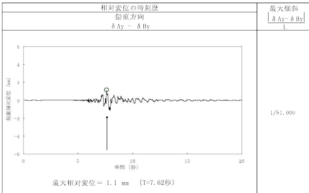
第1.2-124表(2) 原子炉建屋基礎底面両端の鉛直方向の相対変位・傾斜 ( X_{1L}-X_{1L}' 断面、Ss-2)
