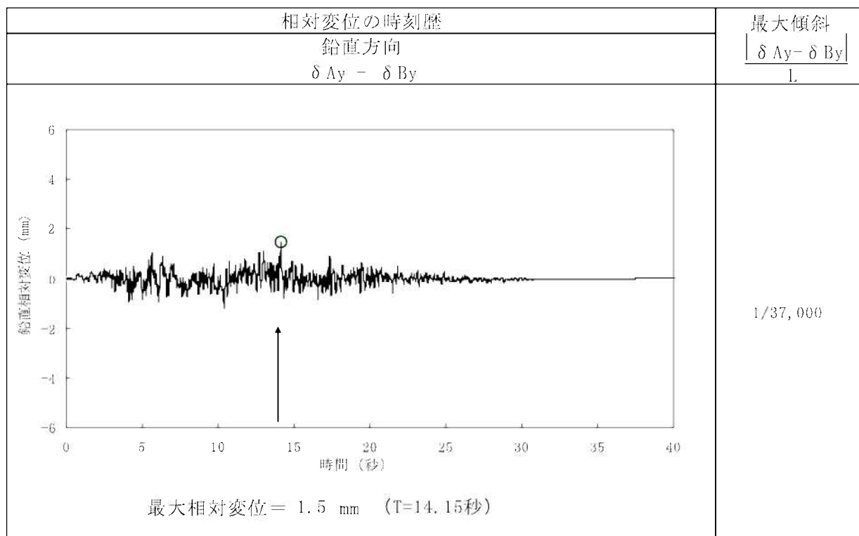
第1.2-124表(1) 原子炉建屋基礎底面両端の鉛直方向の相対変位・傾斜 ( X_{1L}-X_{1L}' 断面、Ss-1)
