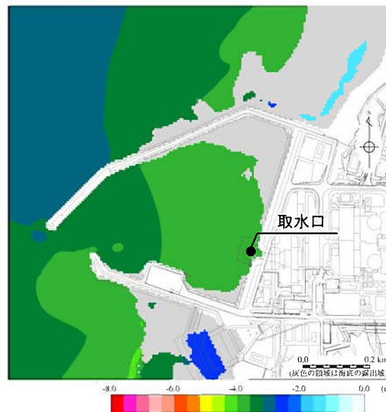
第1.2-23図(2) 基準津波の最大水位下降量分布 (初期潮位: T.P.±0.00m)
