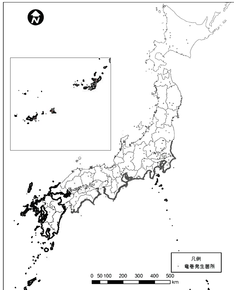
第1.2-37図 竜巻検討地域
