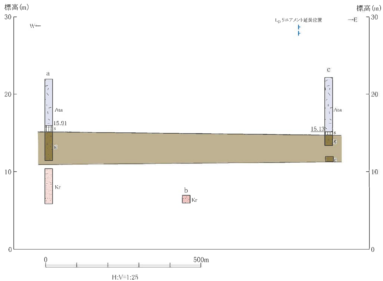
第1.2-95図 薩摩川内市戸田－庄込間の柱状対比
