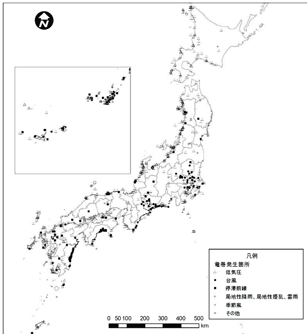
第1.2-31図 気象要因別の竜巻発生位置
