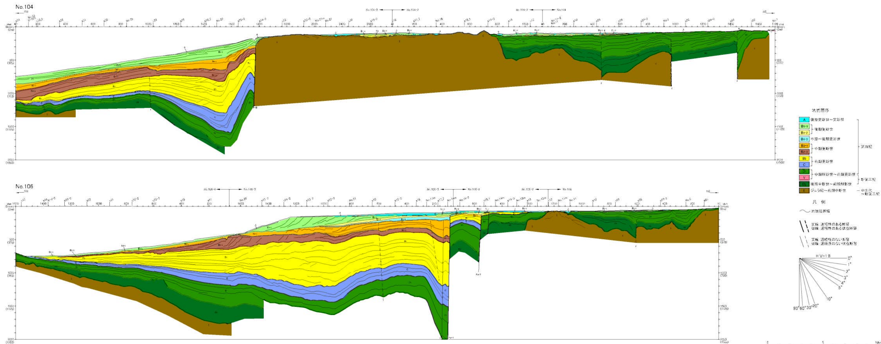
第1.2-161図(3) 敷地前面海域の海底地質断面図(その3)
