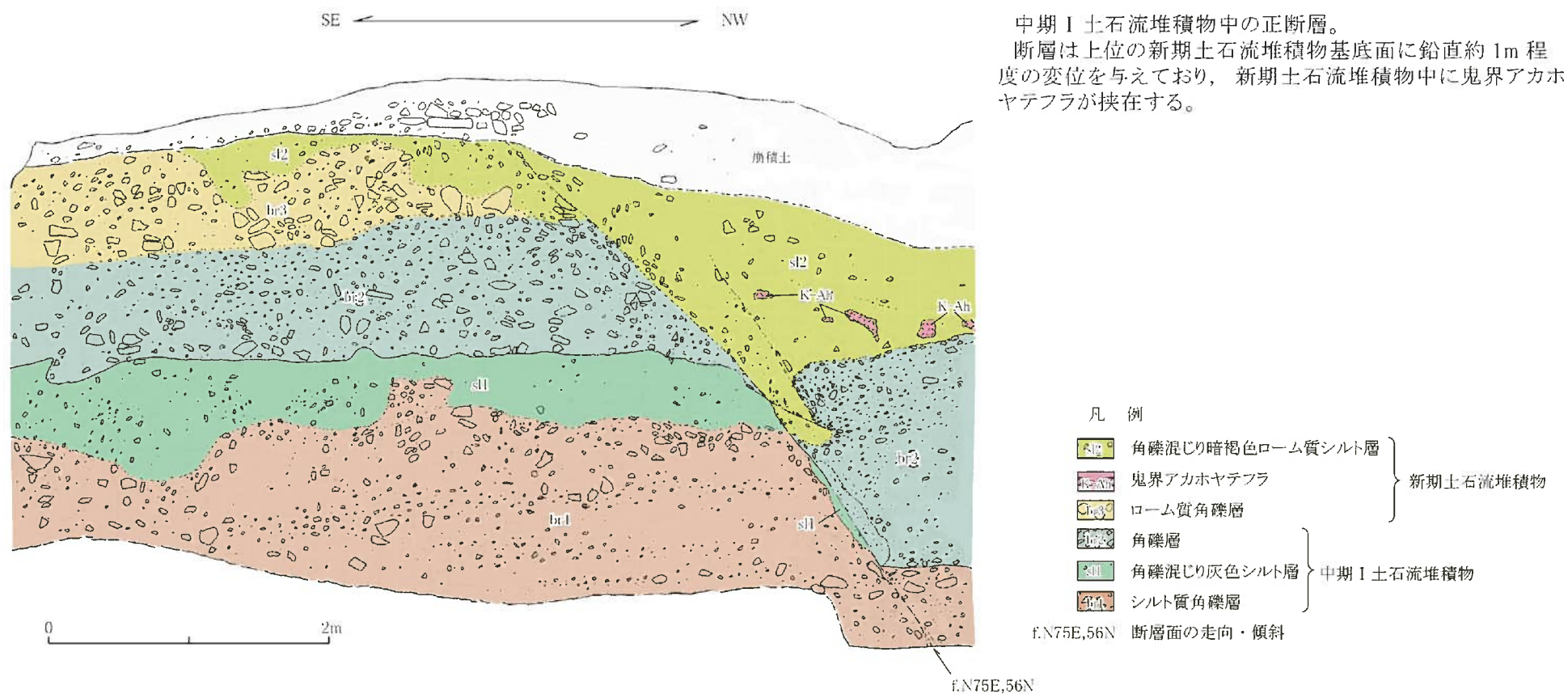
第1.2-126図(2) 露頭スケッチ (Loc.Tz-2, 薩摩川内市須口池南西)
