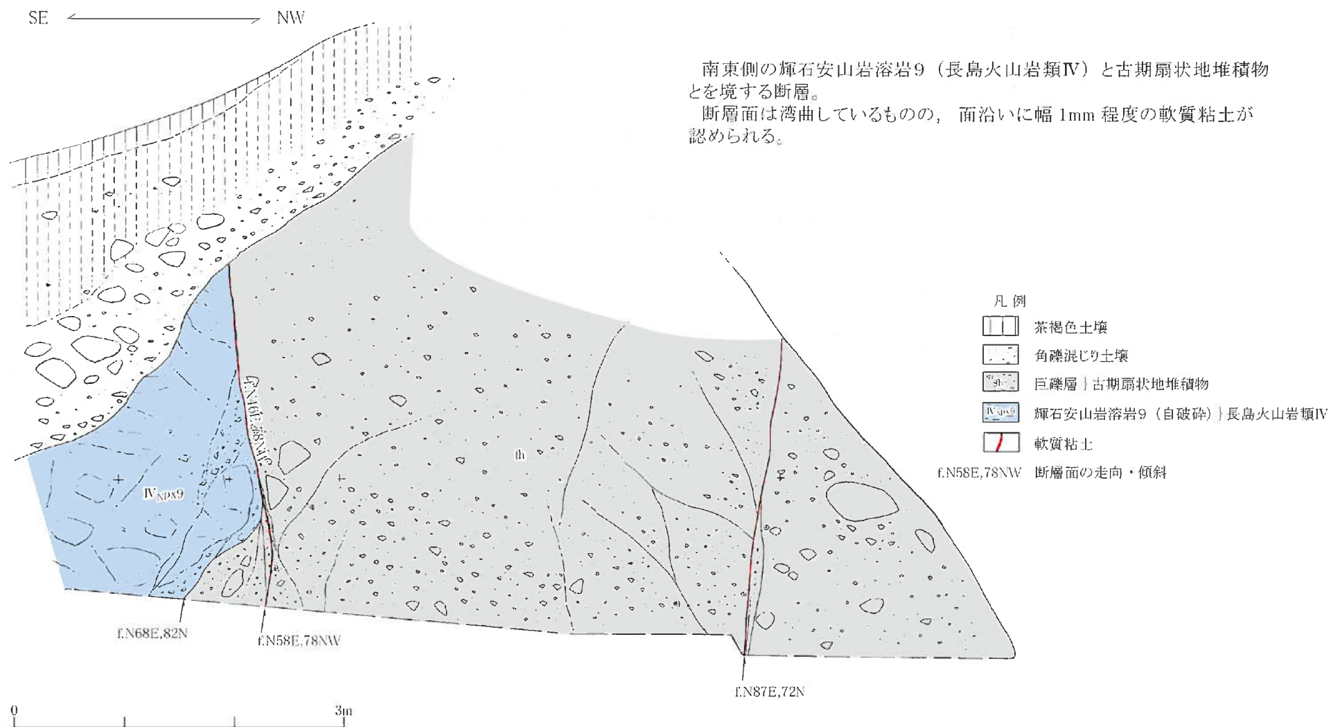
第1.2-120図(3) 露头スケッチ (Loc.Ky-3, 出水市連尺野)
