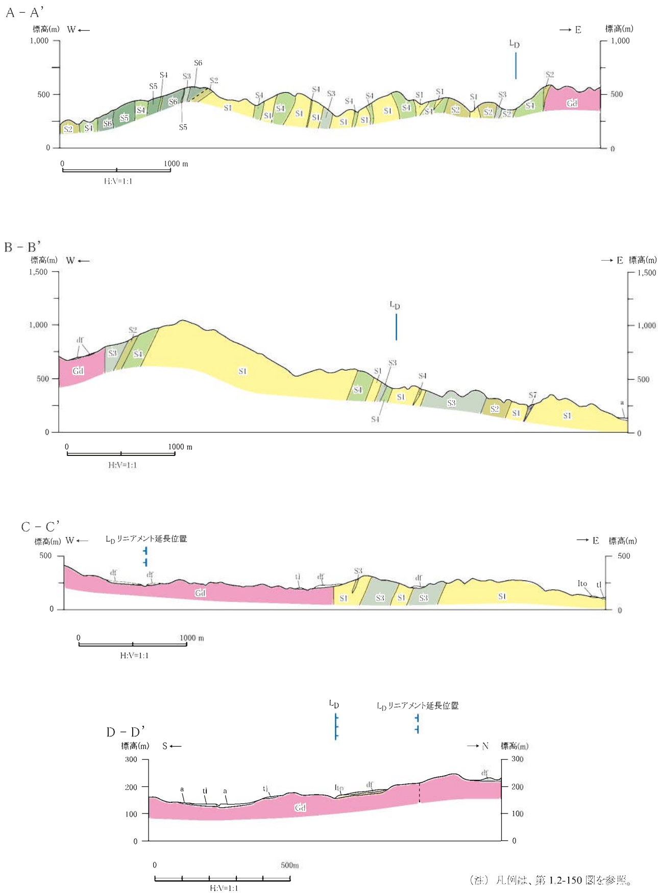
第 1.2-151 図 紫尾山南・泊野リニアメント周辺の地質断面図
