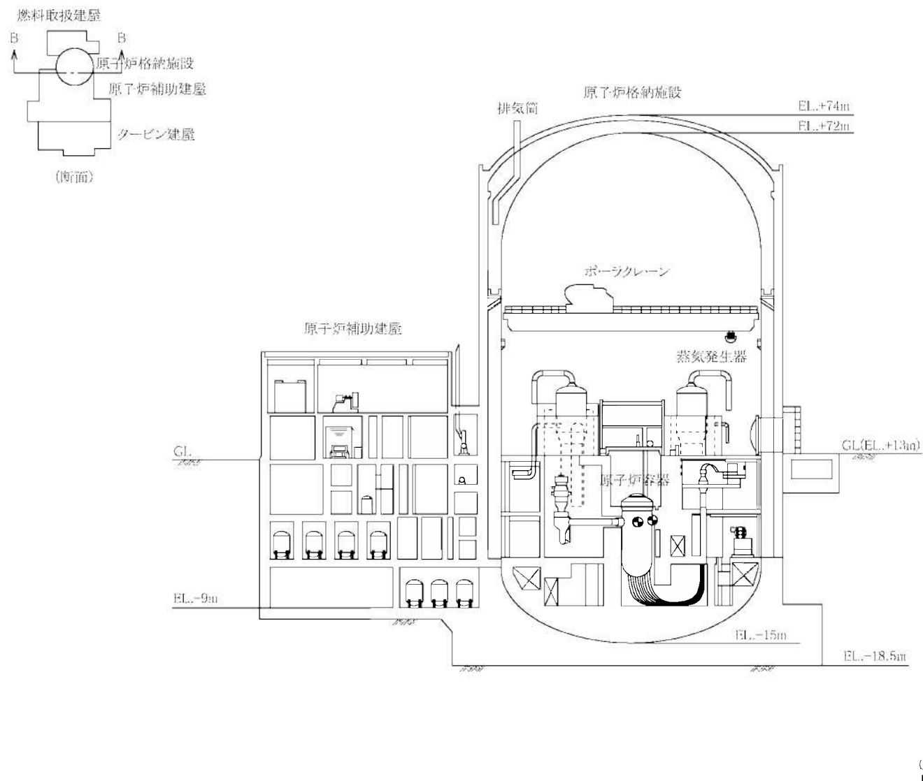
第1.9-33図 主要建屋断面図(B-B断面)
