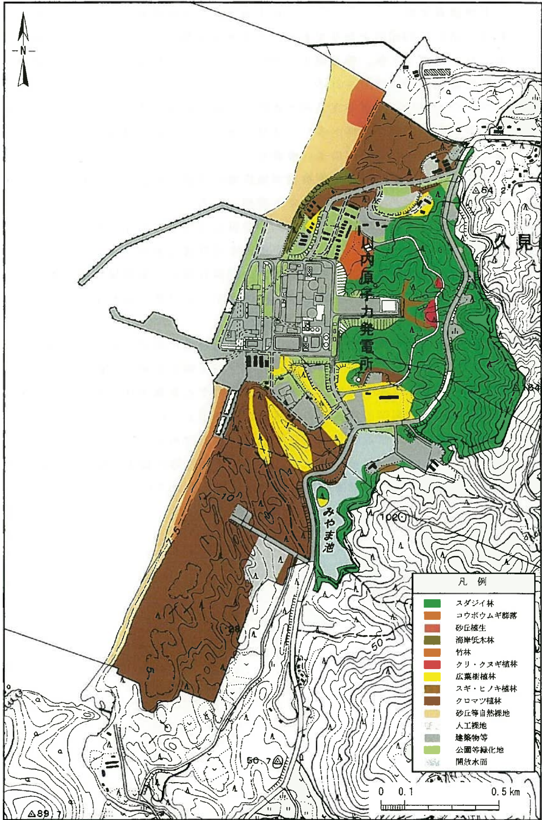
第1.20-2図 川内原子力発電所の植生
