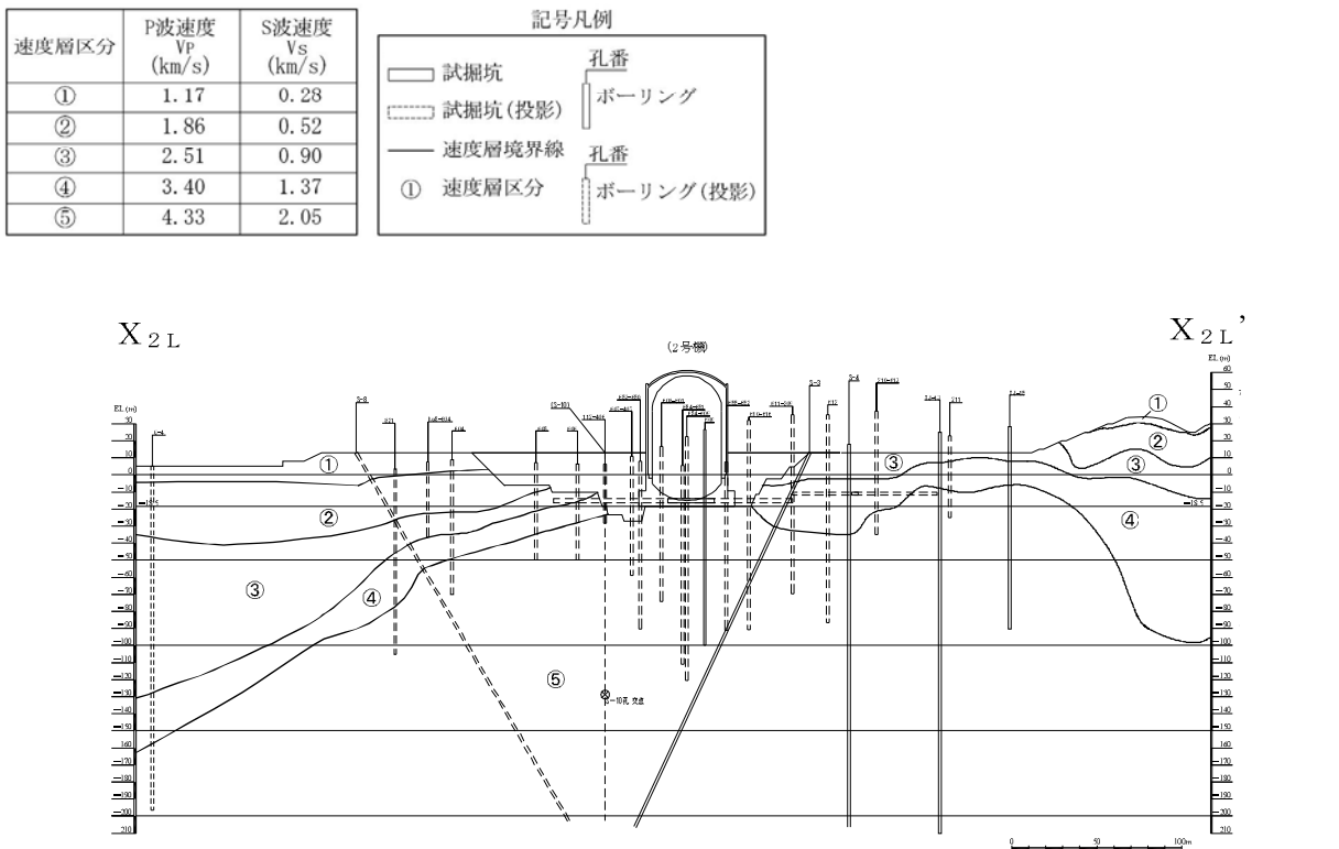
第1.2-330図(2) 速度層断面図(X 2L —X 2L '断面)
