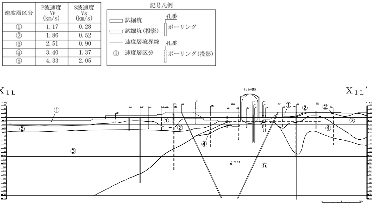
第1.2-330図(1) 速度層断面図(X 1L —X 1L '断面)
