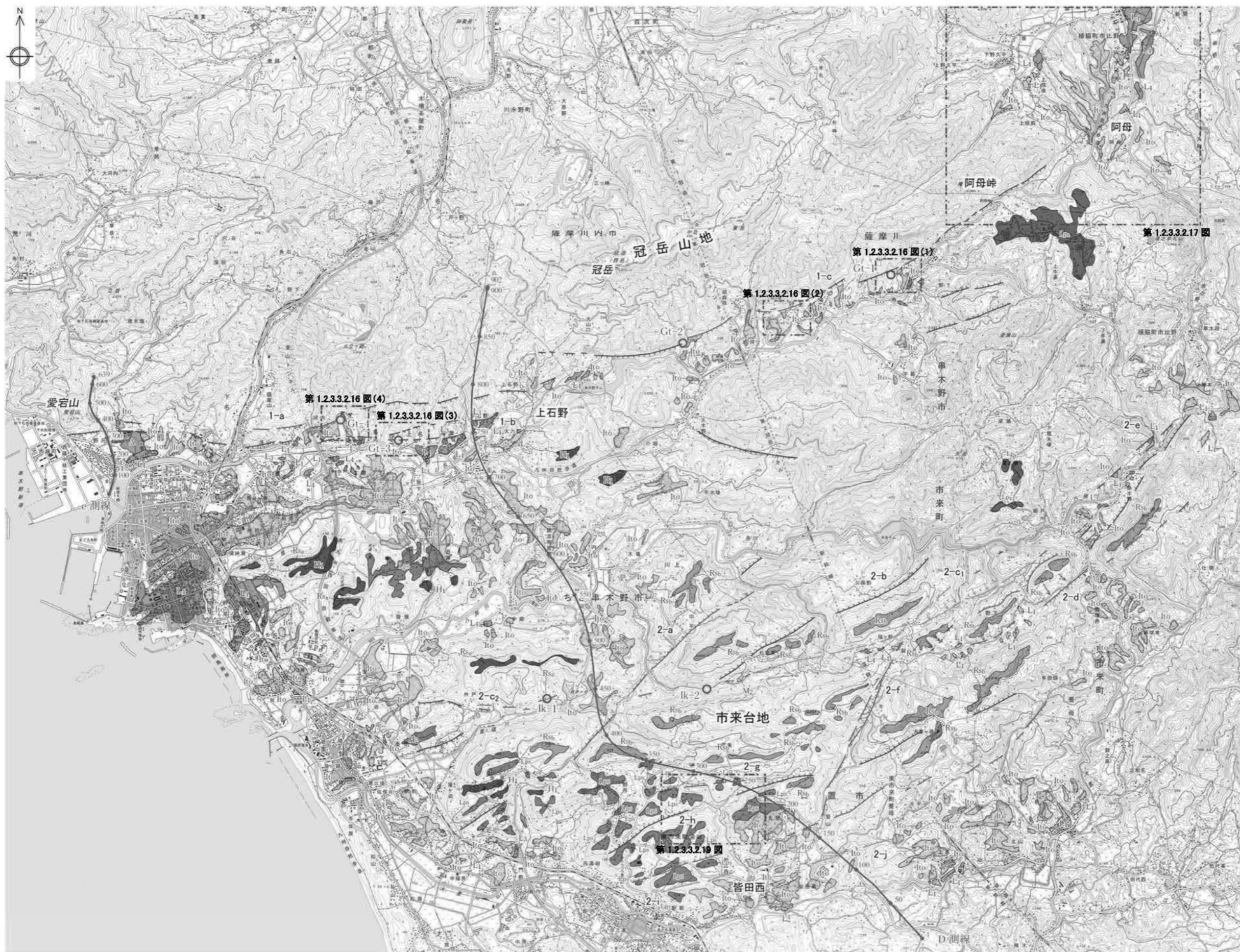
第 1.2.3.3.2.10 図 市来断層系周辺(五反田川断層含む)の空中写真判読図
