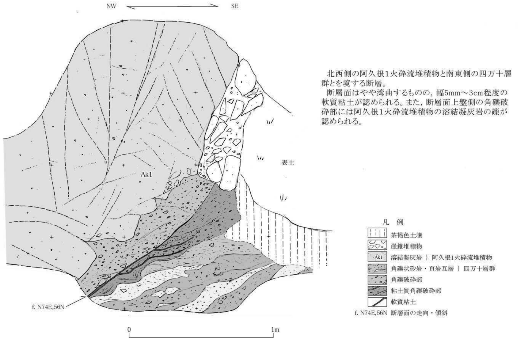
第 1.2.3.3.2.41 図 露頭スケッチ (Loc.Iz-4, 出水市野田町上特手)
