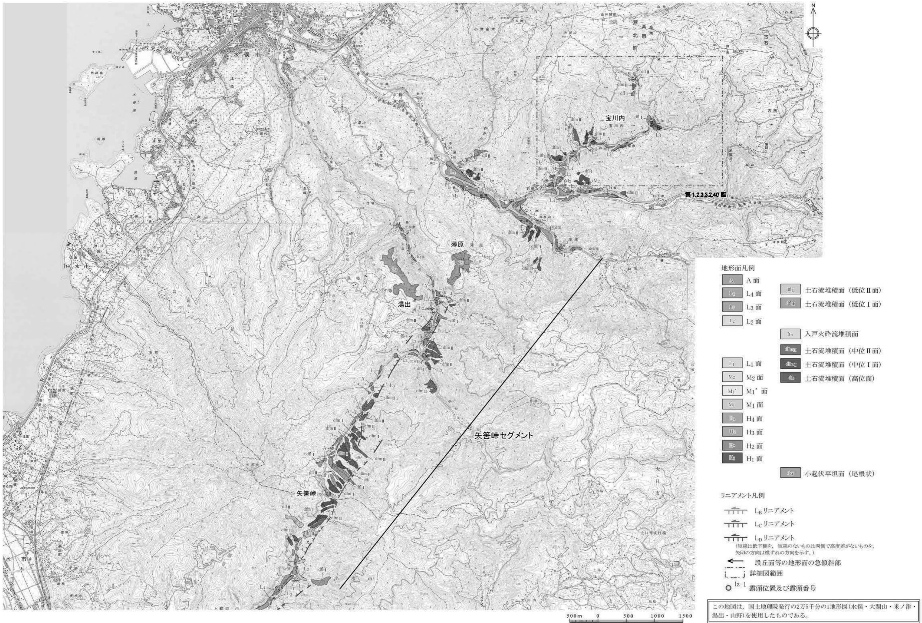
第 1.2.3.3.2.36 図(1) 出水断層系周辺の空中写真判読図(北部)
