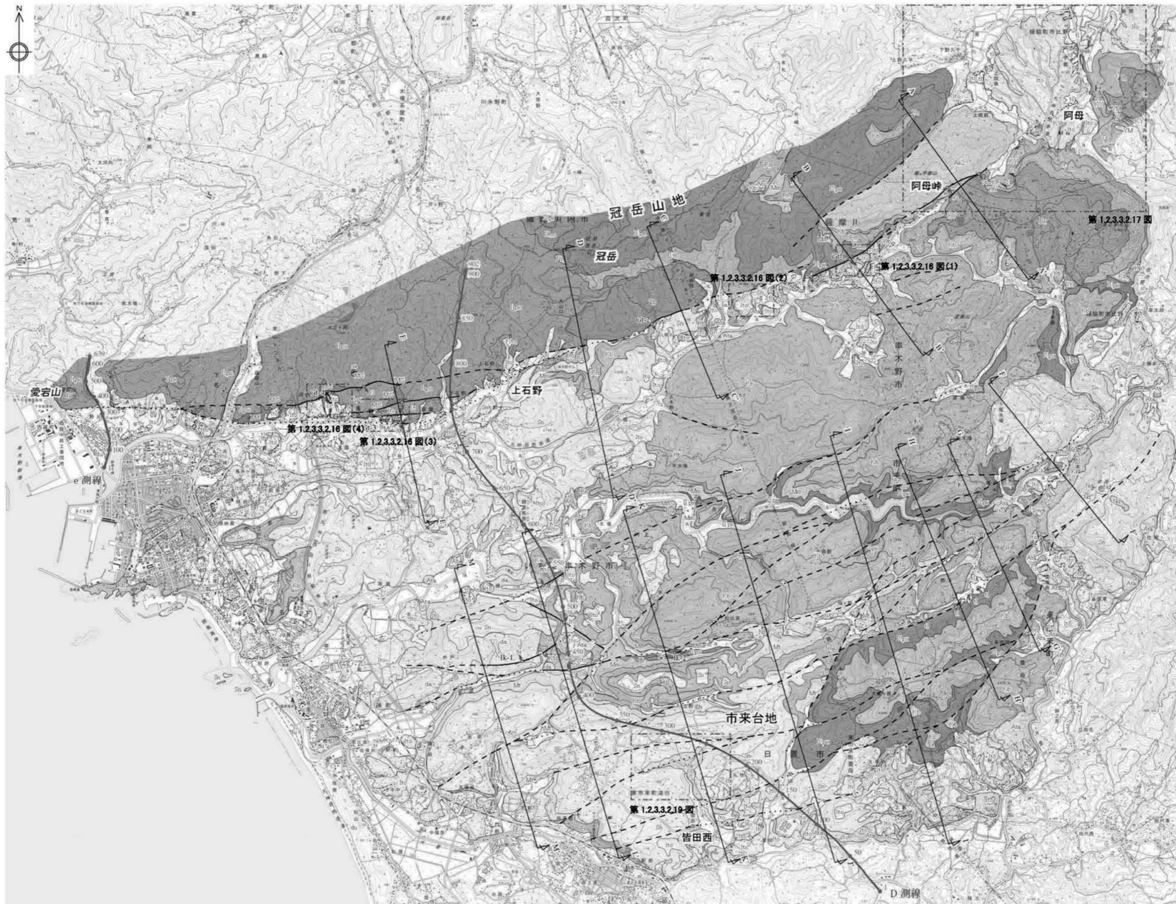
第 1.2.3.3.2.11 図 市来断層系周辺(五反田川断層含む)の地質図
