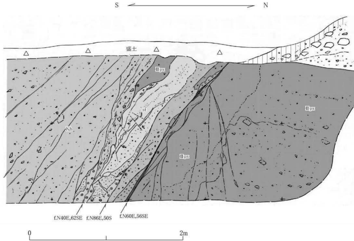
第 1.2.3.3.2.15 図(1) 露頭スケッチ (Loc.Gt-1, 薩摩川内市野下)
