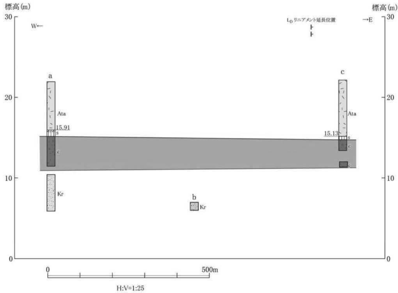
第 1.2.3.3.2.31 図 薩摩川内市戸田一庄込間の柱状対比
