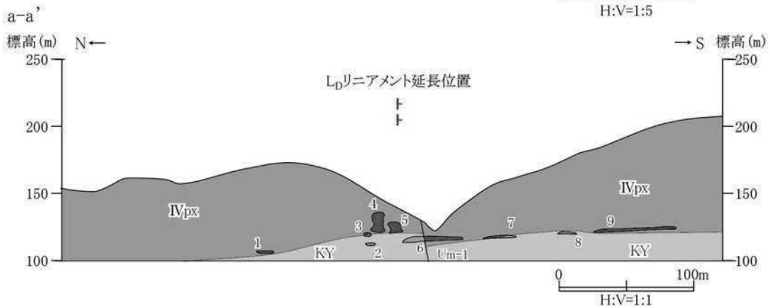
第 1.2.3.3.2.24 図 ルートマップ及び地形・地質断面図(薩摩川内市八重付近)
