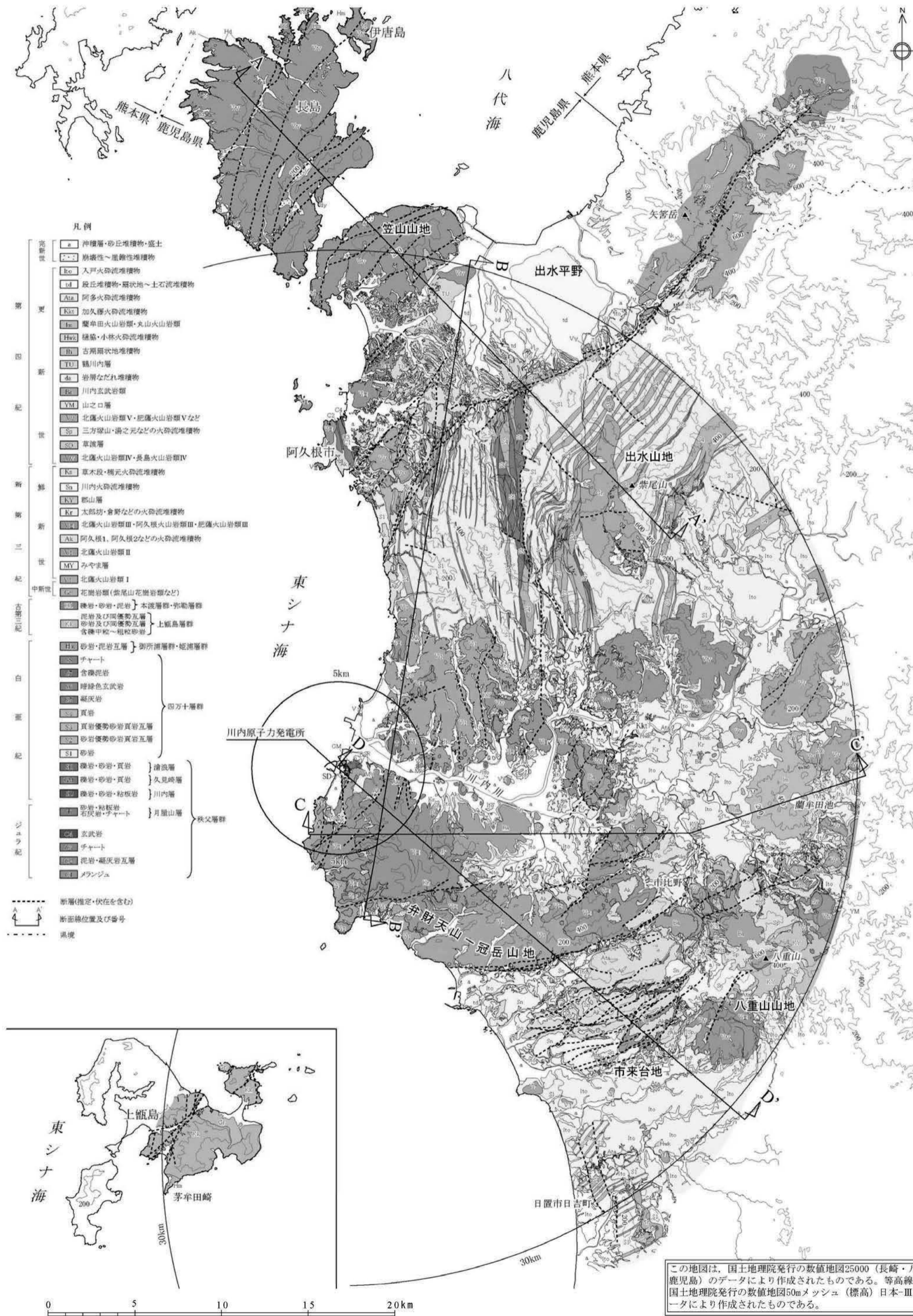
第 1.2.3.3.2.2 図 敷地周辺陸域の地質図
