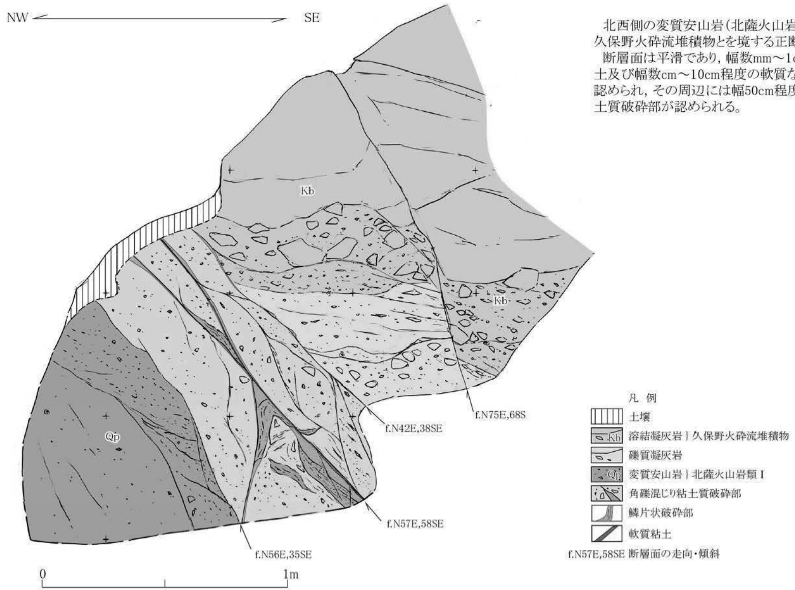
第 1.2.3.3.2.15 図(2) 露頭スケッチ (Loc.Gt-2, いちき串木野市八牟礼)
