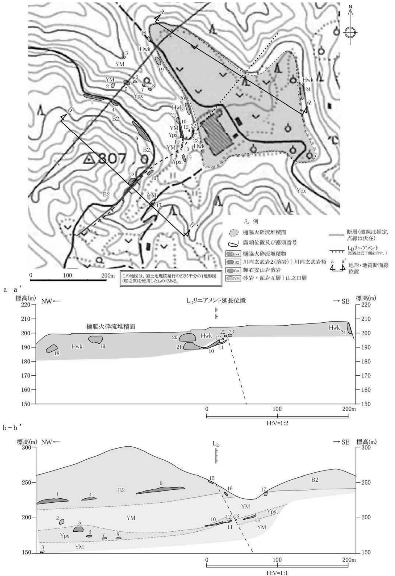
第 1.2.3.3.2.25 図 ルートマップ及び地形・地質断面図(薩摩川内市中山北方付近)
