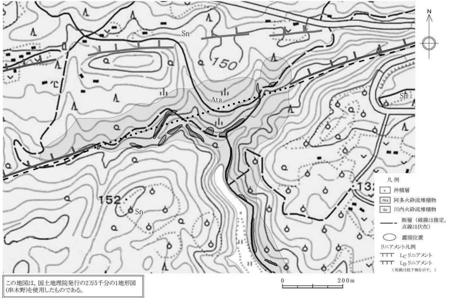
第 1.2.3.3.2.19 図 ルートマップ(日置市皆田西北方付近)
