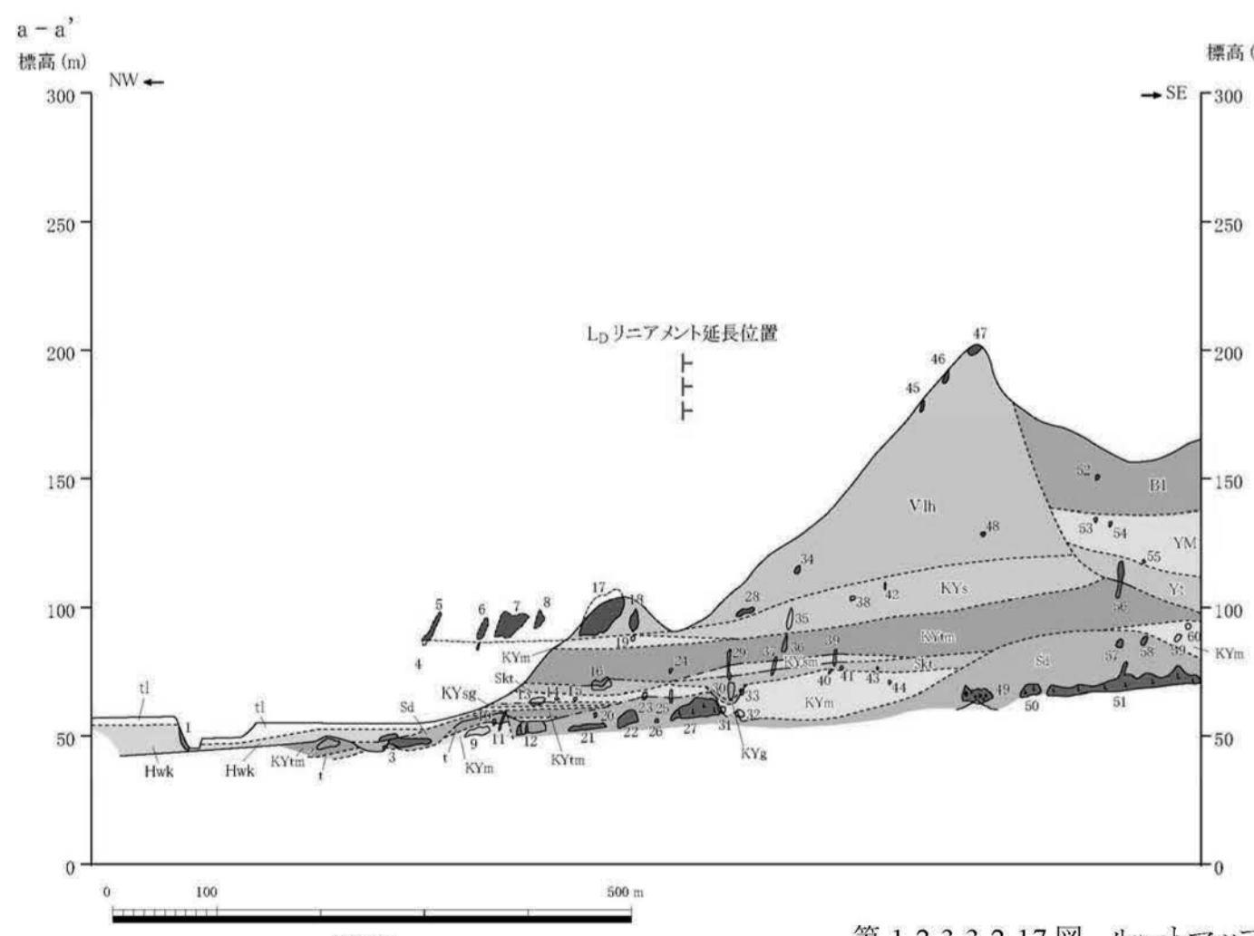
第 1.2.3.3.2.17 図 ルートマップ・地質断面図(薩摩川内市阿母付近)
