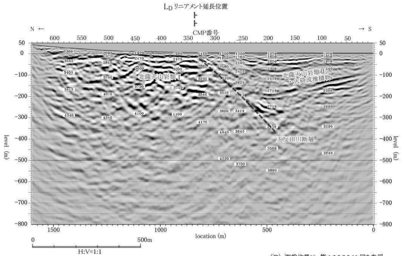
第 1.2.3.3.2.14 図(2) 反射法地震探査による深度断面とその解釈 (e測線)
