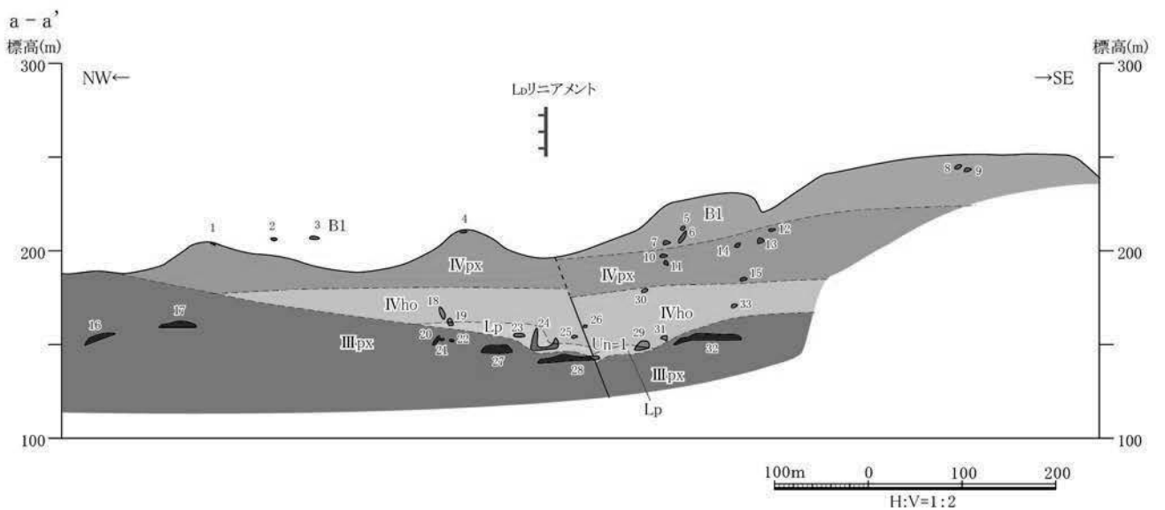
第 1.2.3.3.2.33 図 ルートマップ・地質断面図(薩摩川内市皿山北東付近)
