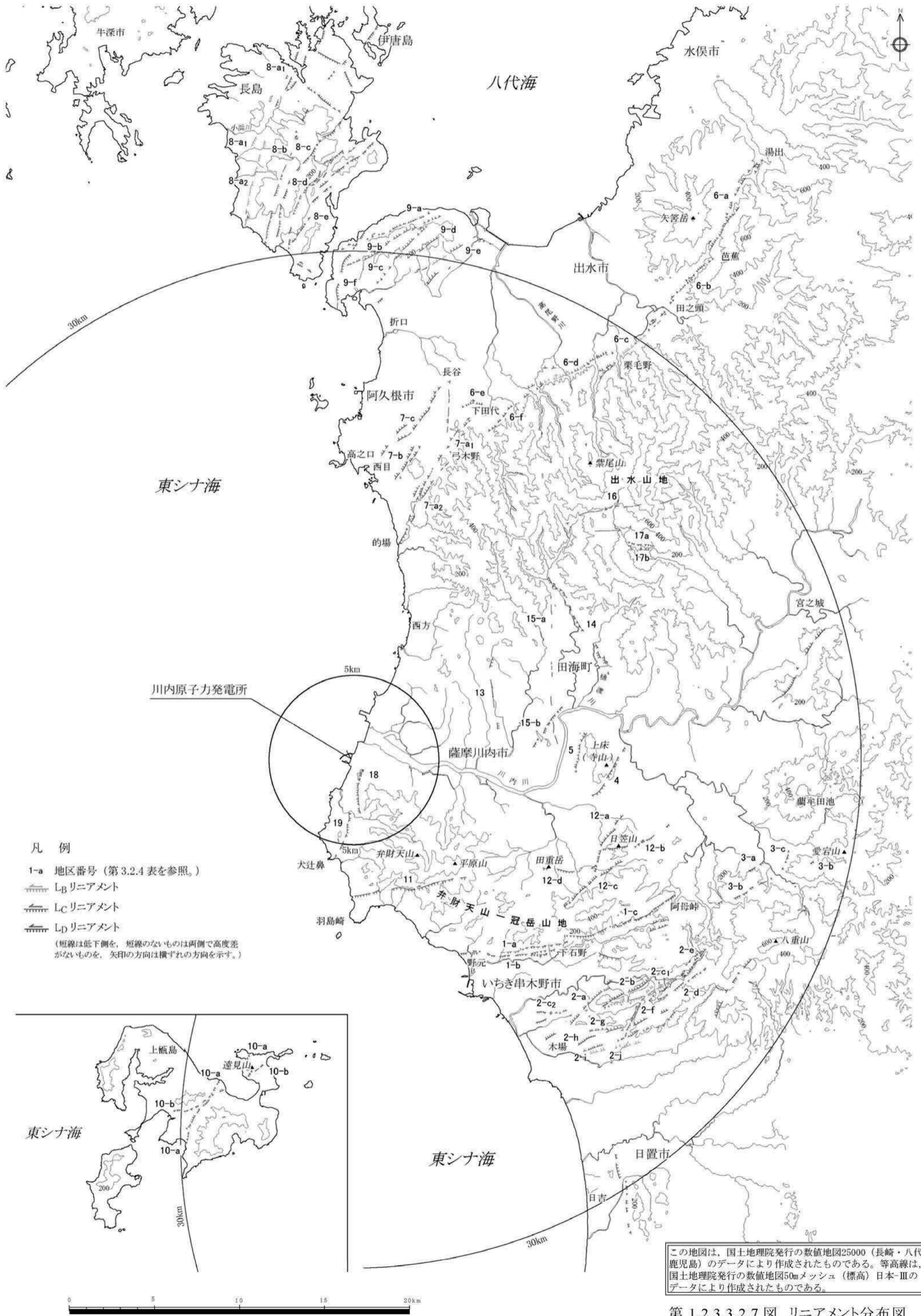
第 1.2.3.3.2.7 図 リニアメント分布図
