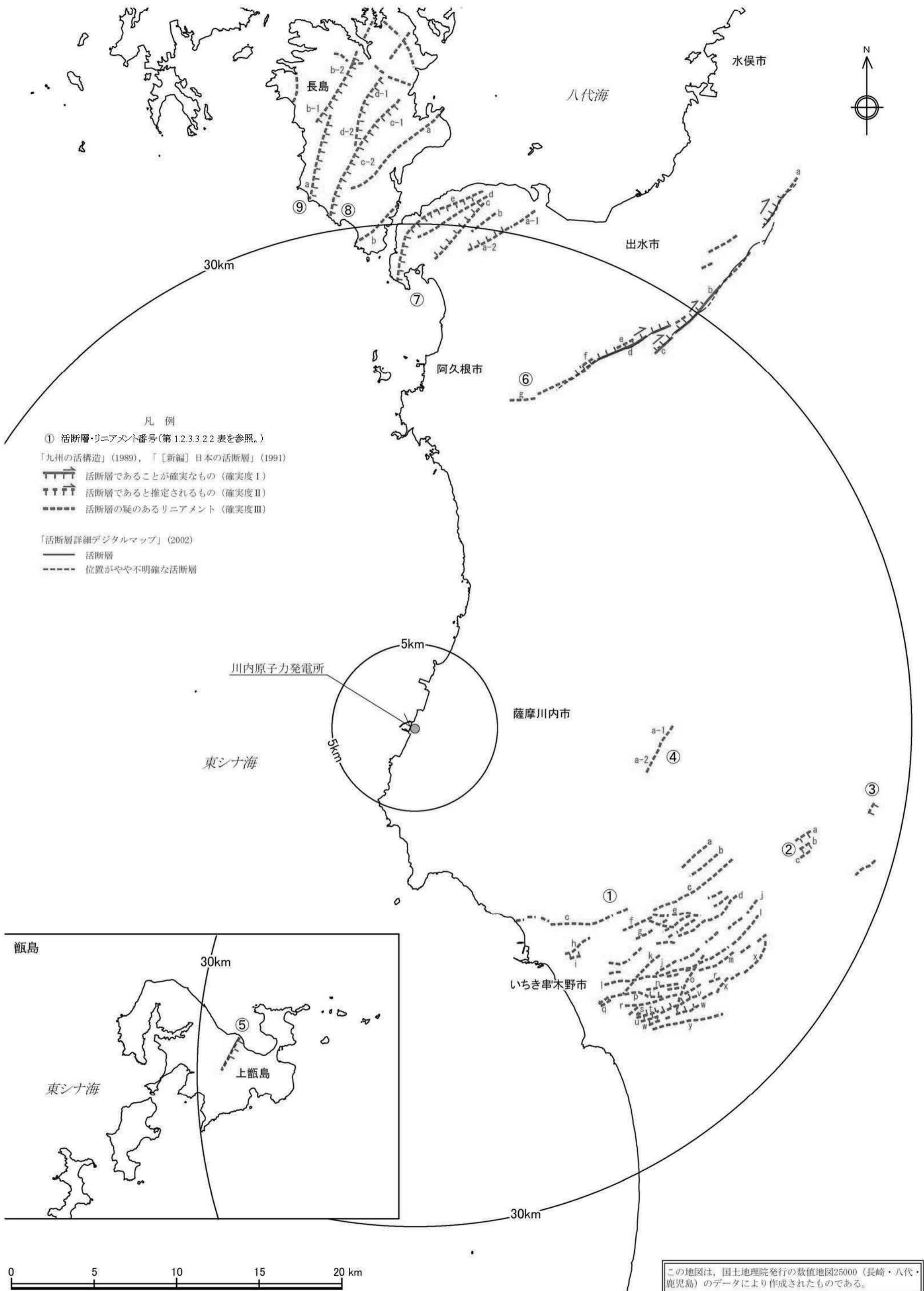
第 1.2.3.3.2.6 図 文献による活断層・リニアメント分布図
