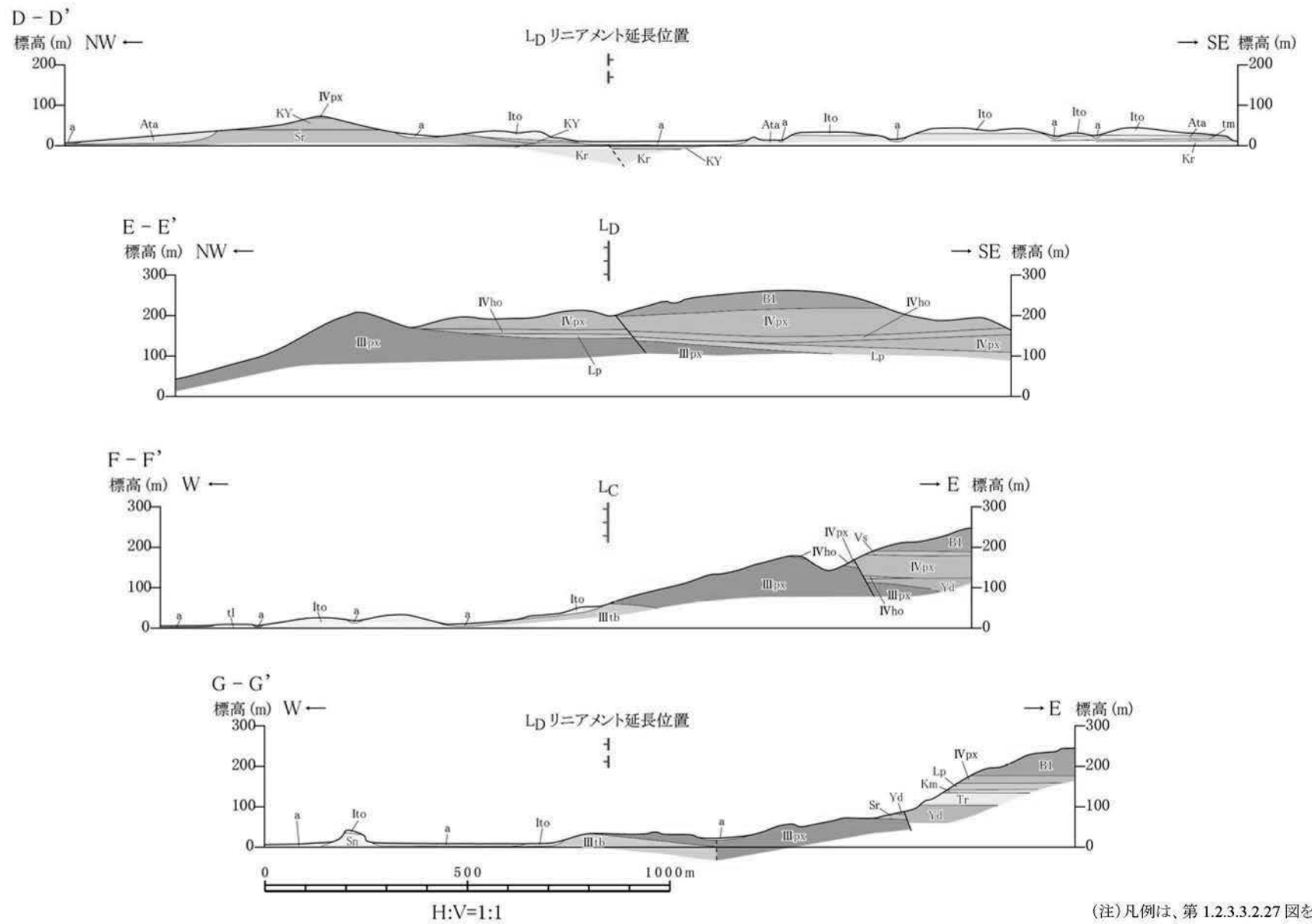
第 1.2.3.3.2.32 図 上床西リニアメント周辺の地質断面図
