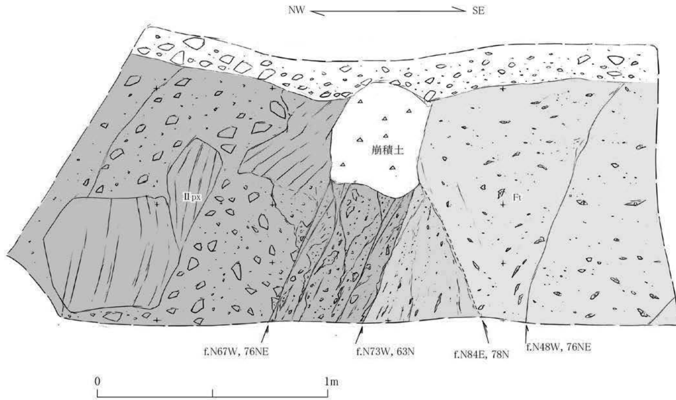
第 1.2.3.3.2.18 図(2) 露頭スケッチ (Loc.Ik-2, いちき串木野市松比良南西)
