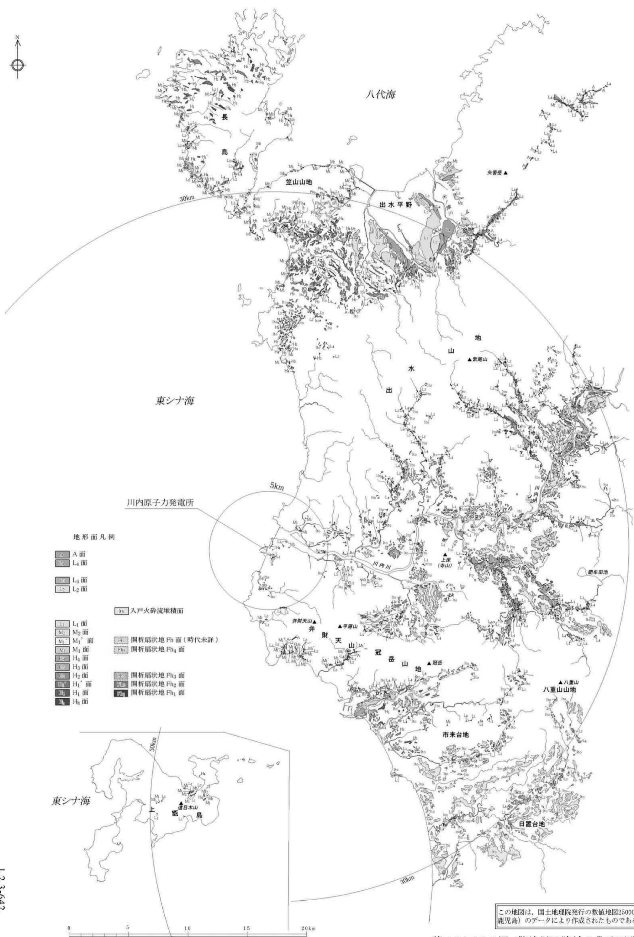
第 1.2.3.3.2.4 図 敷地周辺陸域の段丘面分布図
