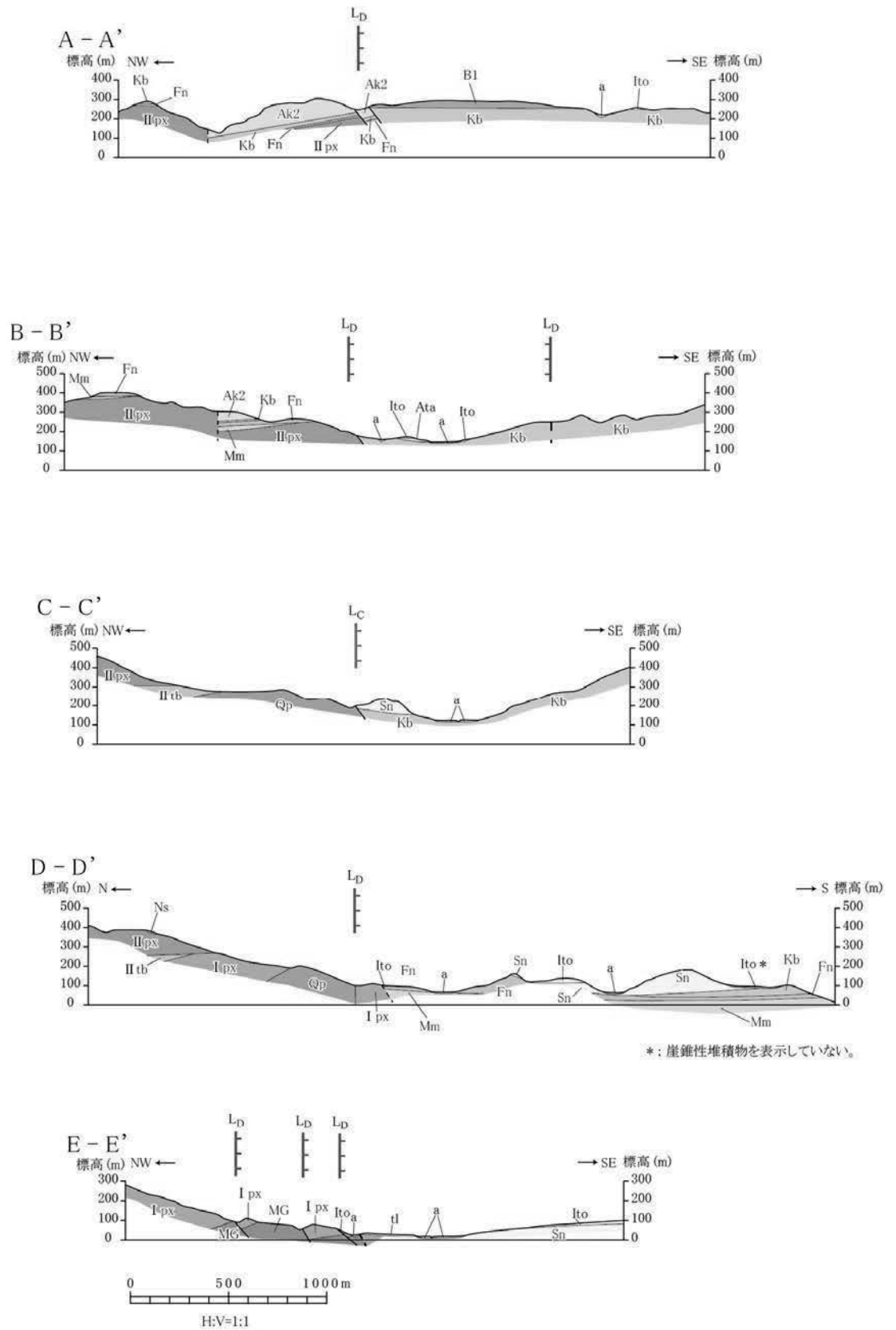
第 1.2.3.3.2.12 図 五反田川断層周辺の地質断面図
