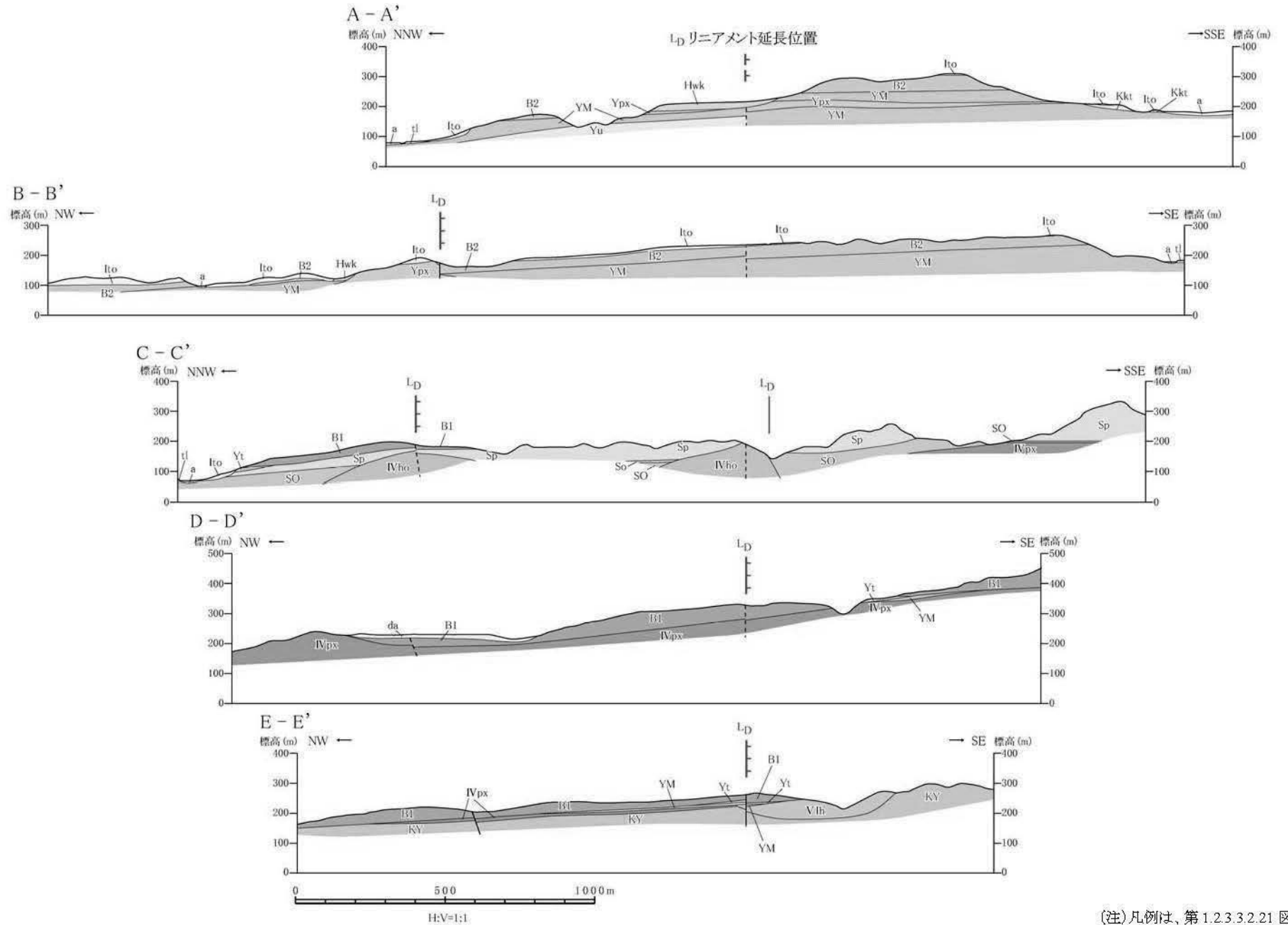
第1.2.3.3.2.22図 浦之名断層系周辺の地質断面図
