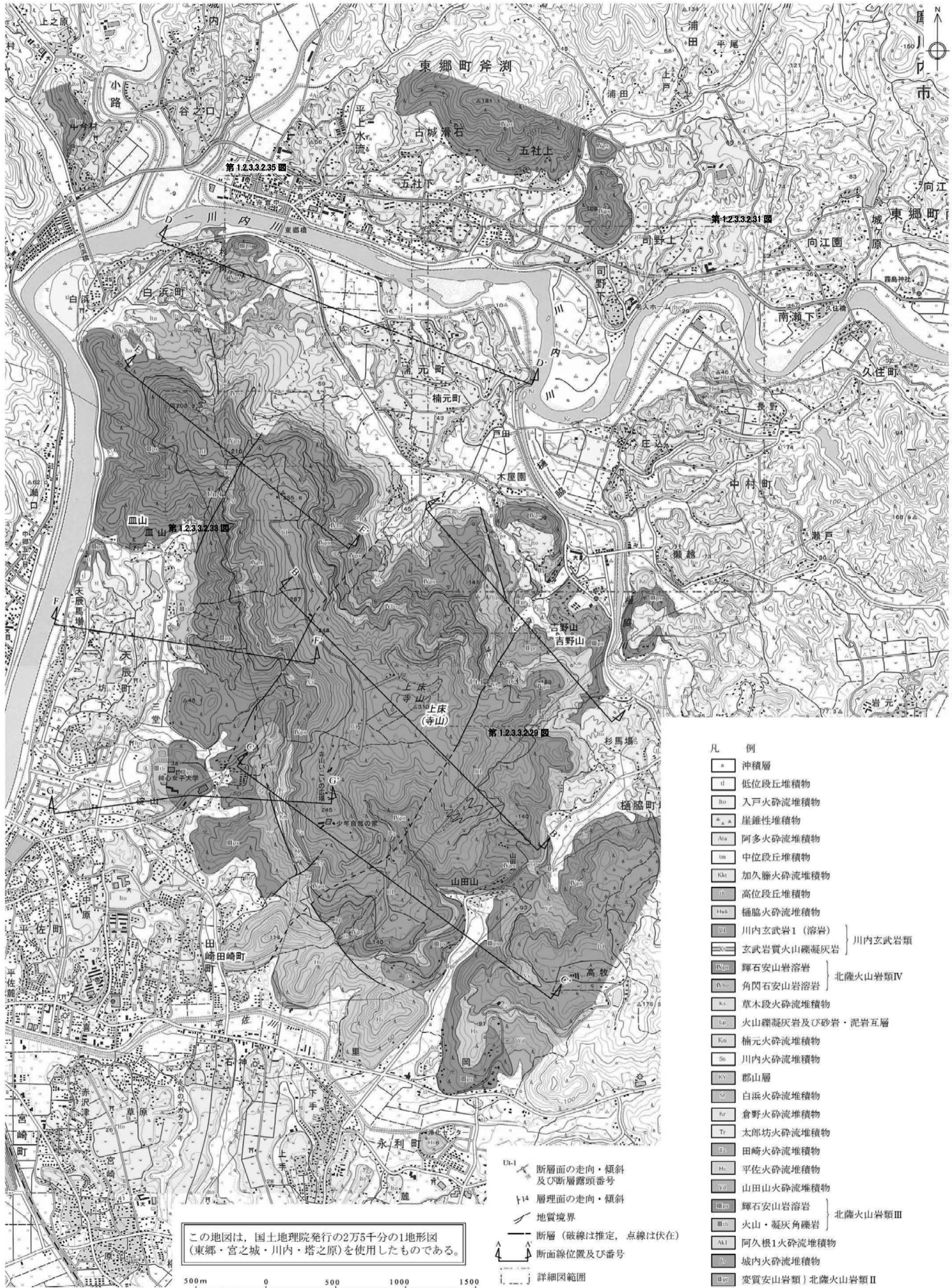
第 1.2.3.3.2.27 図 上床断層及び上床西リニアメント周辺の地質図
