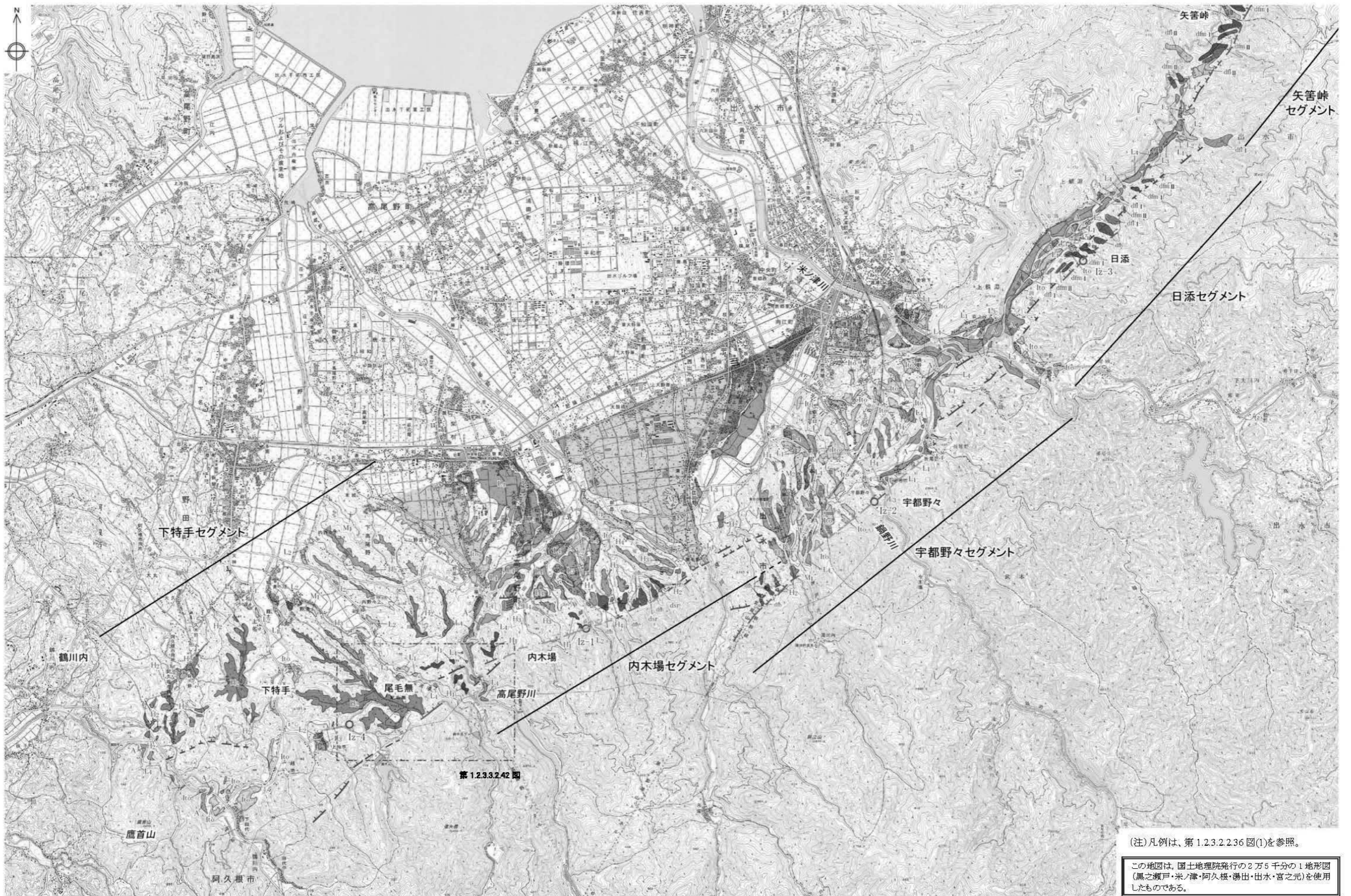
第 1.2.3.3.2.36 図(2) 出水断層系周辺の空中写真判読図(南部)
