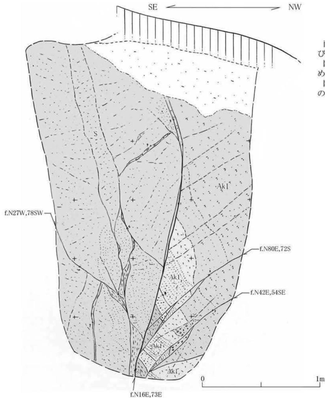
第 1.2.3.3.2.46 図(1) 露頭スケッチ (Loc.A-1, 阿久根市弓木野南方)
