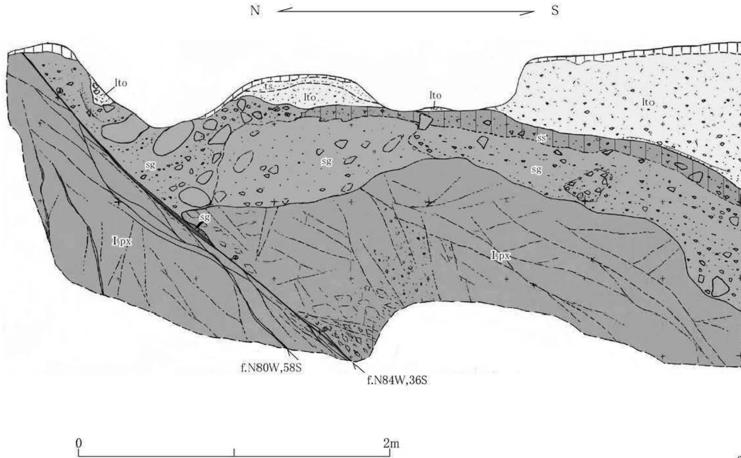
第 1.2.3.3.2.15 図(3) 露頭スケッチ (Loc.Gt-3, いちき串木野市上名)
