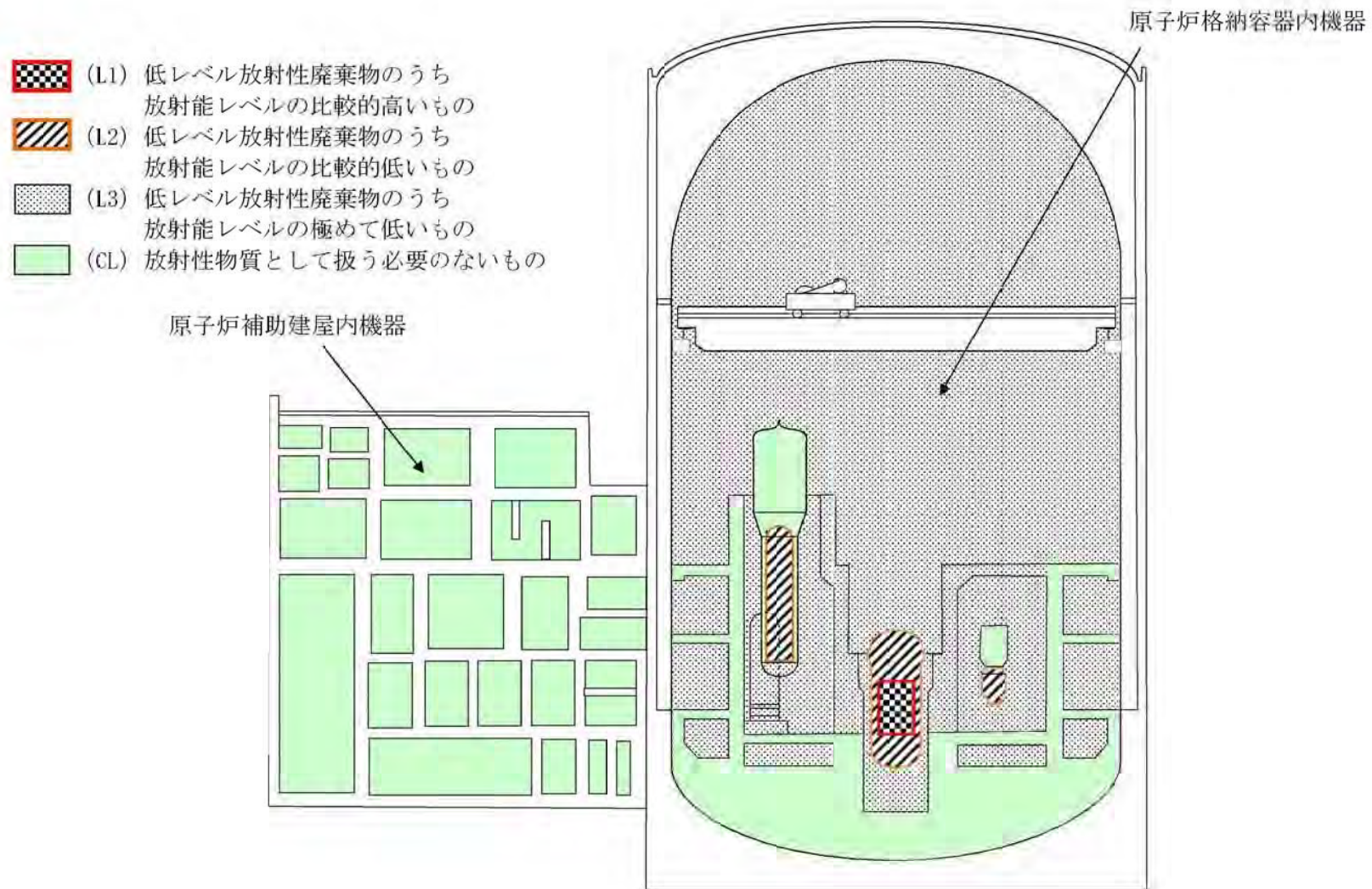
第 1.21-1 図 主な廃止措置対象施設の推定汚染分布
