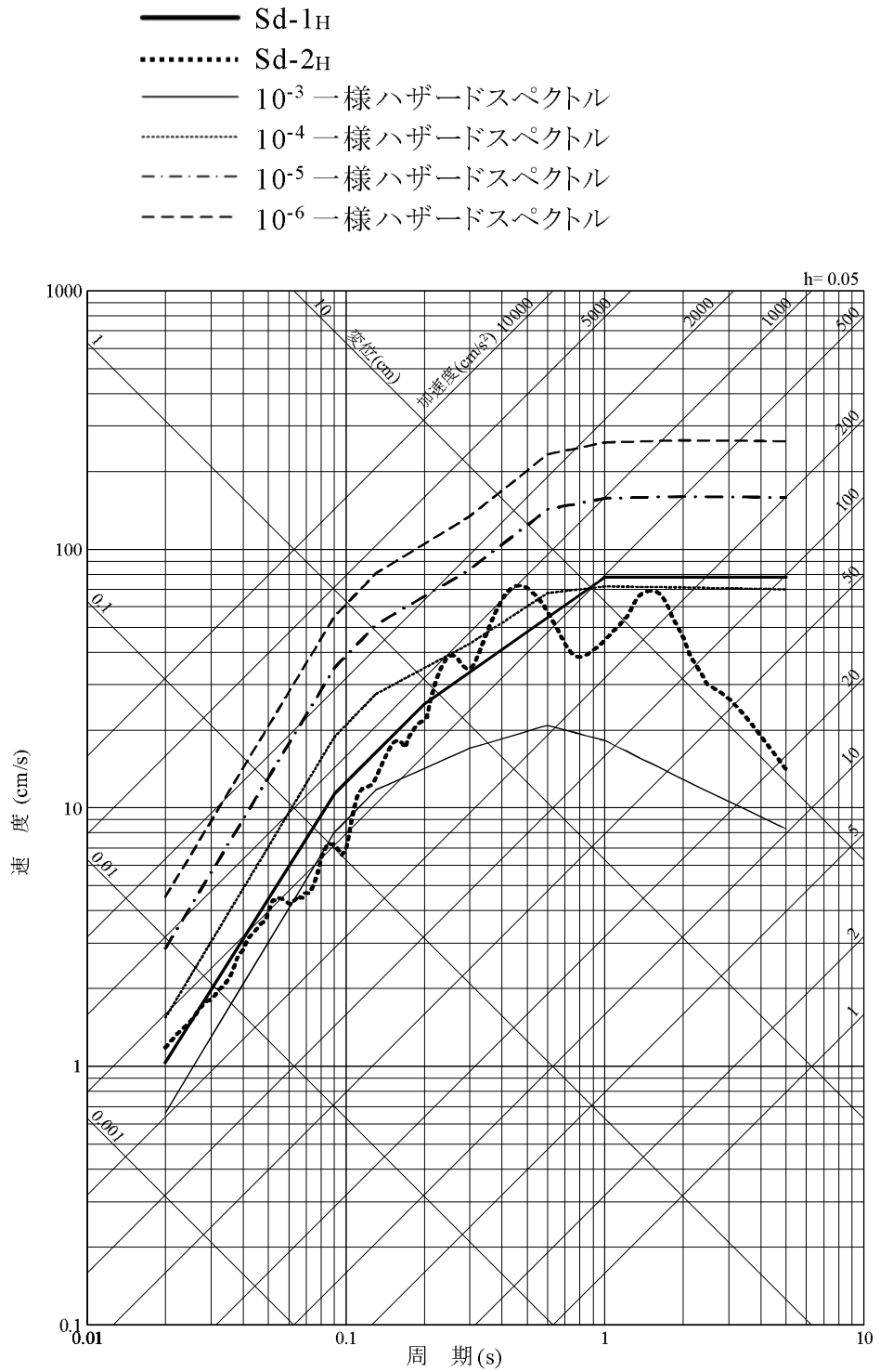
第1.3-22図 弾性設計用地震動の応答スペクトル及び解放基盤表面における地震動の一様ハザードスペクトル(水平方向)
