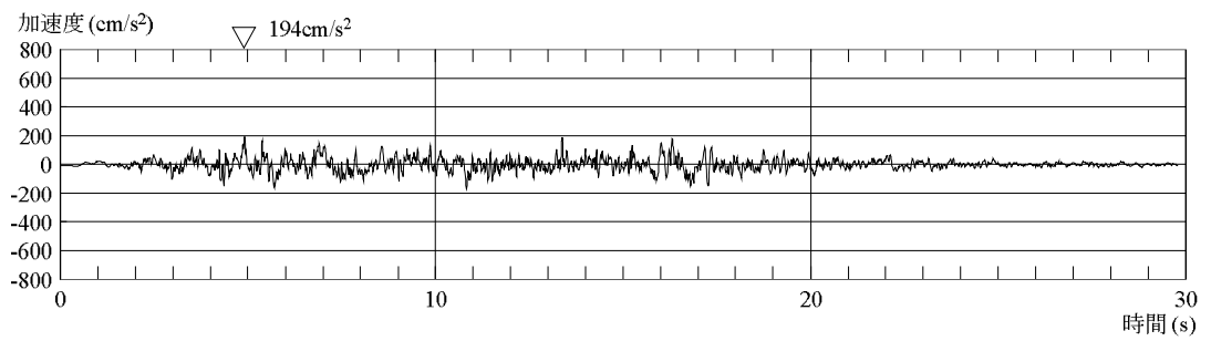
加速度(鉛直方向:Sd-1V)
