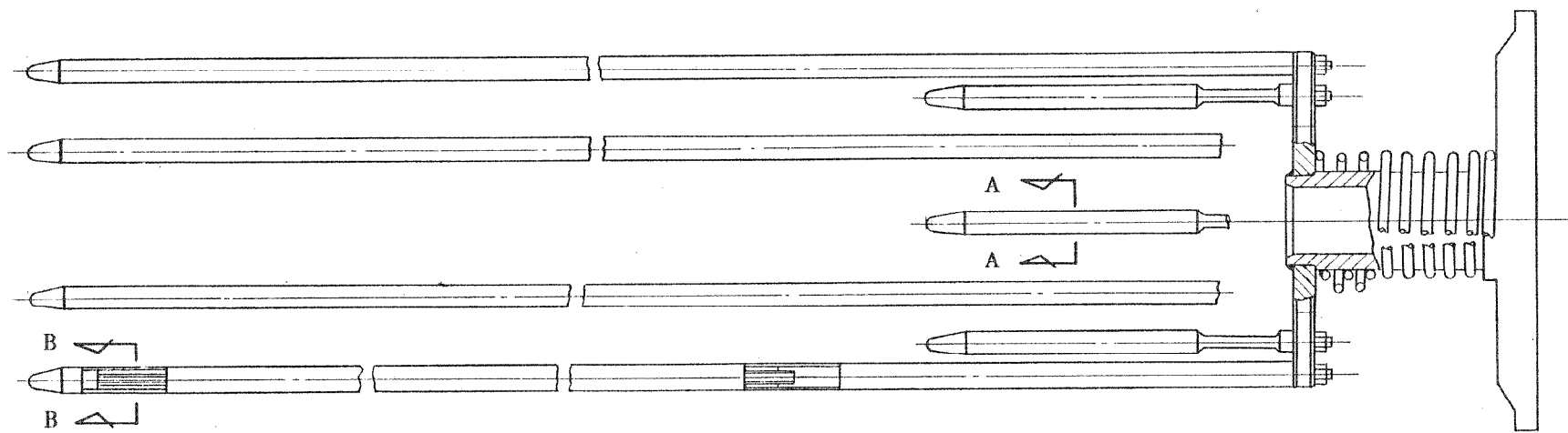
第1.4-25図 パーナブルポイズン構造説明図
