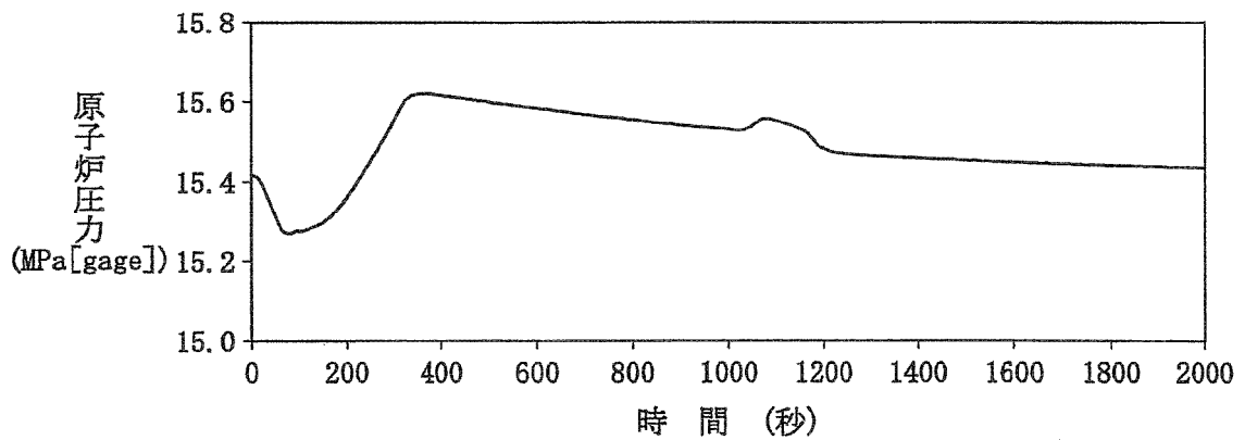
第1.4-19図 5%/minランプ状負荷増加の場合 (15%→100%)
