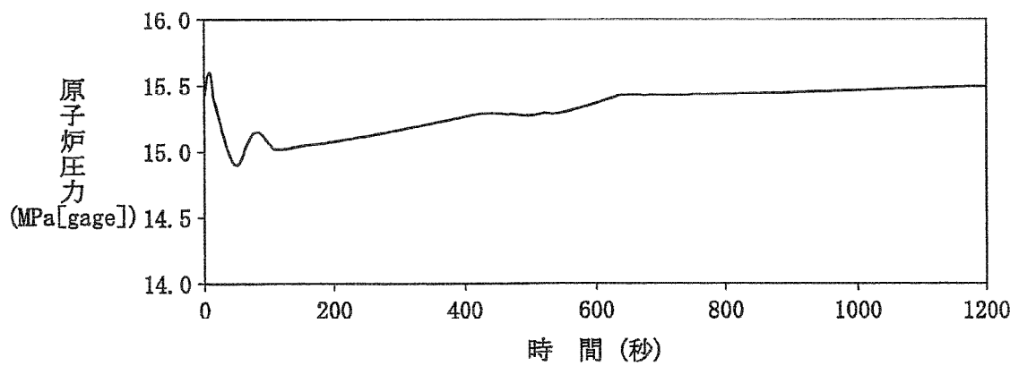
第1.4-21図 50%ステップ状負荷減少の場合(100%→50%)
