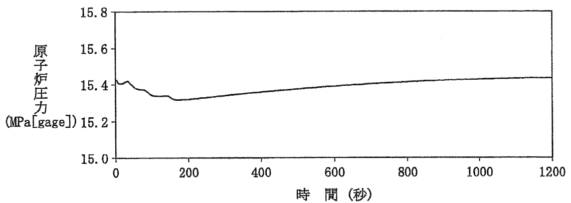
第1.4-17図 10%ステップ状負荷減少の場合(100%→90%)
