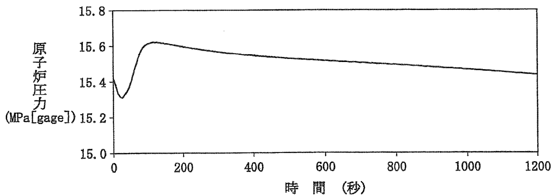
第1.4-18図 10%ステップ状負荷増加の場合(90%→100%)
