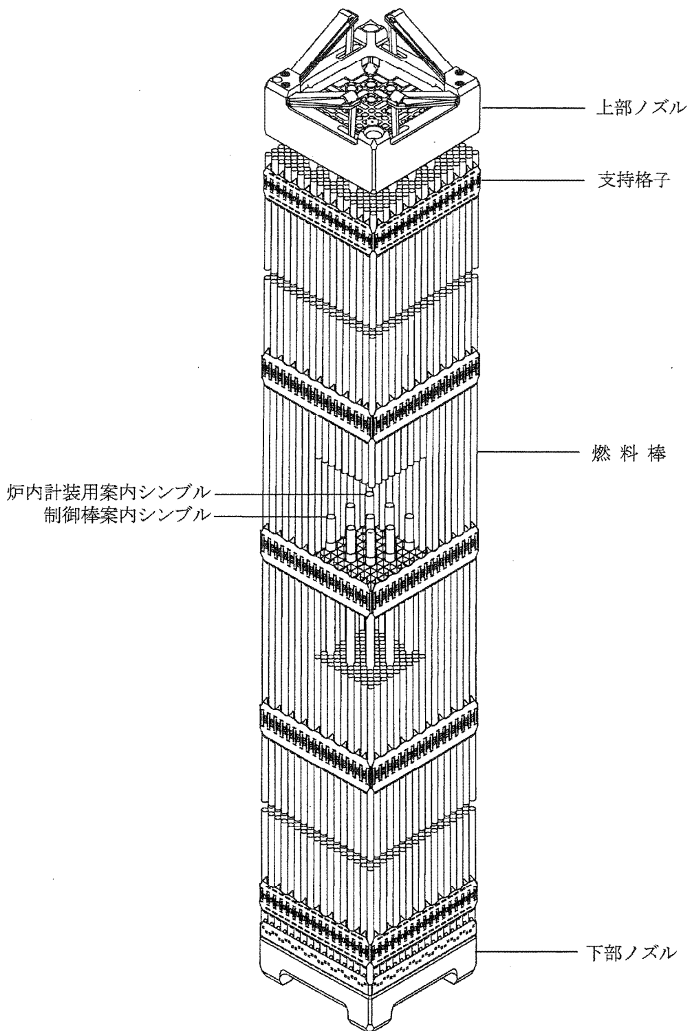
第1.4-5図 燃料集合体構造概要図
