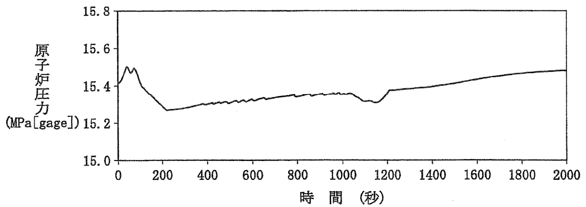
第1.4-20図 5%/minランプ状負荷減少の場合 (100%→15%)
