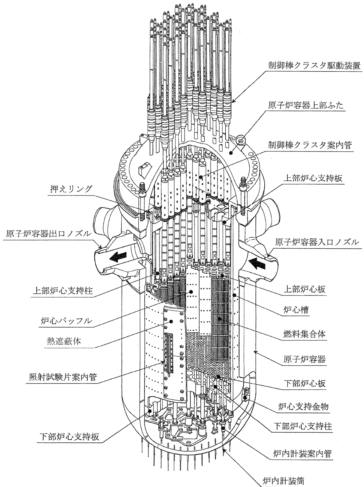
第1.4-1図 原子炉容器内構造説明図
