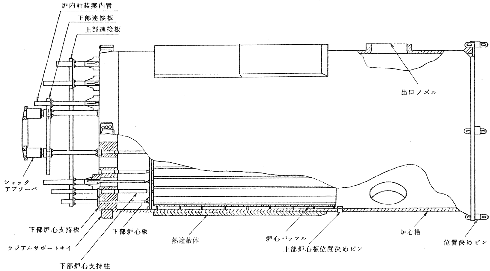
第1.4-32図 下部炉心構造物構造説明図
