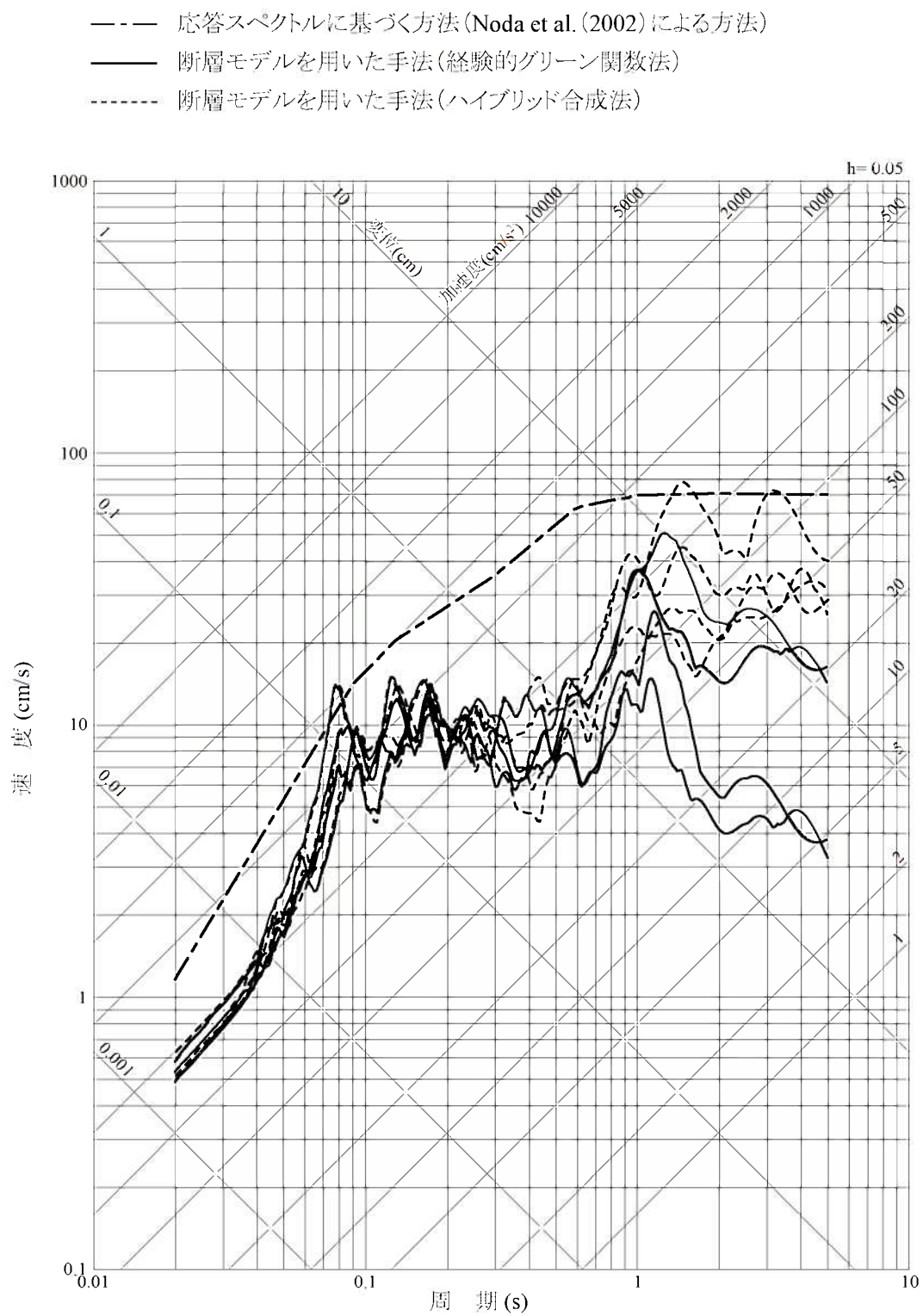
第1.2-282図 断層帯断層区間による地震の不確かさを考慮した地震動の応答スペクトル(断層傾斜角の不確かさを考慮したケース:水平方向)
