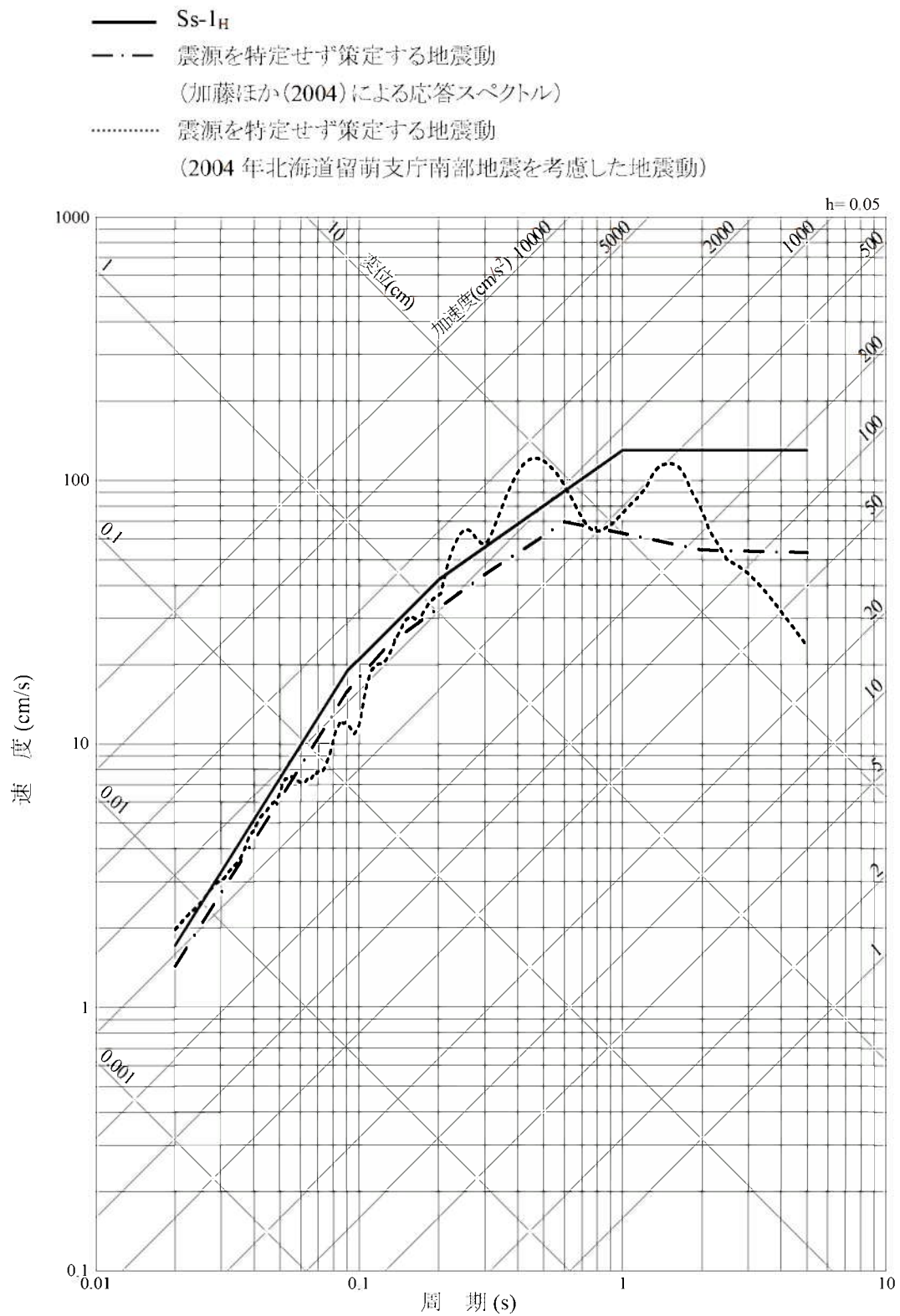
第1.2-309図 基準地震動Ss-Iの設計用応答スペクトルと「震源を特定せず策定する地震動」の応答スペクトル(水平方向)
