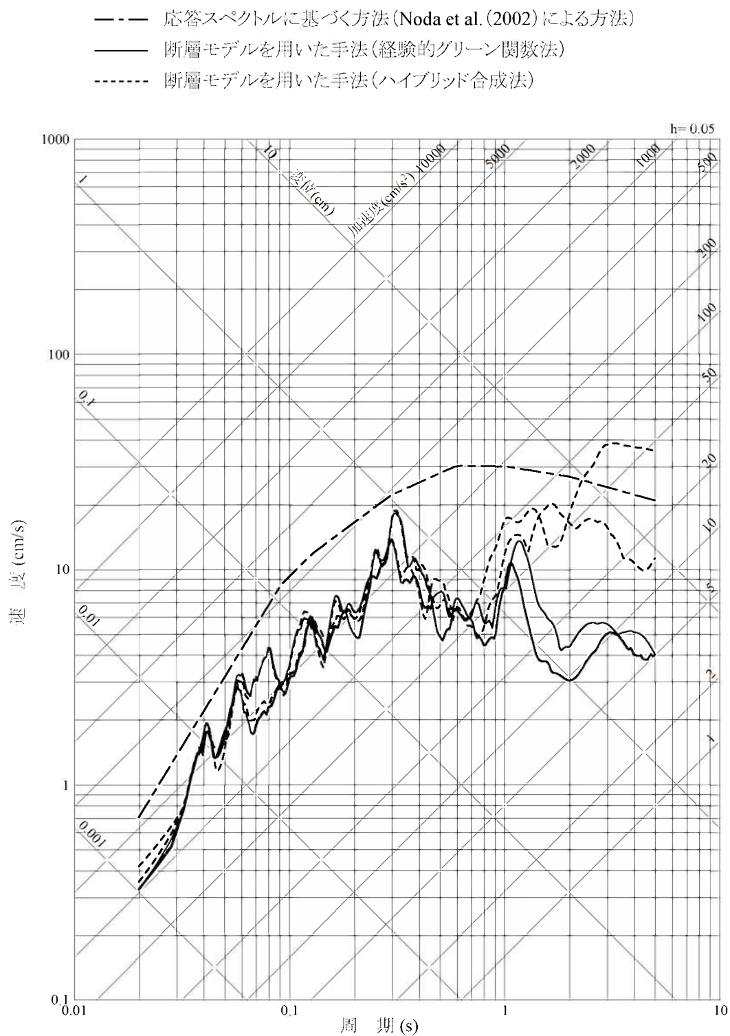
第1.2-283図 断層帯断層区間による地震の不確かさを考慮した地震動の応答スペクトル (断層傾斜角の不確かさを考慮したケース: 鉛直方向)
