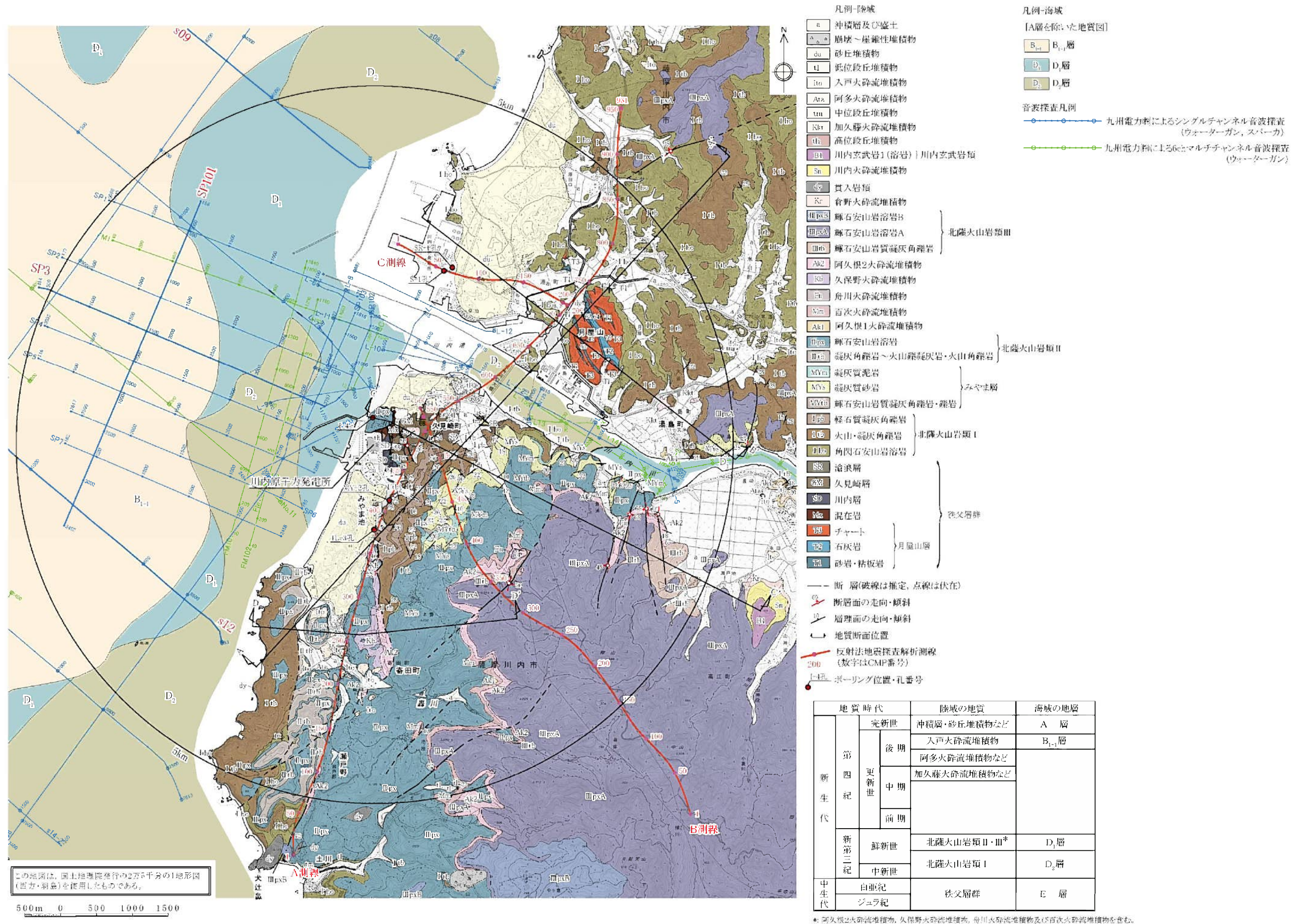
第1.2-182図 敷地近傍の地質図
