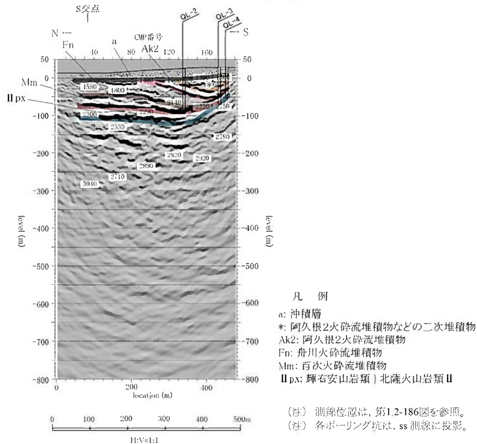
第1.2-194図(4) 反射法地震探査による深度断面とその解釈(ss測線)
