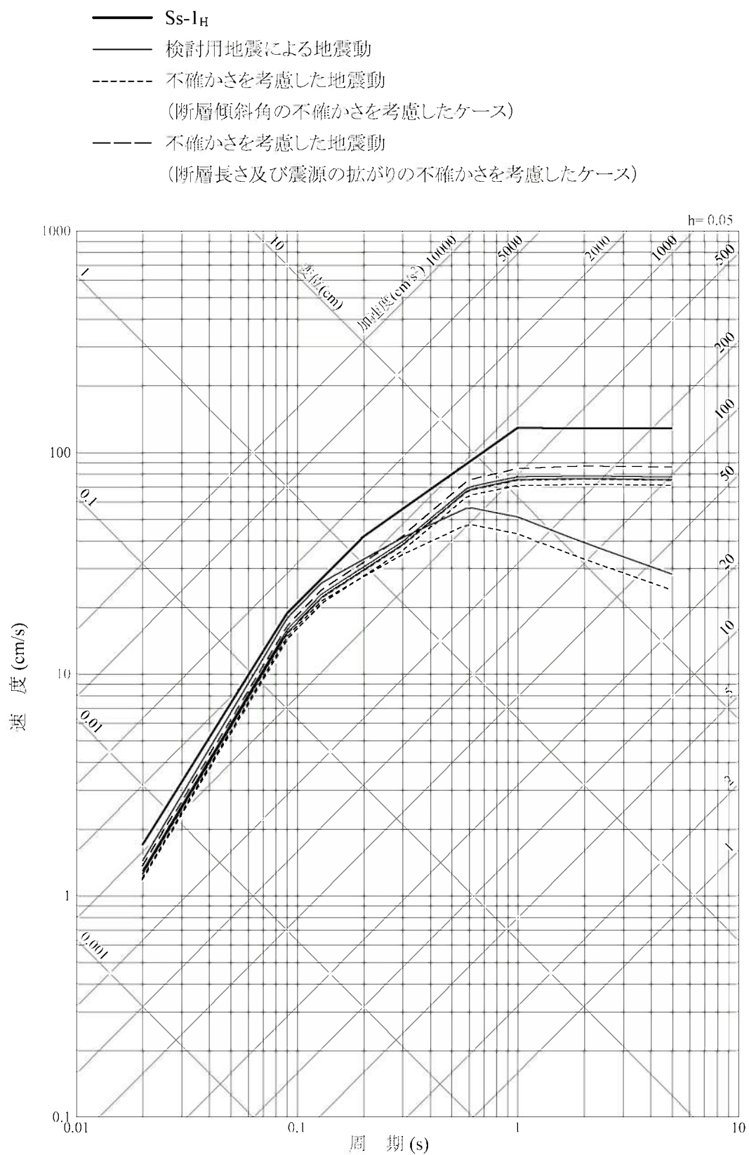
第1.2-302図 基準地震動 S_s-I の設計用応答スペクトル及び検討用地震の 応答スペクトル(応答スペクトルに基づく方法:水平方向)
