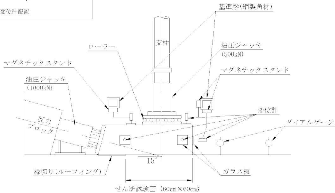
第1.2-214図(2) ブロックせん断試験装置概略図(ST-2及びST-4)
