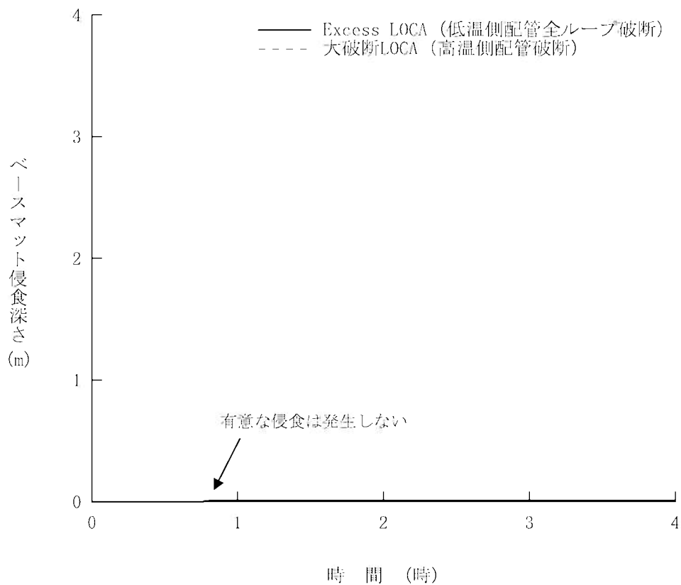
第1.15-426図 ベースマット侵食深さの推移 (低温側配管全ループ破断時の影響確認)
