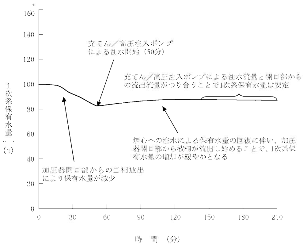
第1.15-342図 1次系保有水量の推移
