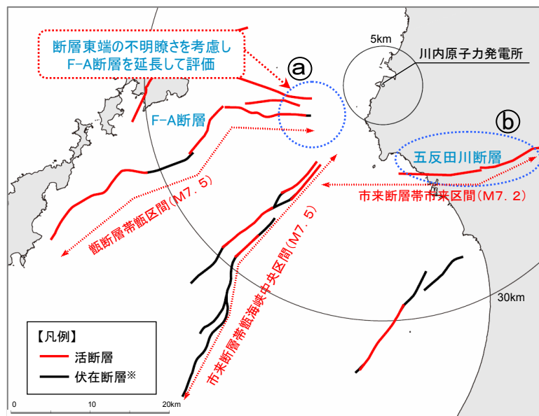
〔発電所周辺の活断層分布〕
