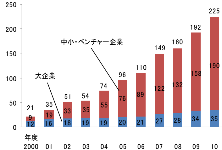
福岡県内先端半導体開発(システムLSI設計)関連の企業集積の推移
