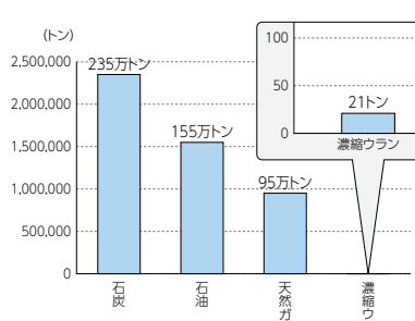
■100万kWの発電所を1年間運転するために必要な燃料
