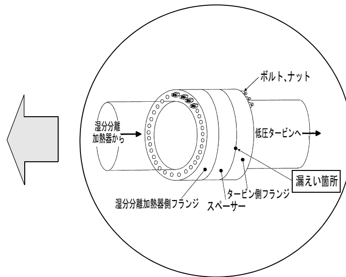
漏えい箇所(フランジ部)
