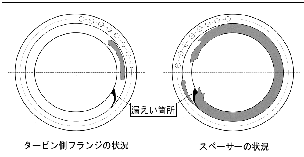
当該フランジ部パッキンの状況
