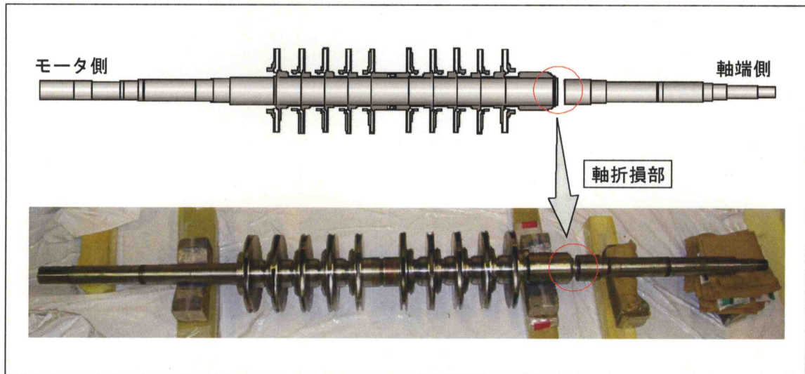
軸全体の構造図及び状況写真
