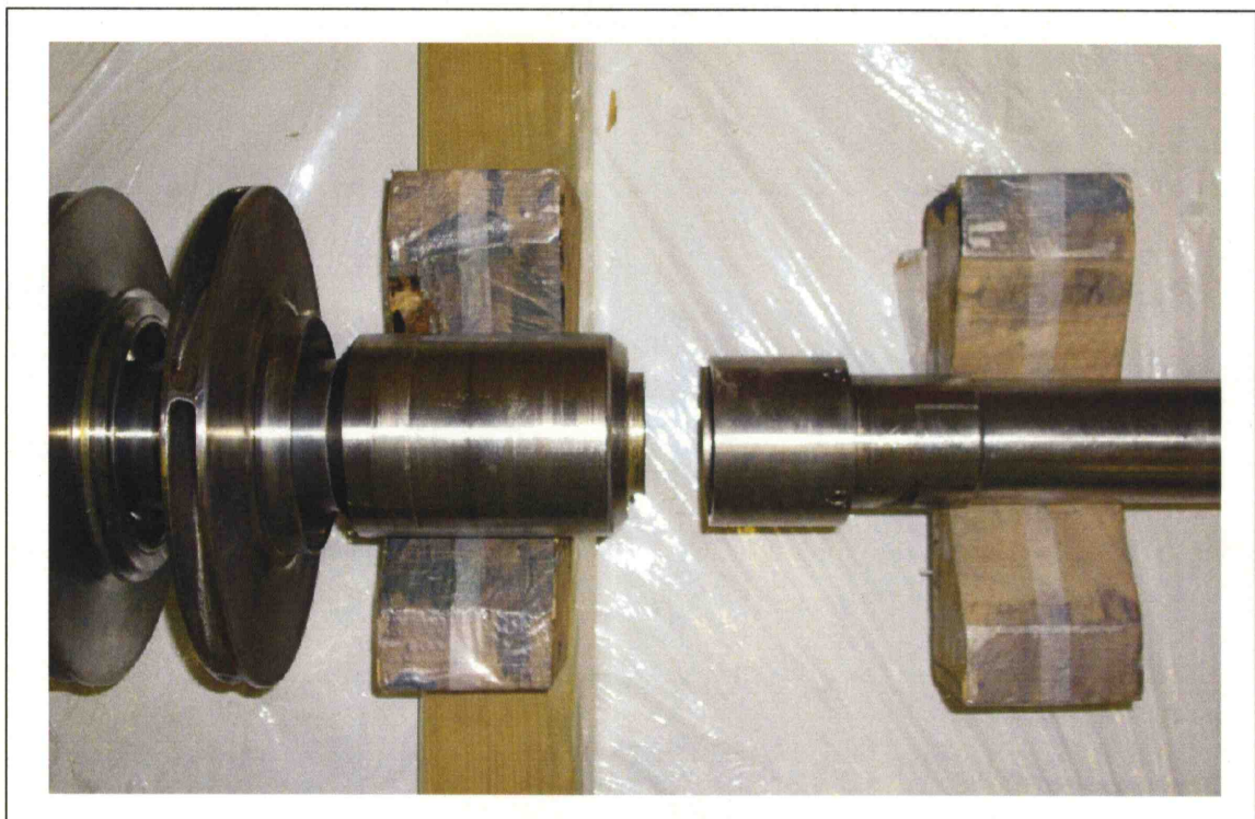
軸折損部の状況写真
