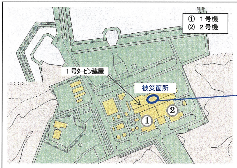
川内原子力発電所 配置図
