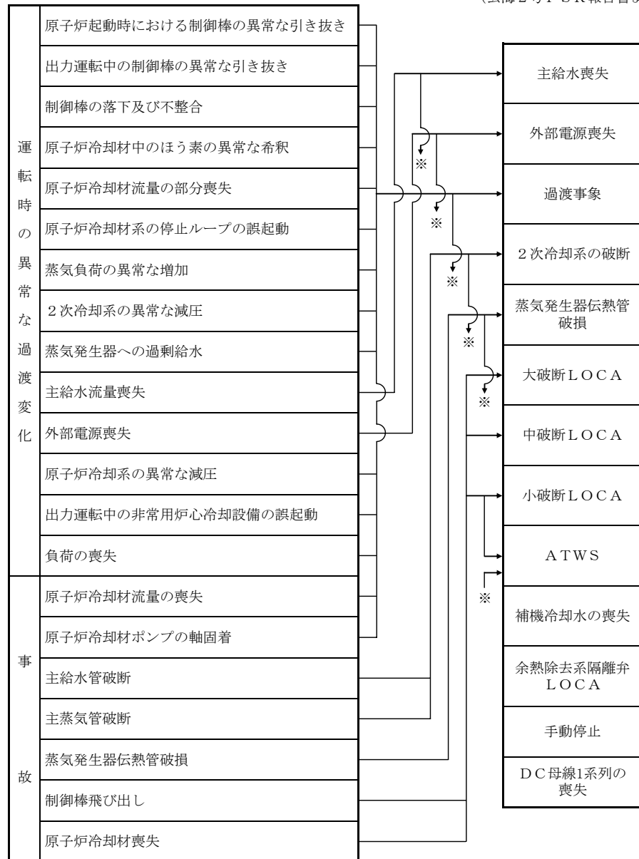
図5-6-1 安全評価審査指針と内的事象P S Aの関連性
