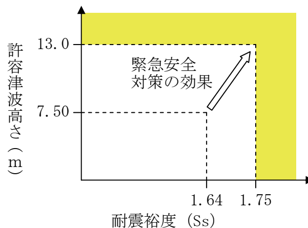
図5-3-3 地震と津波の重畳に関するクリフェッジ評価結果 (炉心：緊急安全対策整備前後の比較)
