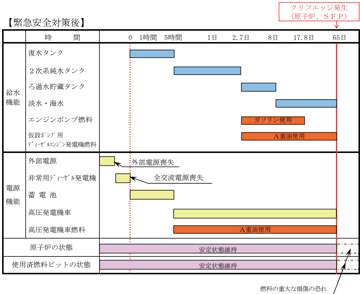
図 5-4-6 プラント運転時における事象の過程の進展を防止する措置の効果の評価結果
