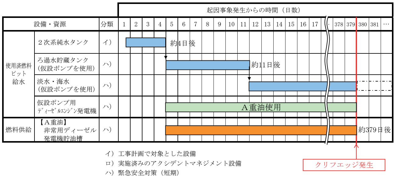
図5-5-4 プラント停止時の給水機能継続時間評価 及びクリフエッジ所在の特定結果
