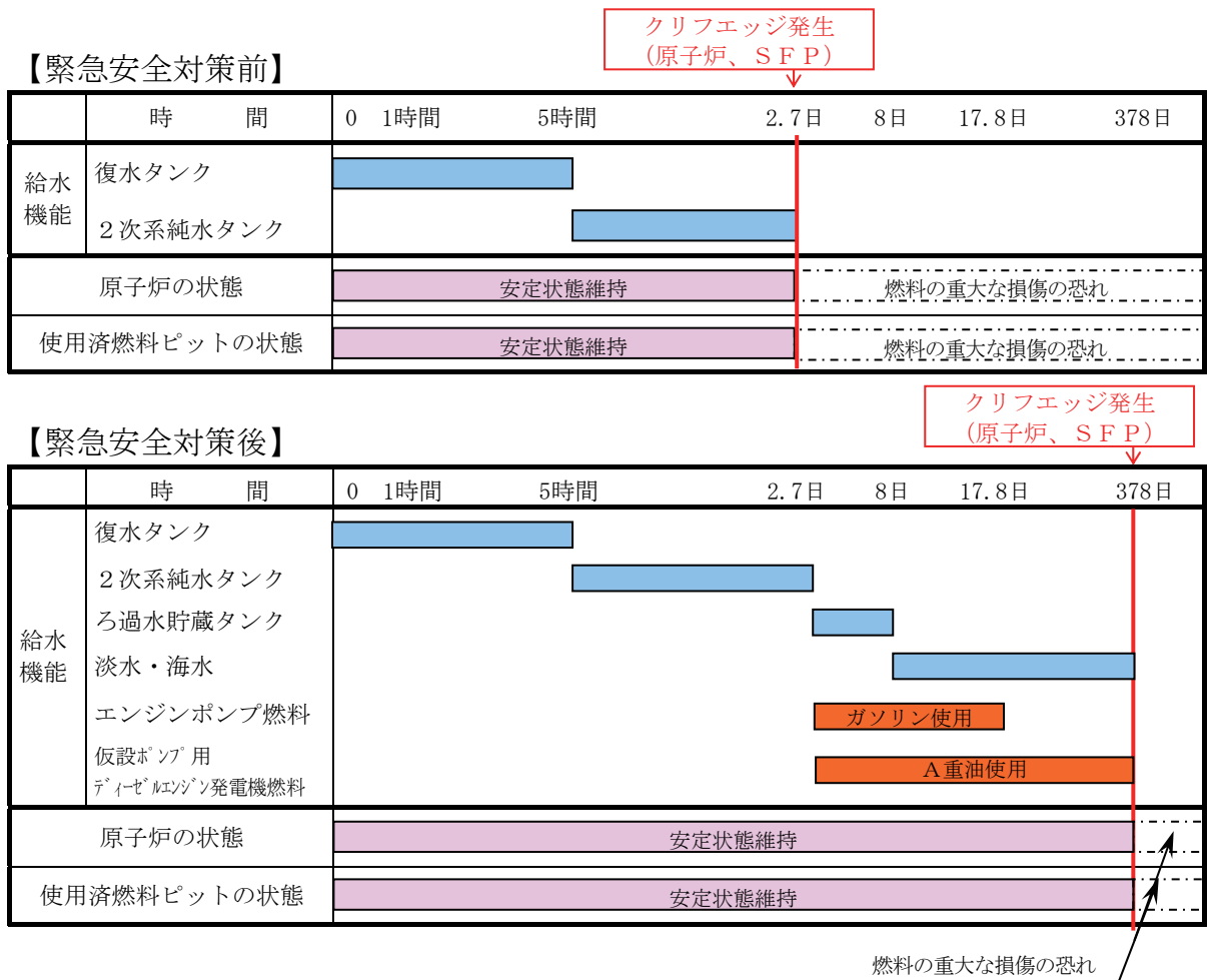
図5-5-5 プラント運転時における事象の過程の進展を防止する措置の効果の評価結果
