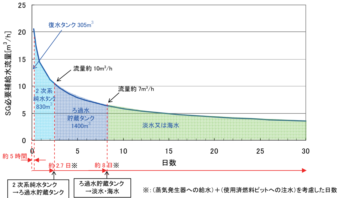
図 2 蒸気発生器 (SG) への必要補給水流量
