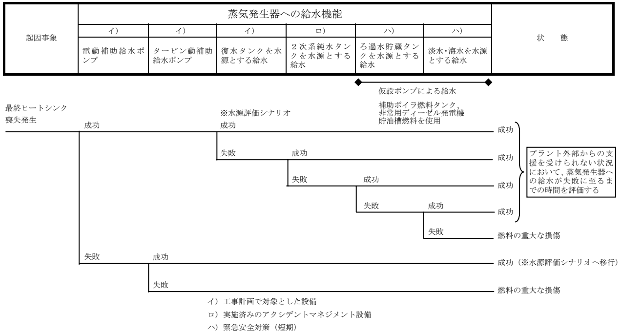
図 5-5-1 最終ヒートシンク喪失から燃料の重大な損傷に至る事象の過程(原子炉)
