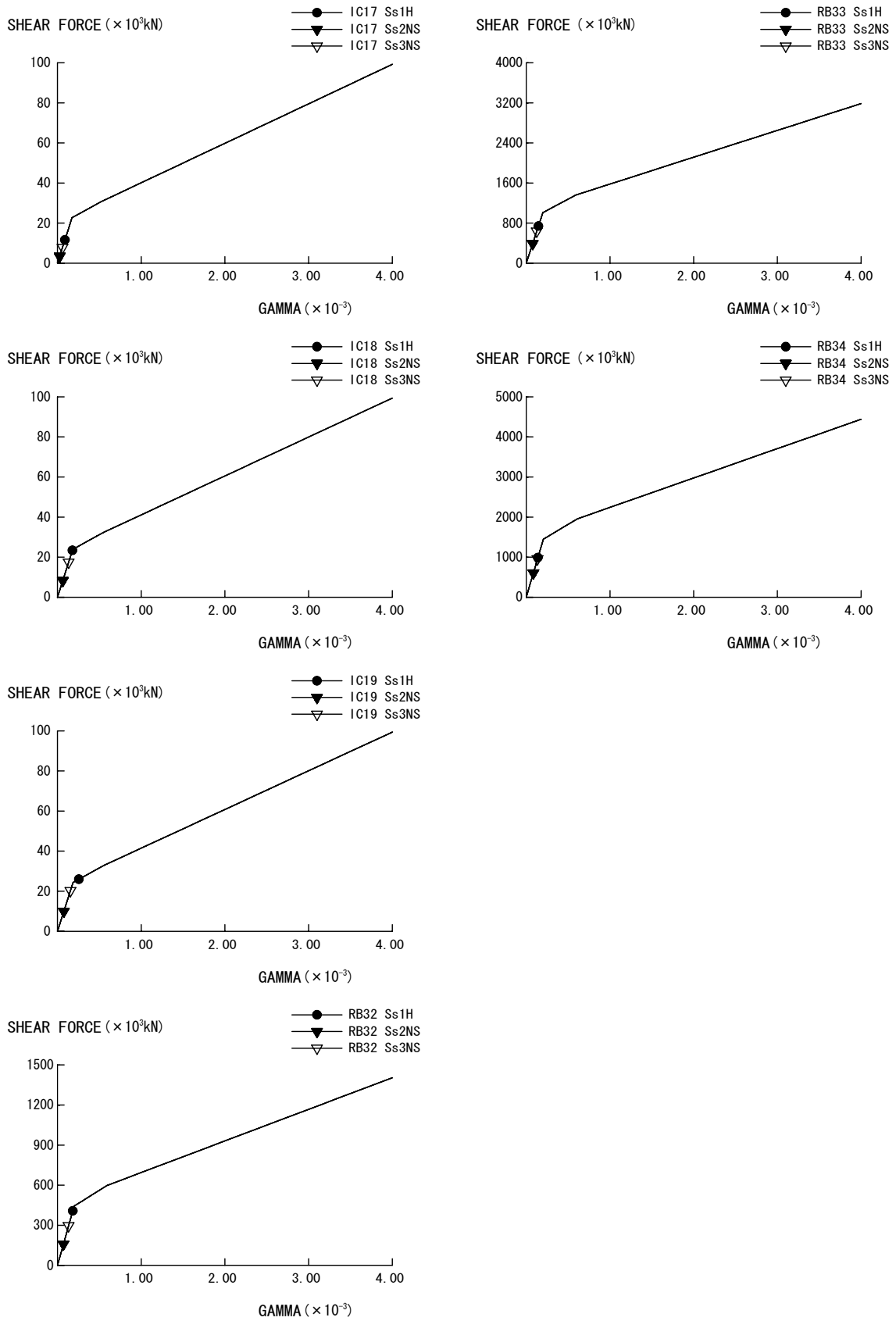
図 2 - 3 - 3 Q- \gamma 関係と最大応答値 (原子炉建屋 IC REB NS 方向)
