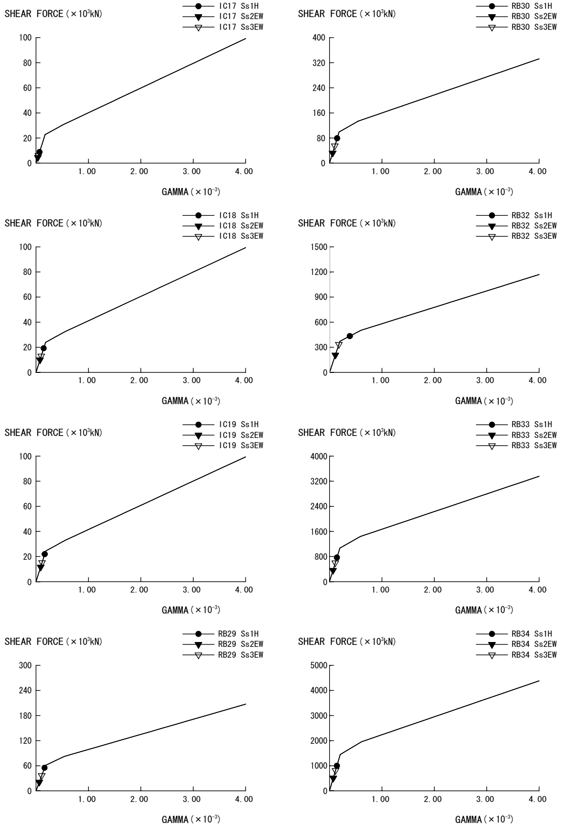
図 2-3-6 Q- \gamma 関係と最大応答値 (原子炉建屋 IC REB EW 方向)
