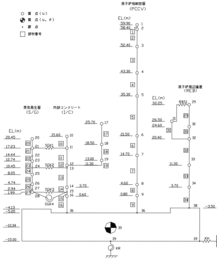
図 2-1 原子炉建屋の解析モデル (水平)
