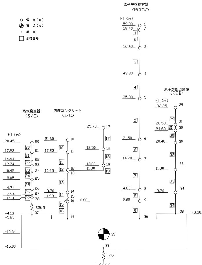
図 2-2 原子炉建屋の解析モデル (鉛直)
