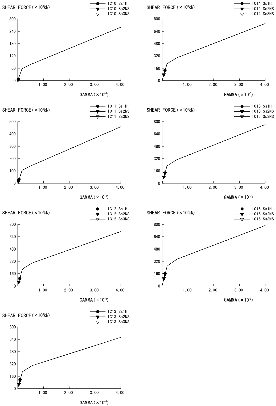
図 2-3-2 Q- \gamma 関係と最大応答値 (原子炉建屋 IC NS 方向)
