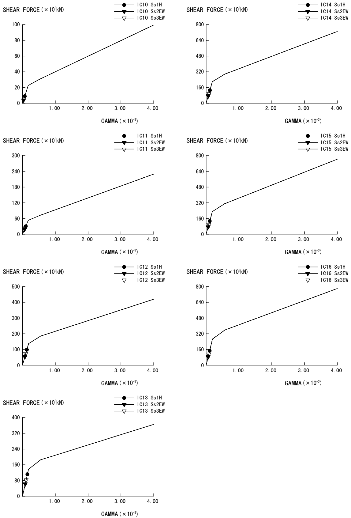
図 2-3-5 Q- \gamma 関係と最大応答値 (原子炉建屋 IC EW 方向)
