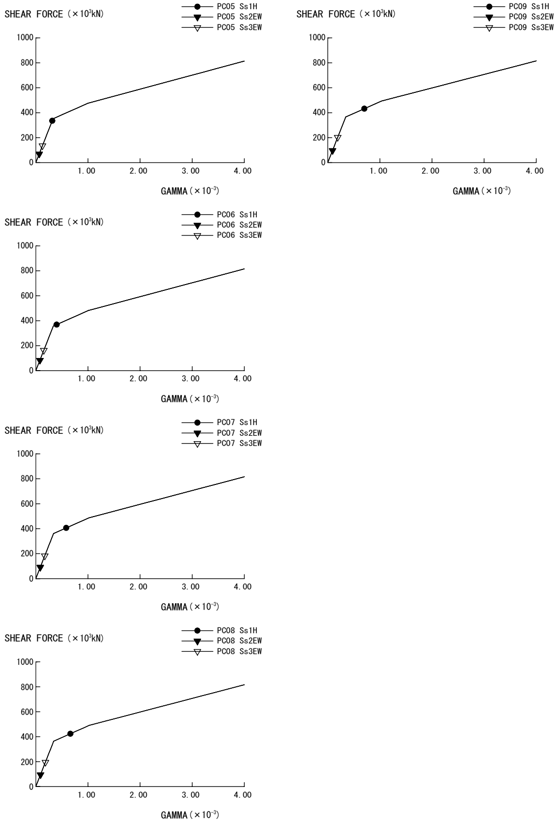
図 2-3-4 Q- \gamma 関係と最大応答値 (原子炉建屋 PCCV EW 方向)
