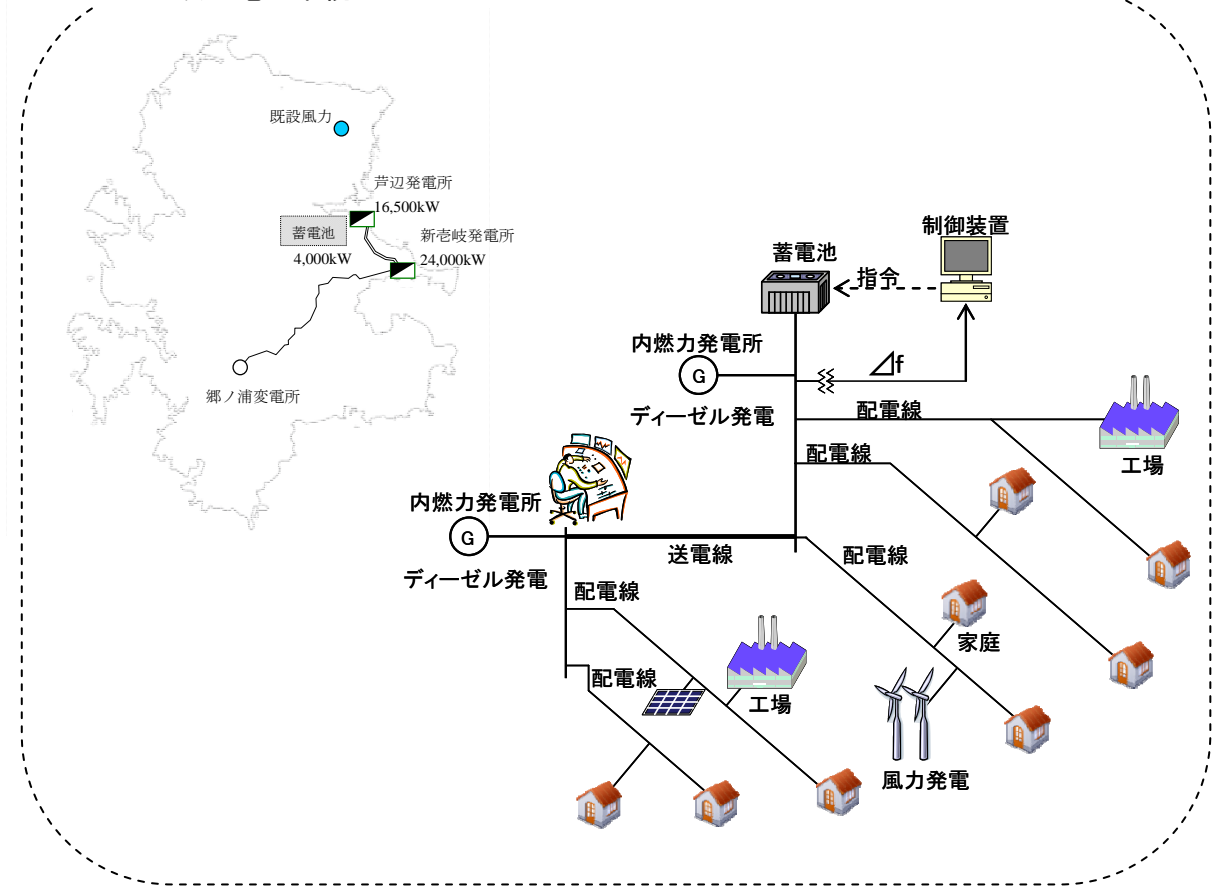
壱岐の電力系統イメージ
