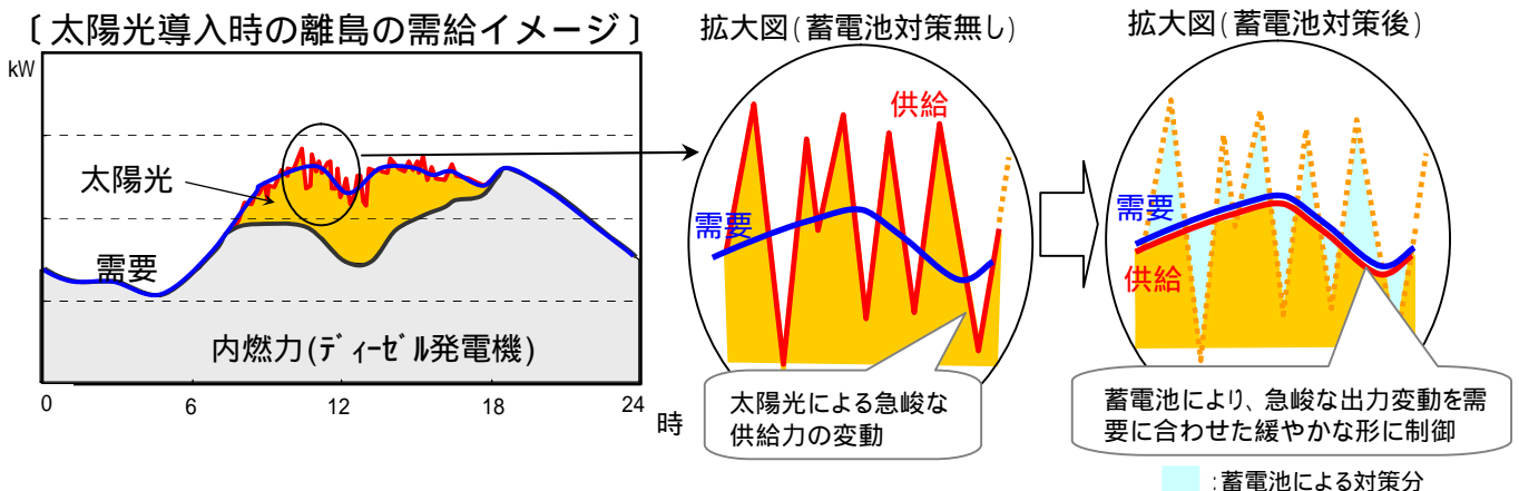
( 図 2 ) 蓄電池による太陽光出力変動抑制のイメージ
