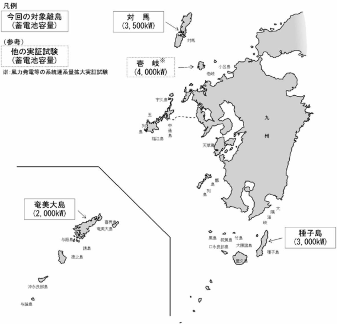
( 図 1 ) 蓄電池の設置場所と蓄電池容量
