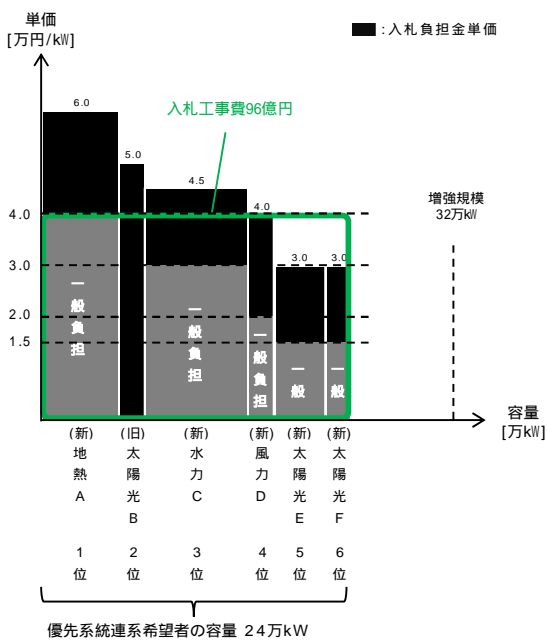
〔 入札対象工事（220kV XY線増強工事） 〕
