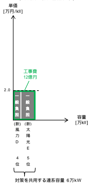
〔 その他供給設備工事（Y変電所1号変圧器増強工事） 〕
