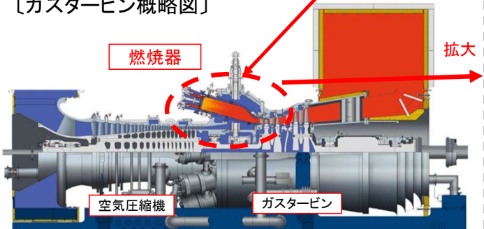
〔ガスタービン概略図〕
