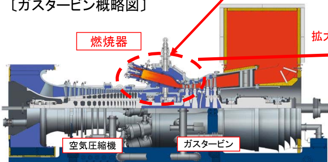
〔ガスタービン概略図〕
