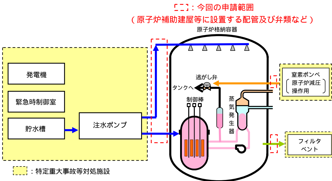
特定重大事故等対処施設の概要図
