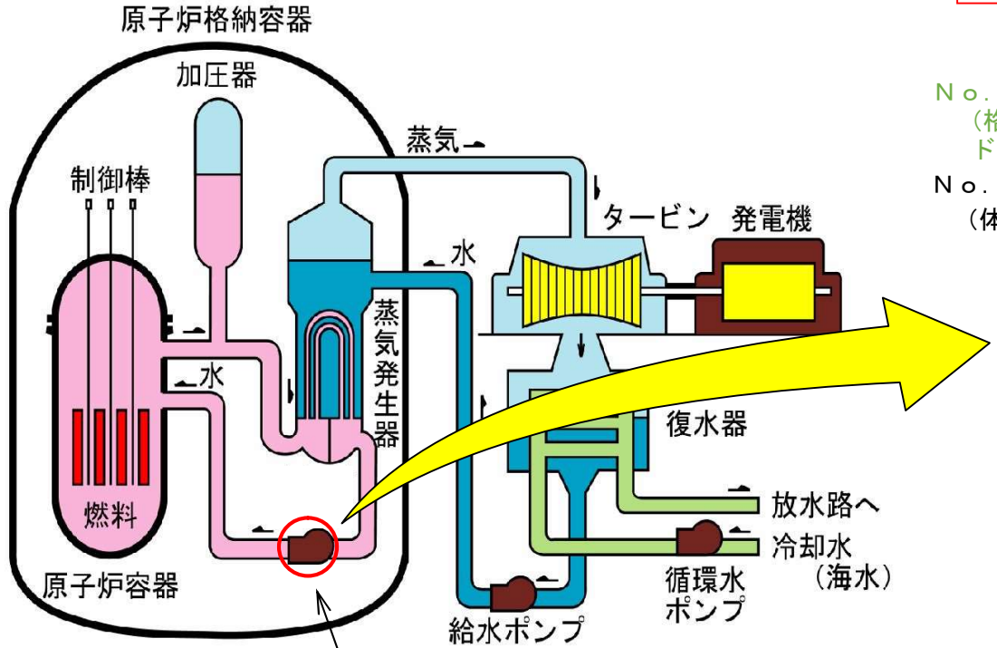
1次冷却材ポンプ (4台) 発電所の系統概略図
