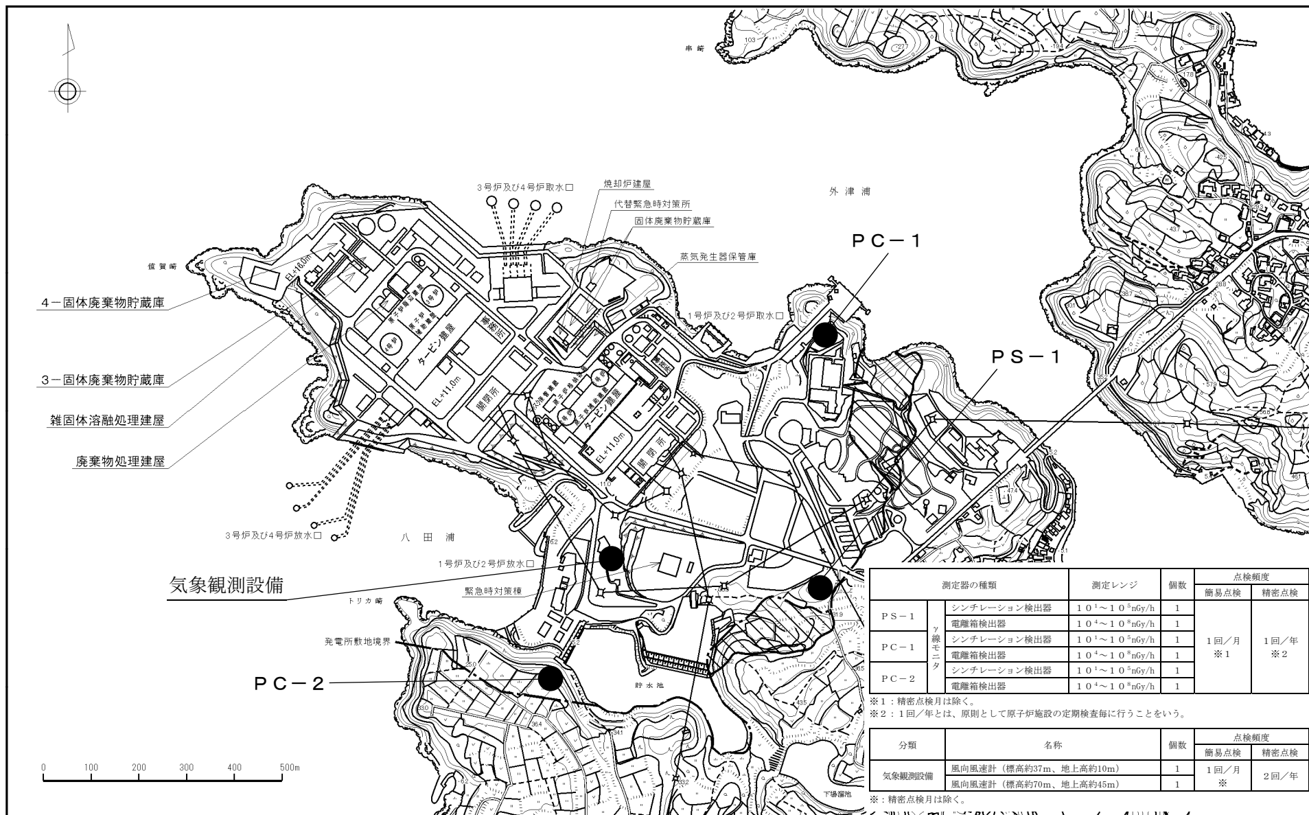
別図3-2 発電所敷地境界付近の放射線測定設備等
