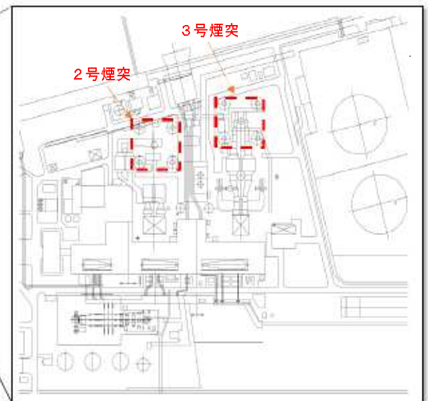
【旧唐津発電所構内配置図】
