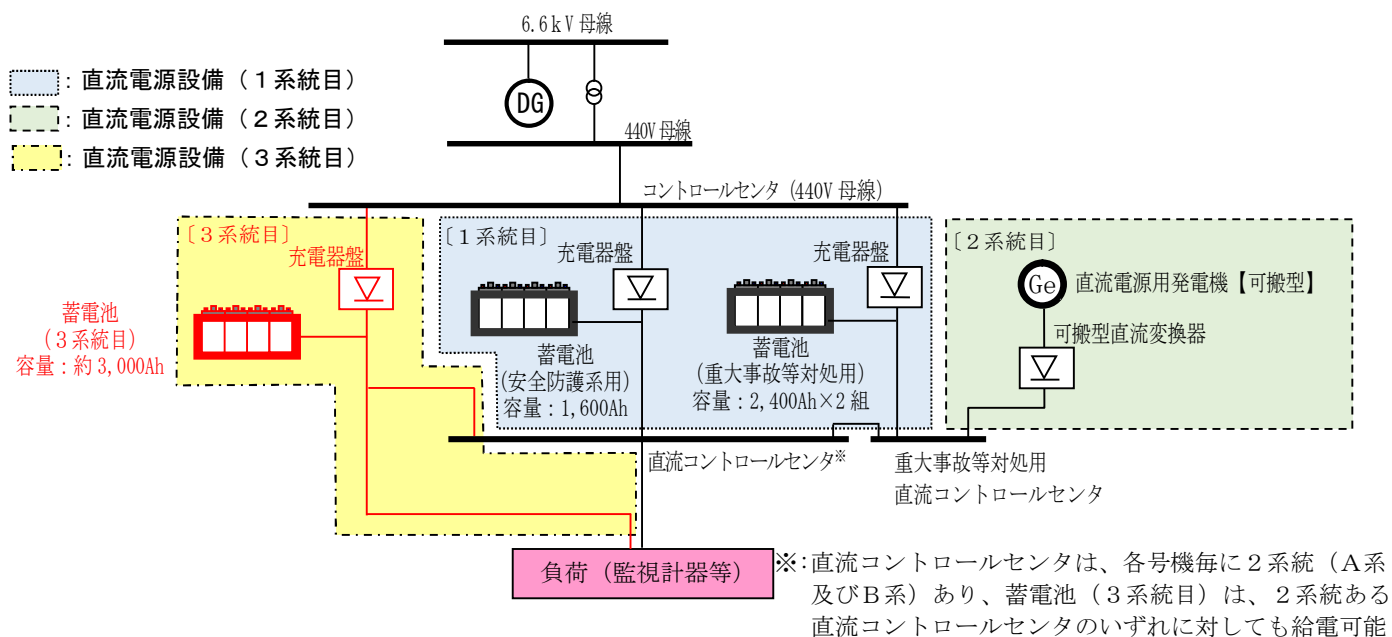
常設直流電源設備の概要図
