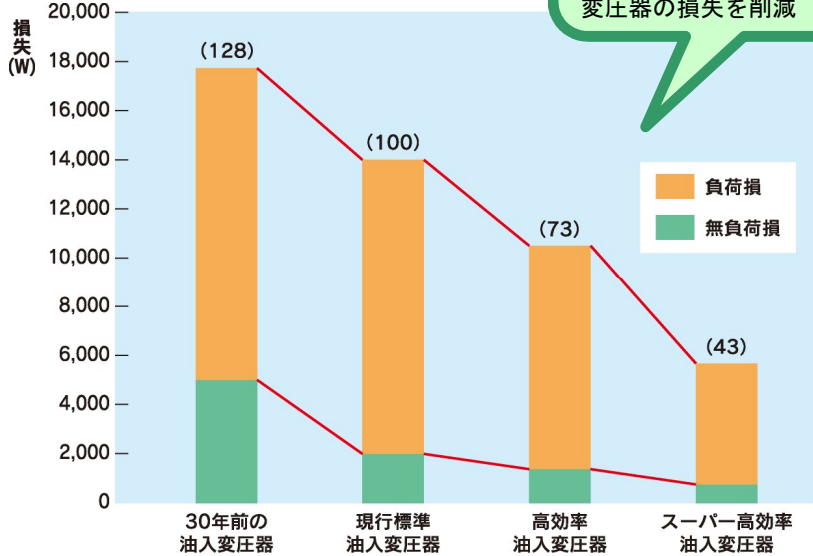
油入変圧器損失の比較
