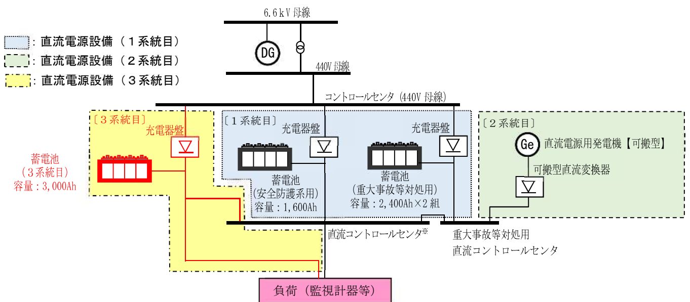
【直流電源設備の系統概要図】
