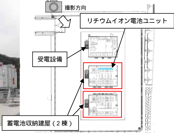
敷地平面図
