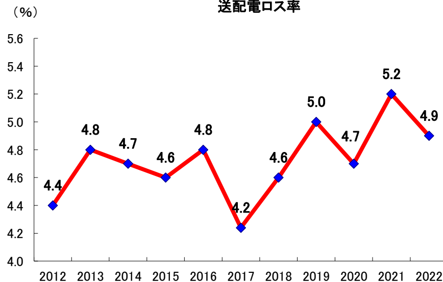
送配電ロス率
