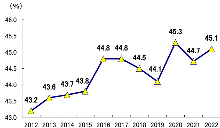
火力発電所熱効率(発電端)
