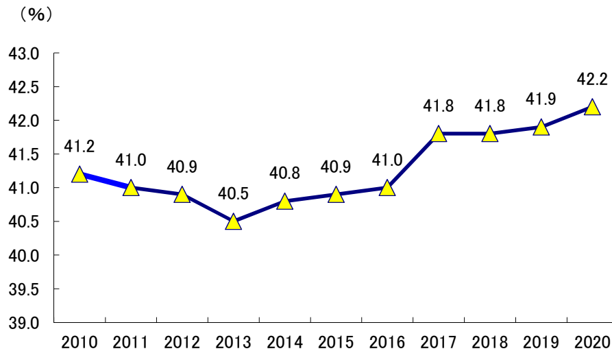
火力発電所熱効率(発電端)
