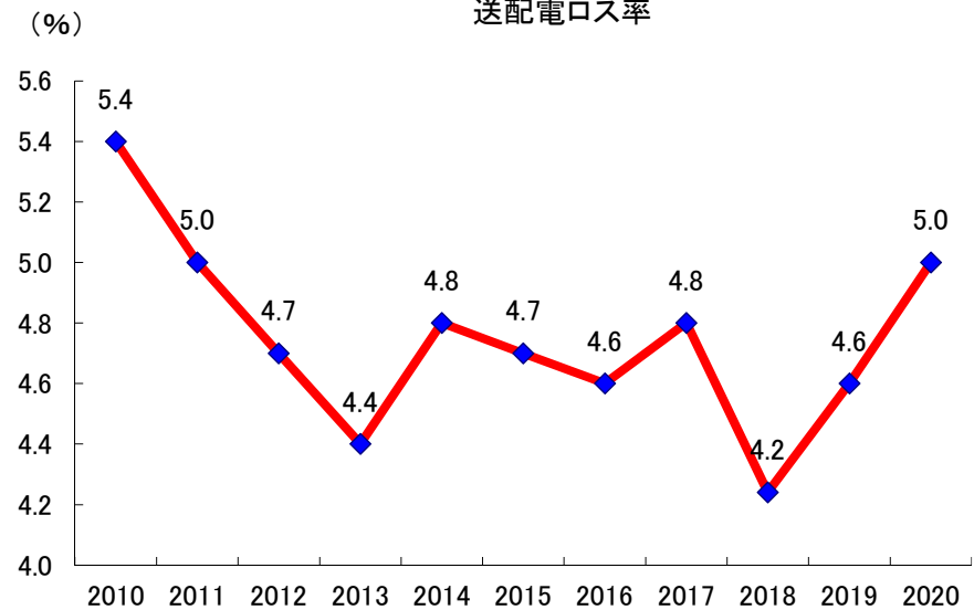
送配電ロス率
