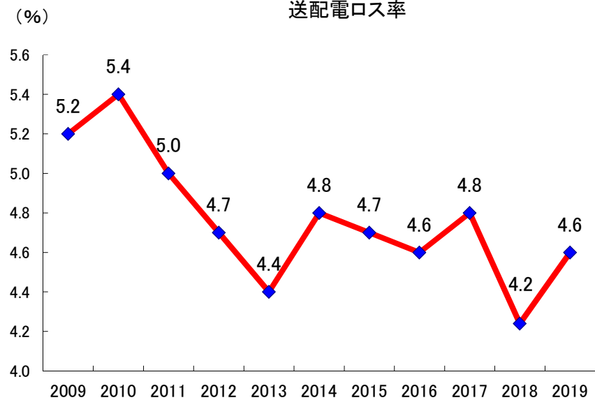
送配電ロス率
