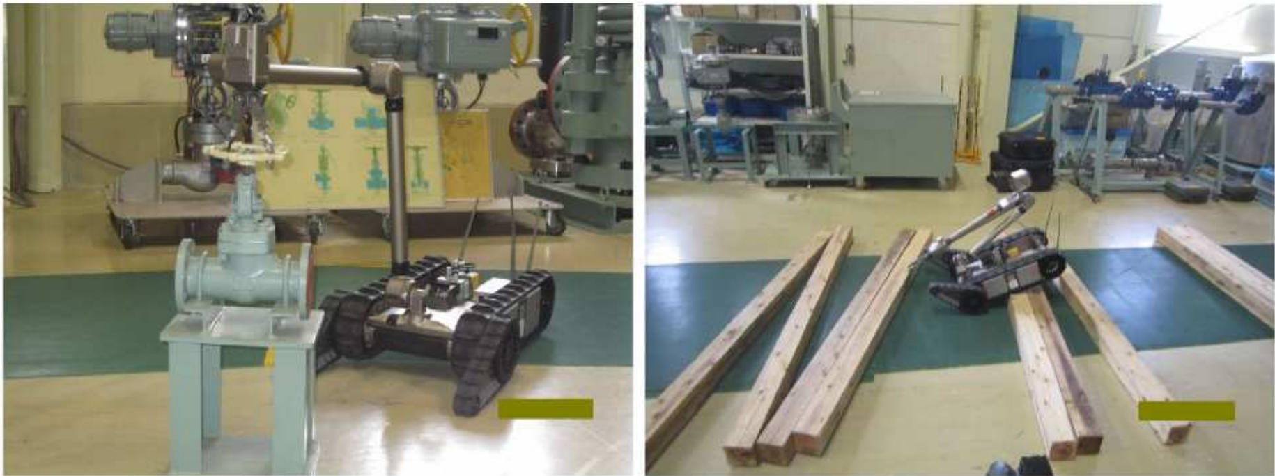
発電所におけるロボット操作の訓練状況
