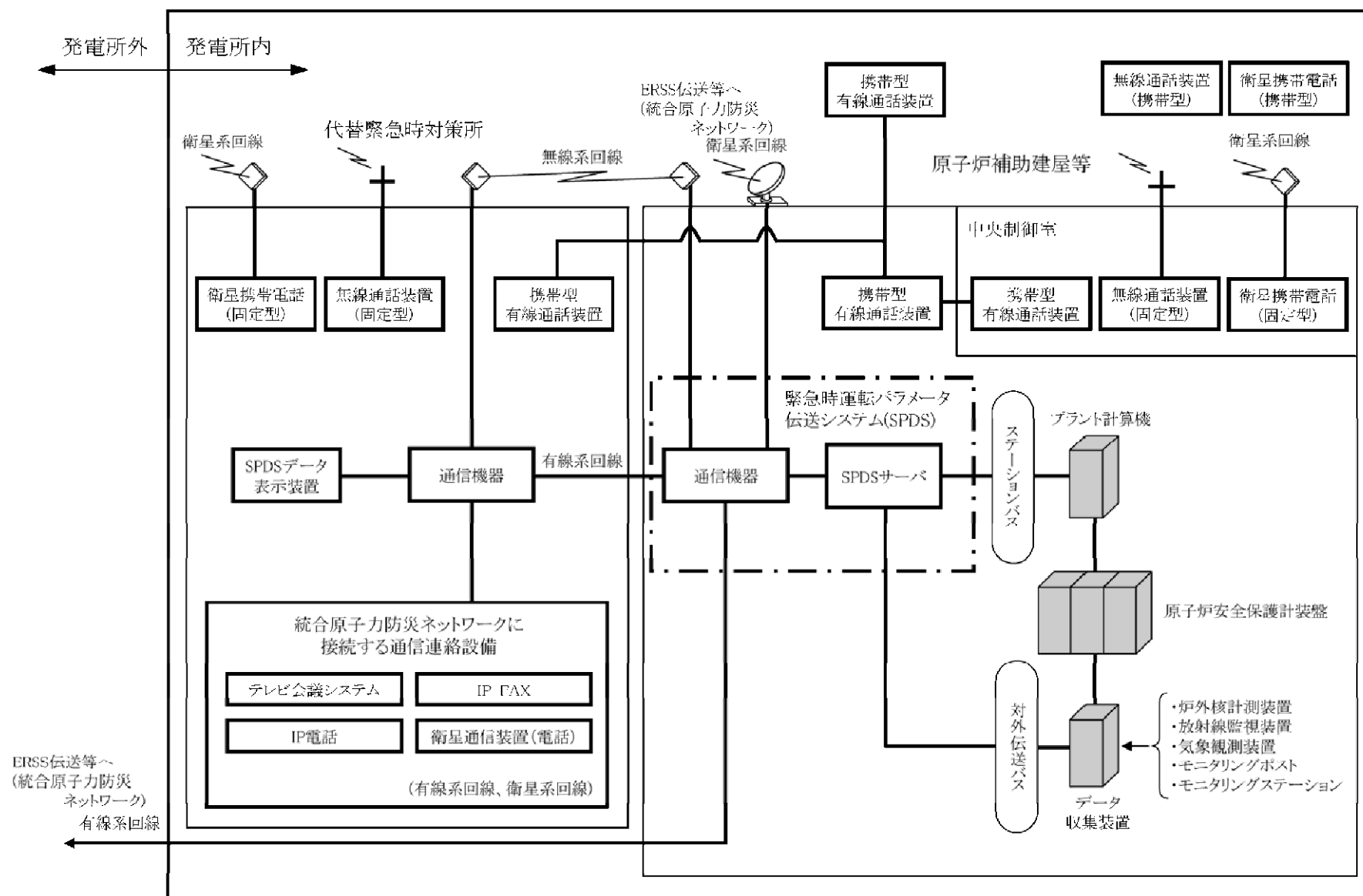
第1.7-27図 通信連絡設備 概略系統図(1)
