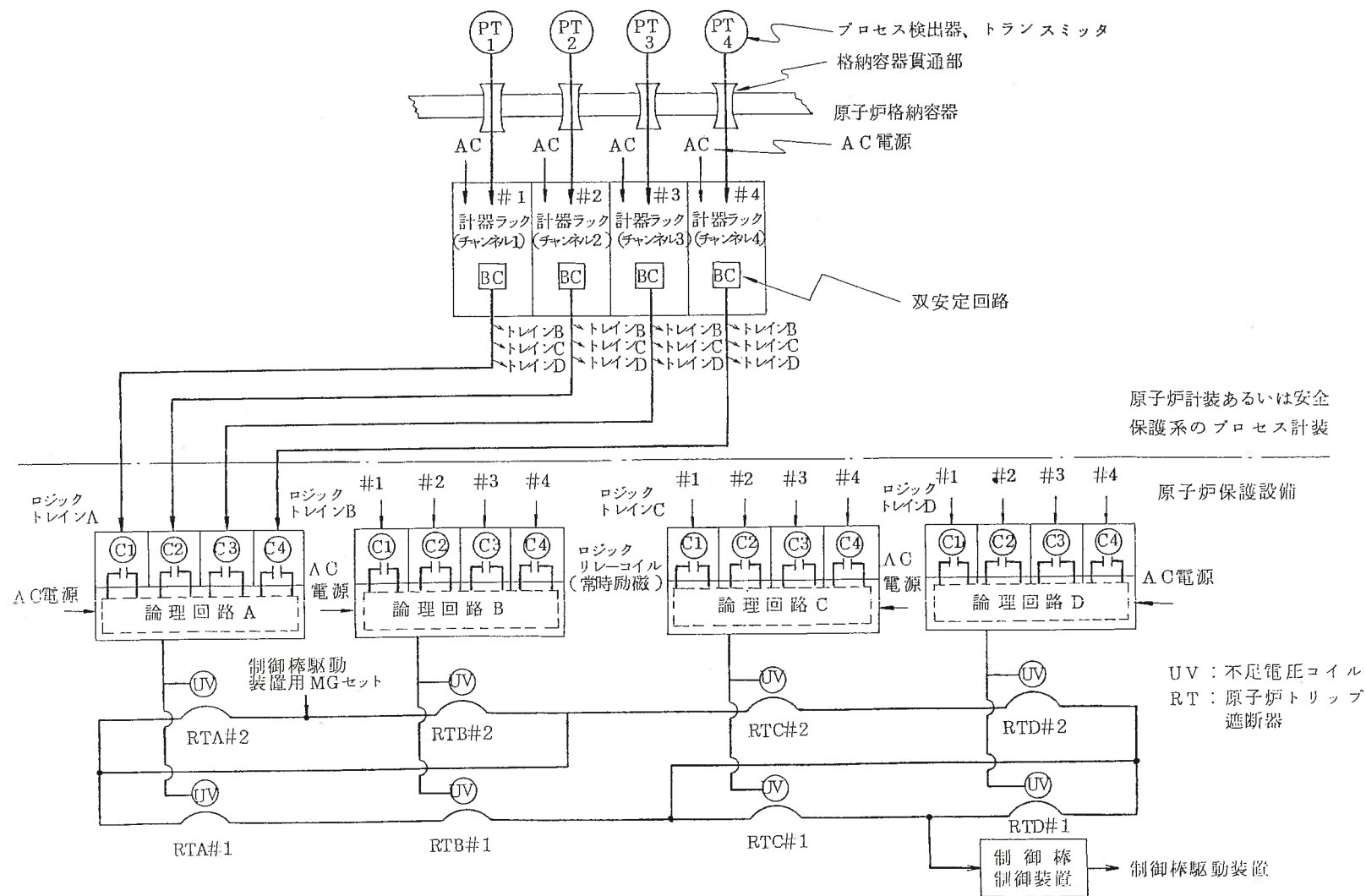
第1.7-7図 原子炉保護設備説明図 (2 out of 4の場合)
